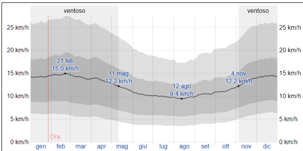
Figura 77: Media delle velocità del vento orarie medie (riga grigio scuro), con fasce del 25° - 75° e 10° - 90° percentile. (Fonte: MERRA-2 Modern-Era Retrospective Analysis_NASA)
