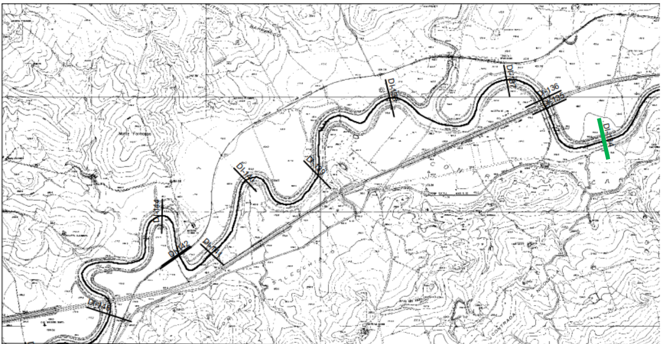
Figura 89: Schema planimetrico con l'ubicazione delle sezioni di calcolo per le verifiche idrauliche nel tratto del fiume Dittaino - In verde la sezione analizzata DI-134 - 8 Km a Nord dell'area di progetto
