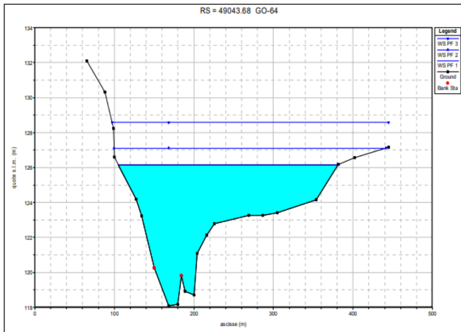
Figura 88: SEZIONE GO-64 "Appendice idraulica" del PAI - estratto piano di stralcio di bacino PAI 2005 (agg. 2008)
