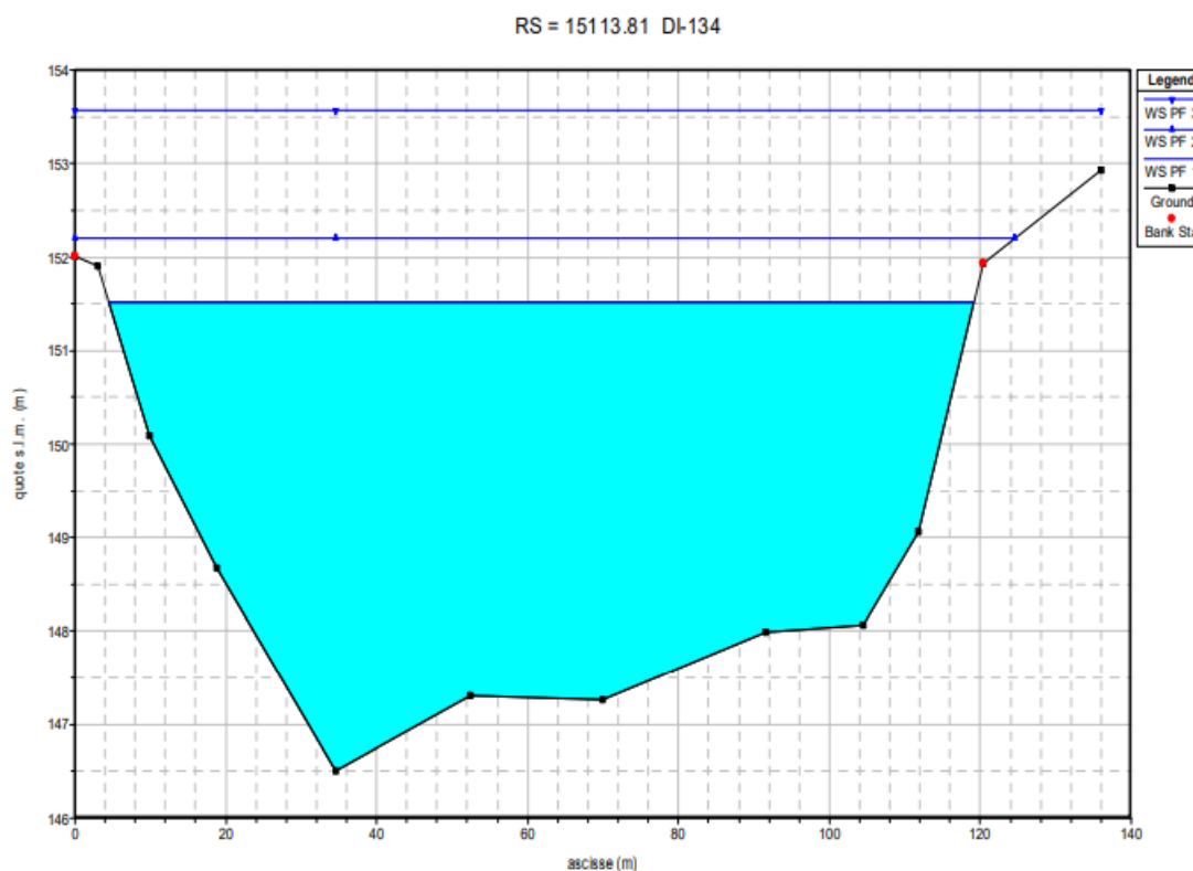
Figura 91: SEZIONE DI-134 "Appendice idraulica" del PAI - estratto piano di stralcio di bacino PAI 2005 (agg. 2008)
