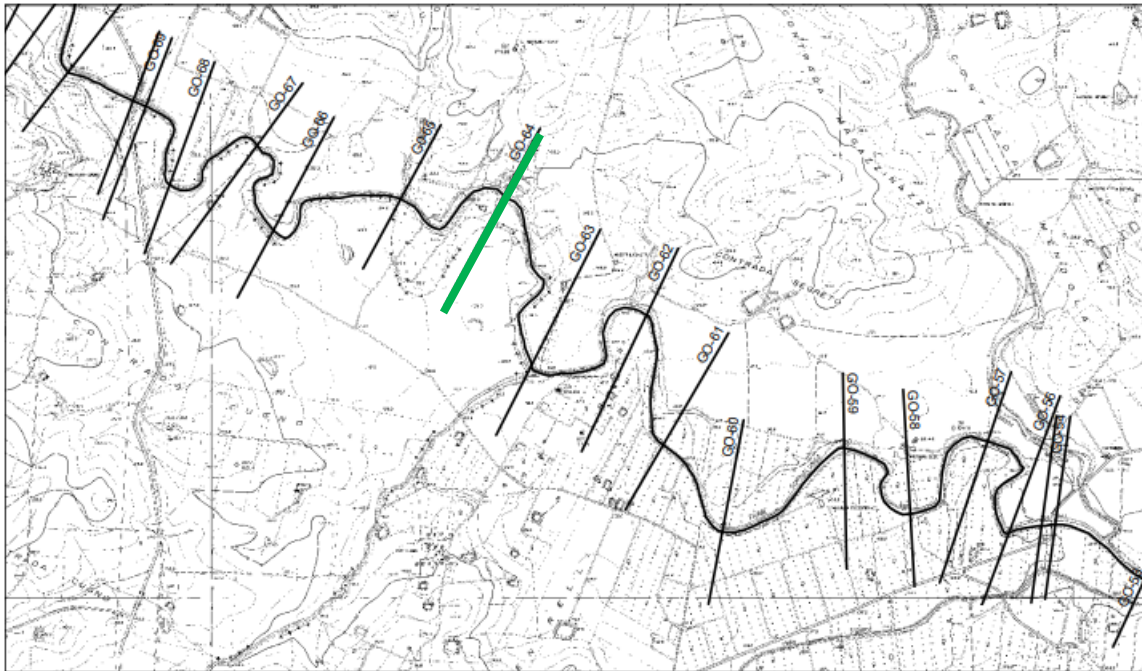
Figura 86: Schema planimetrico con l'ubicazione delle sezioni di calcolo per le verifiche idrauliche nel tratto del fiume Gornalunga - In verde la sezione analizzata GO-64
