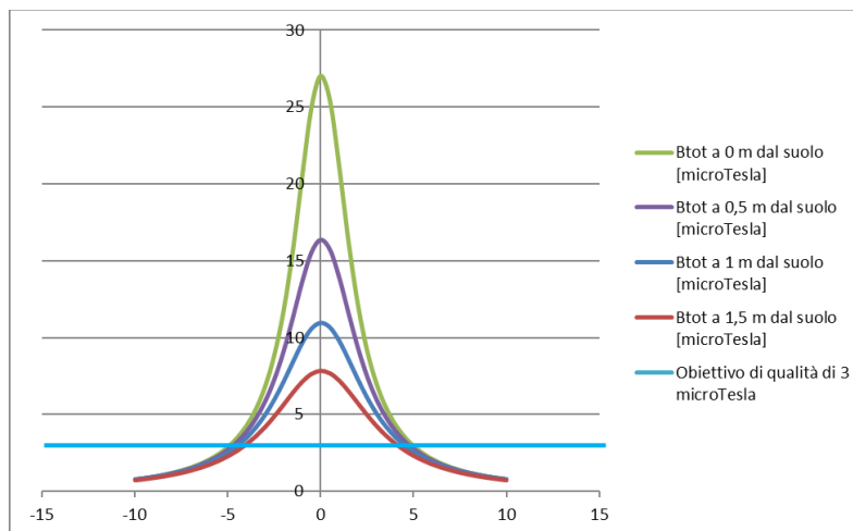
Andamento del campo magnetico generato dal cavidotto, composto da una terne da 1.600 mm 2
