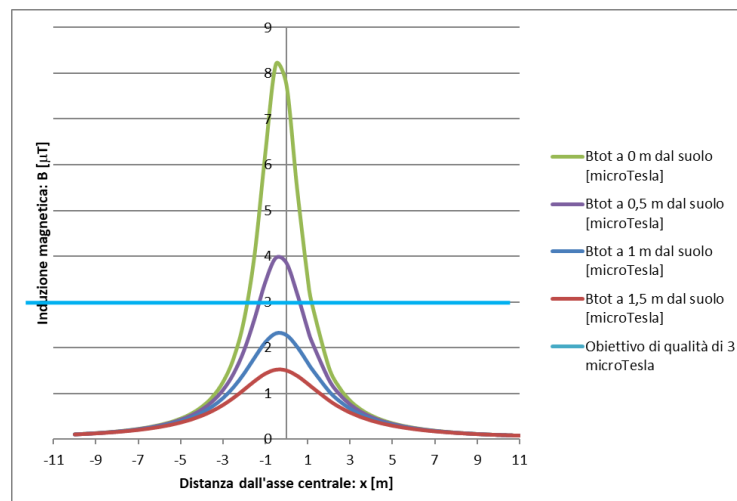
Figura 3: Andamento del campo magnetico generato dal cavidotto, composto da due terme da 630 mm 2
