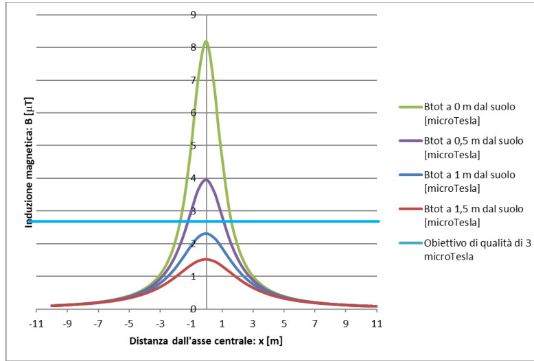
Andamento del campo magnetico generato composto da tre terne due da 630 mm 2 e una da 120 mm 2
