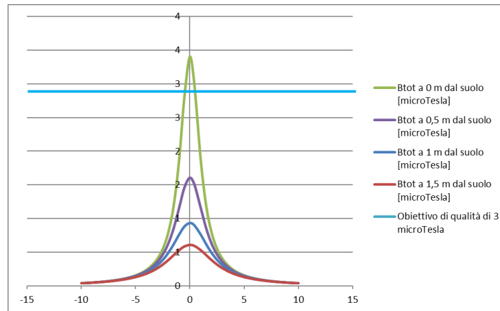
Andamento del campo magnetico generato dal cavidotto, composto da una terna da 400 mm 2
