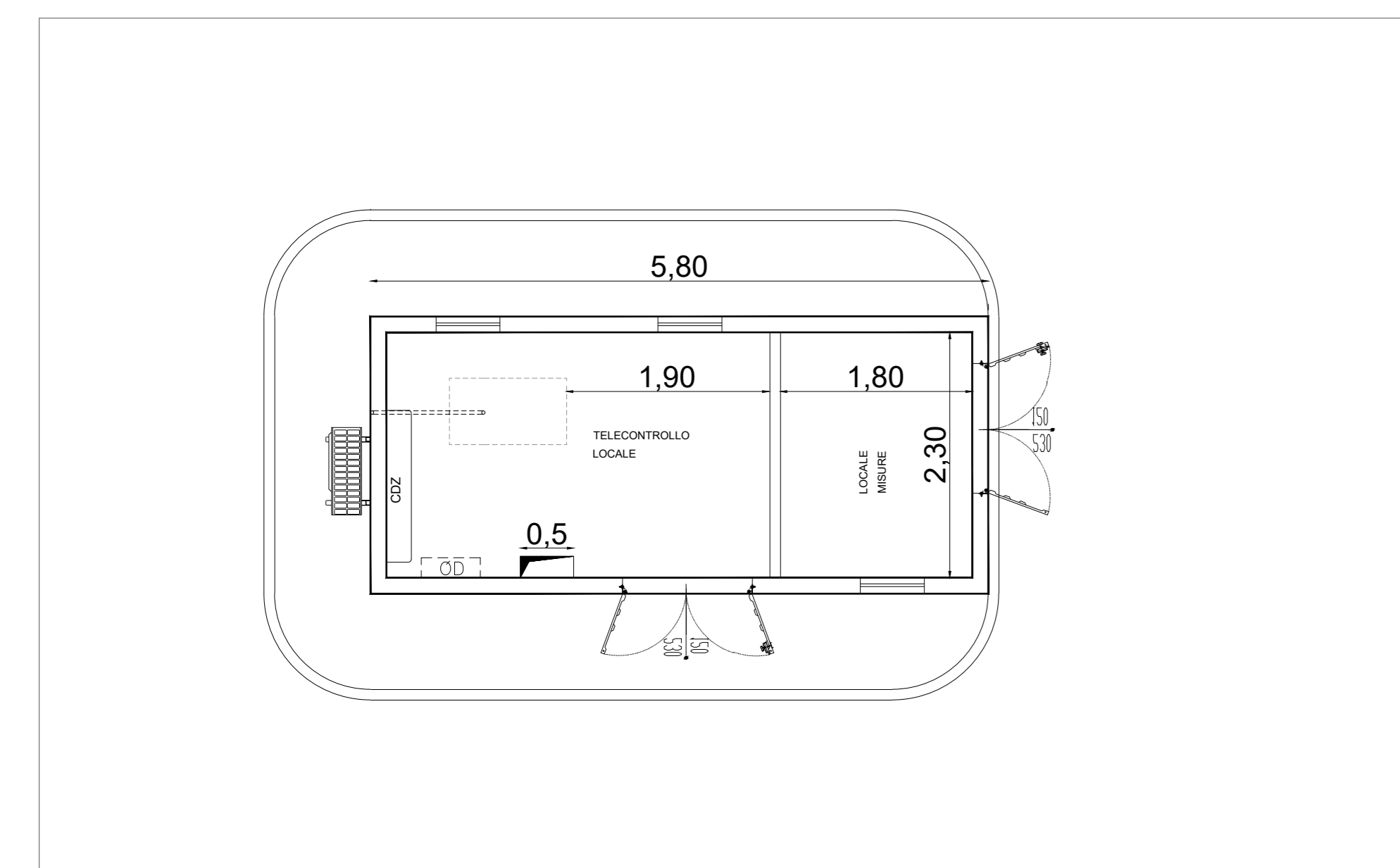
PLANIMETRIA LOCALI TECNICO E TLC Scala 1:50
