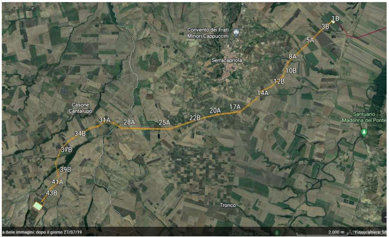
Fig. 2 – Elettrodotto di collegamento (SE) Serracapriola 2 – Rotello (SSE)
