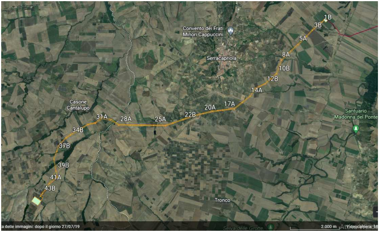
Elettrodotto Serracapriola 2 (SSE smistam) – Rotello (SSE)
