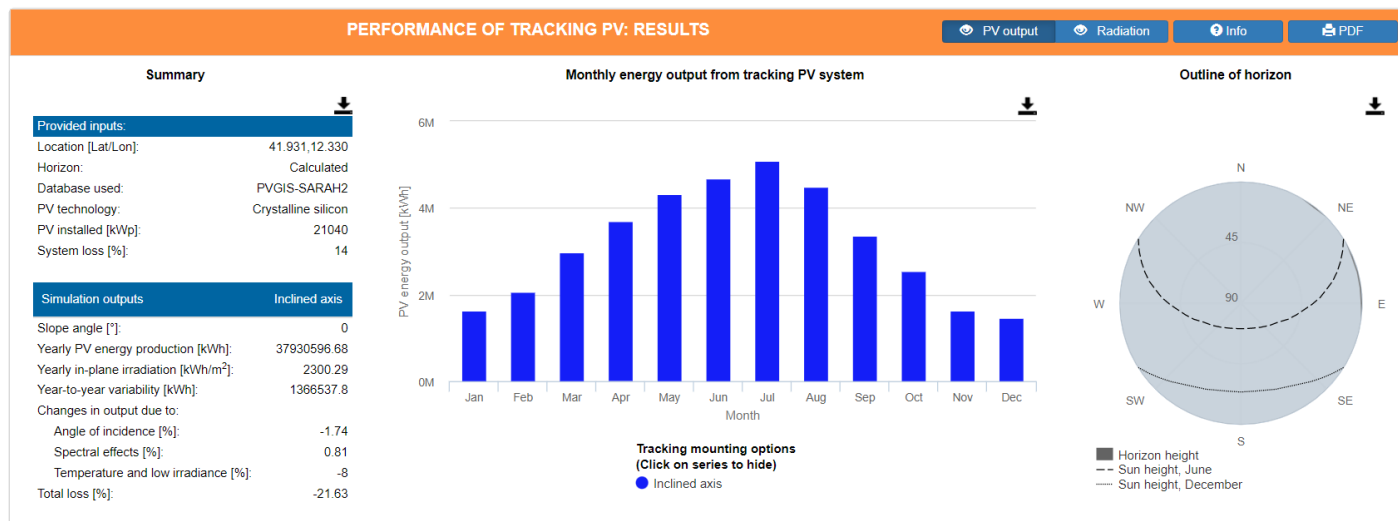
Figura 8 risultato della simulazione PVGIS di un impianto fotovoltaico sulla stessa area
