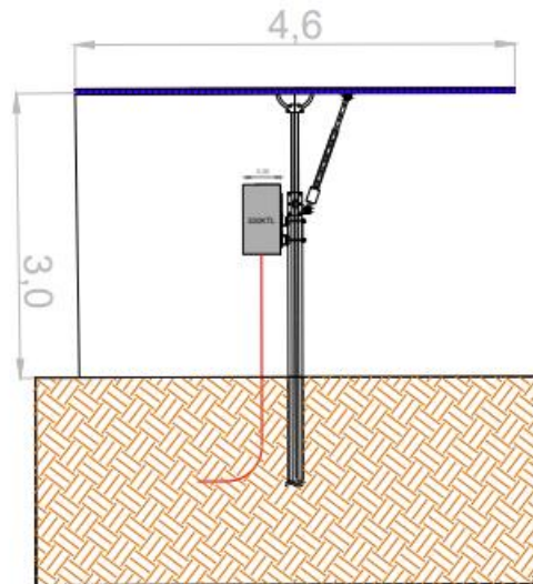
Figura 9 tipico strutture tracker
