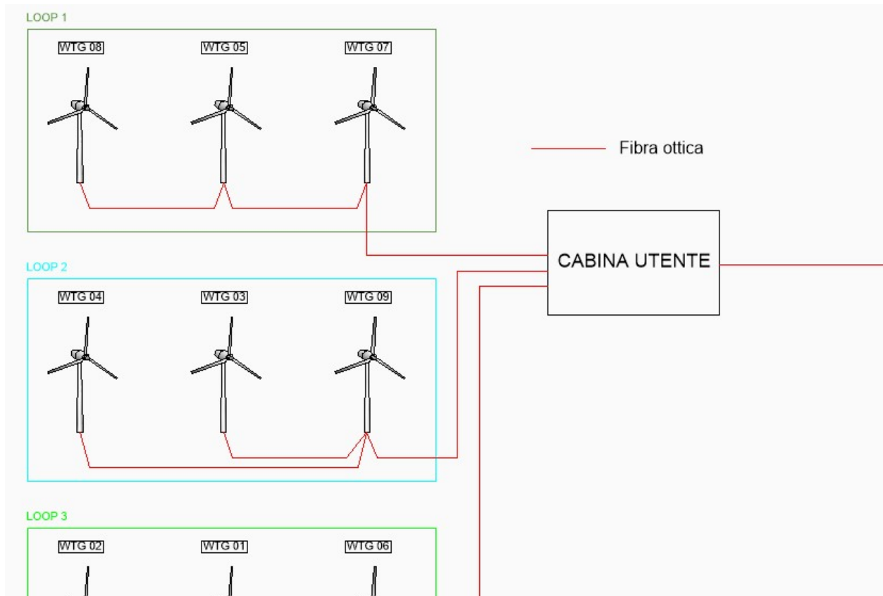
Figura 5 - Schema fibra ottica
