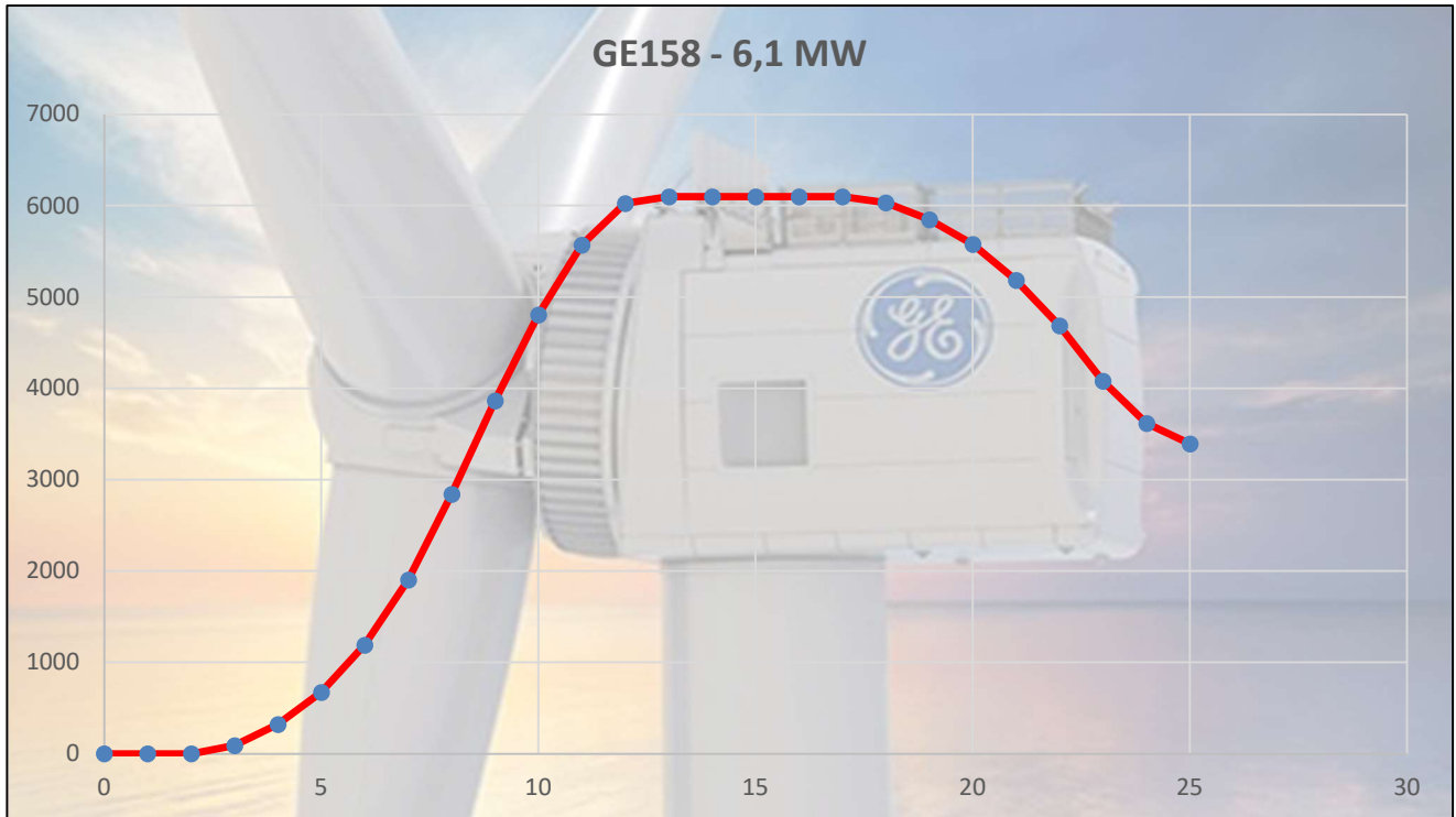
Figura 6 - Grafico curva di potenza dell'aerogeneratore
