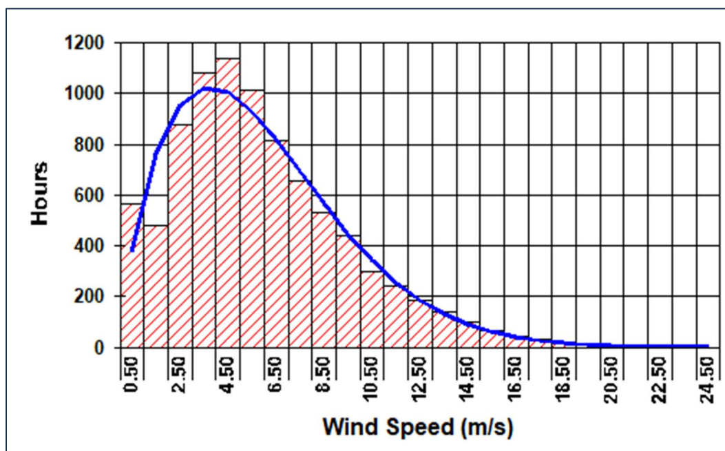
Figura 7 - Distribuzione di Weibull delle velocità del vento
