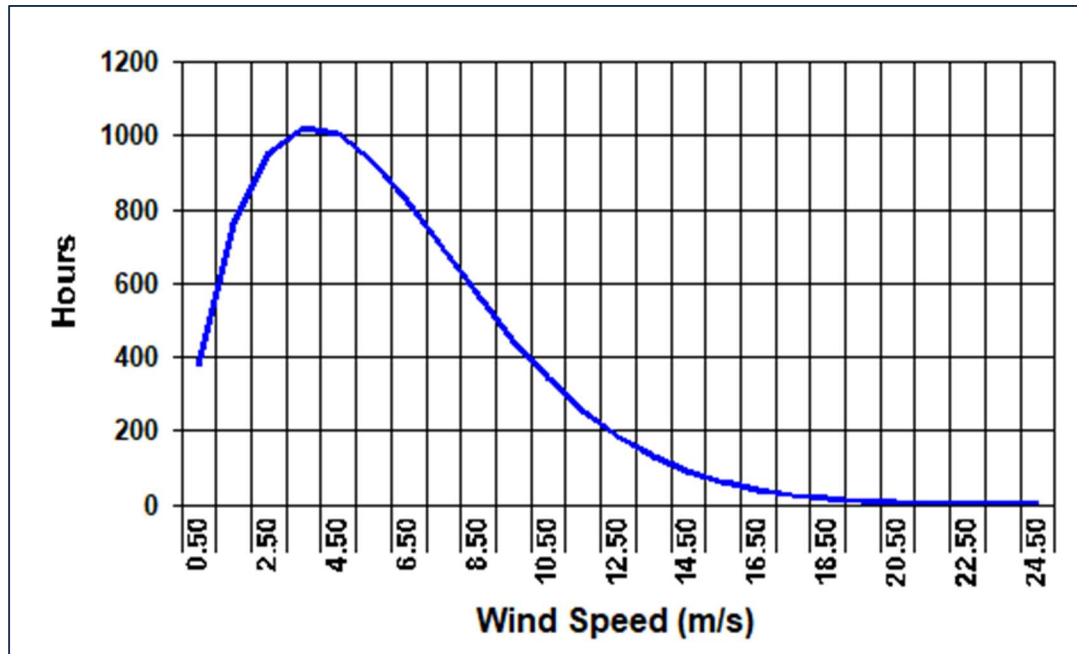
Figura 4 - Distribuzione di Weibull delle velocità del vento
