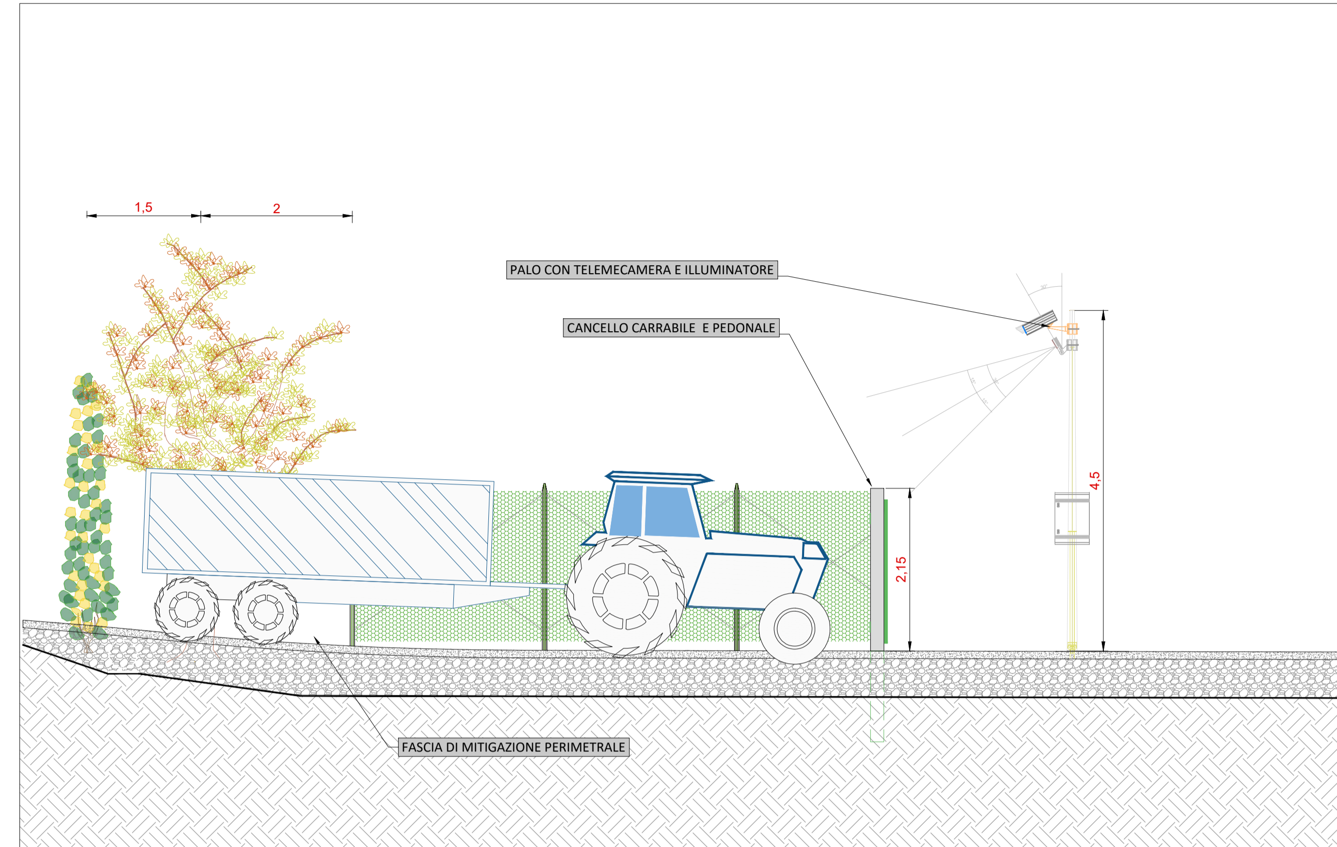
Sezione trasversale - Scala 1:50
