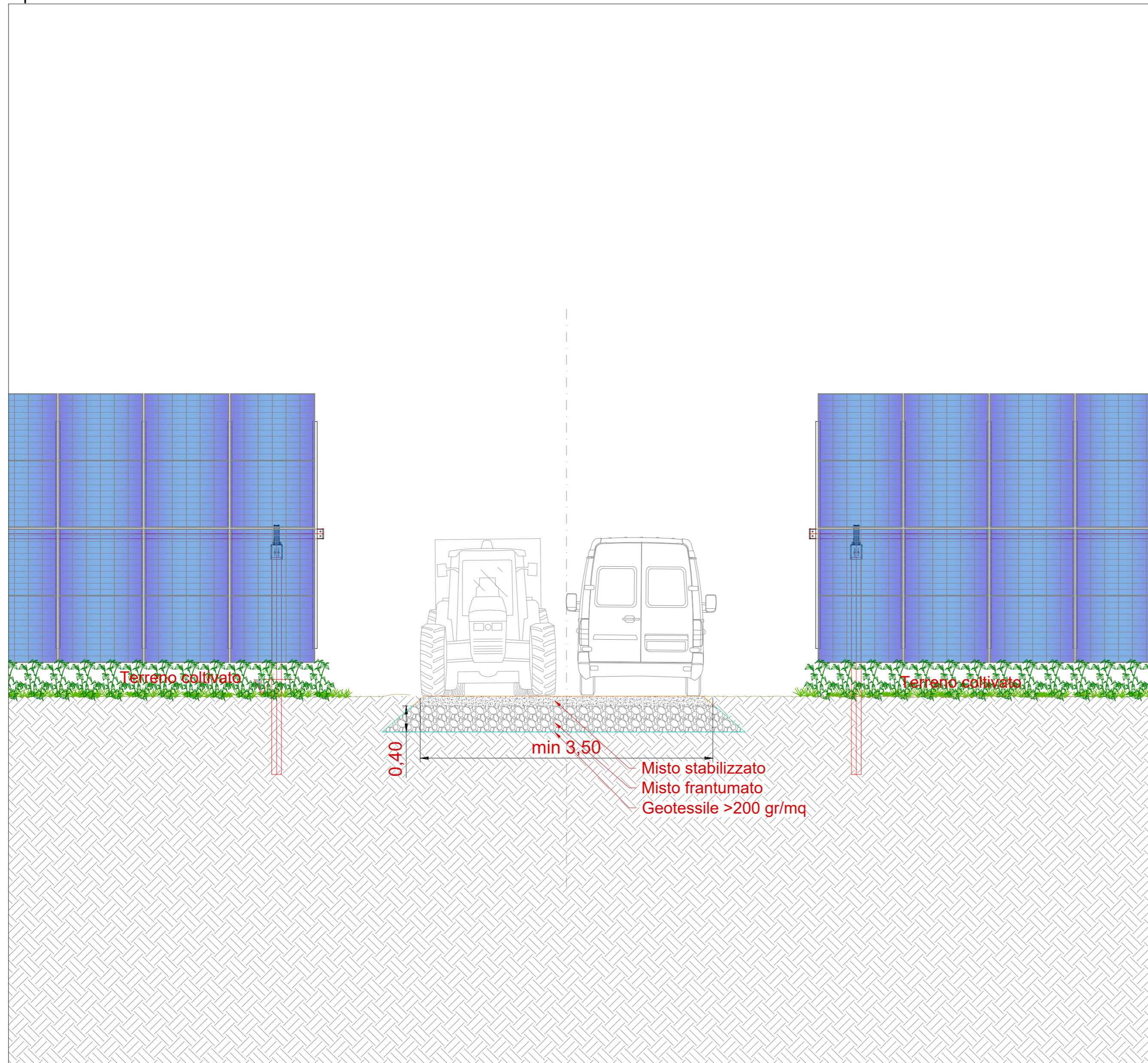
Tipico strada interna - scala 1:50
