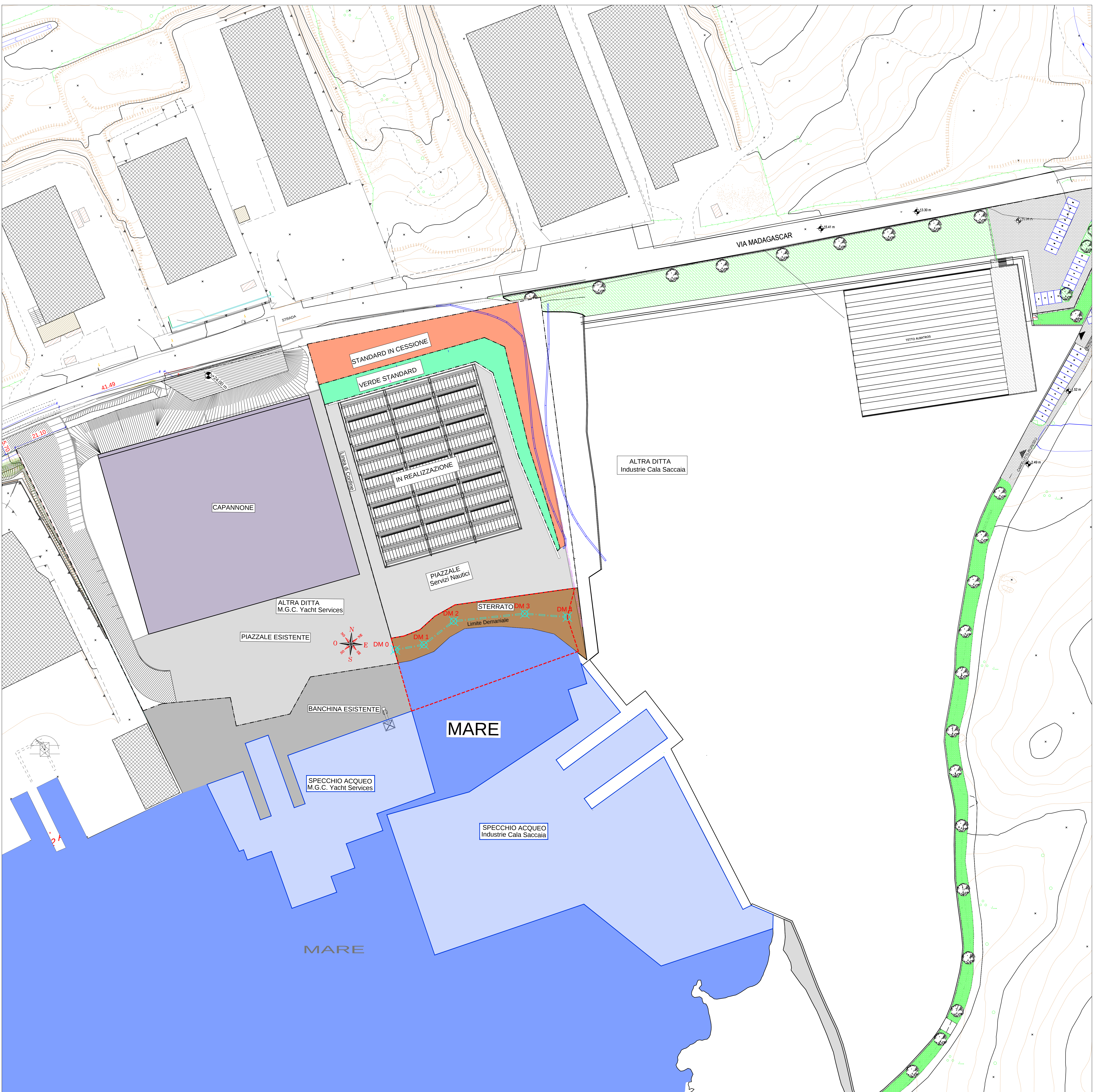
PLANIMETRIA GENERALE
