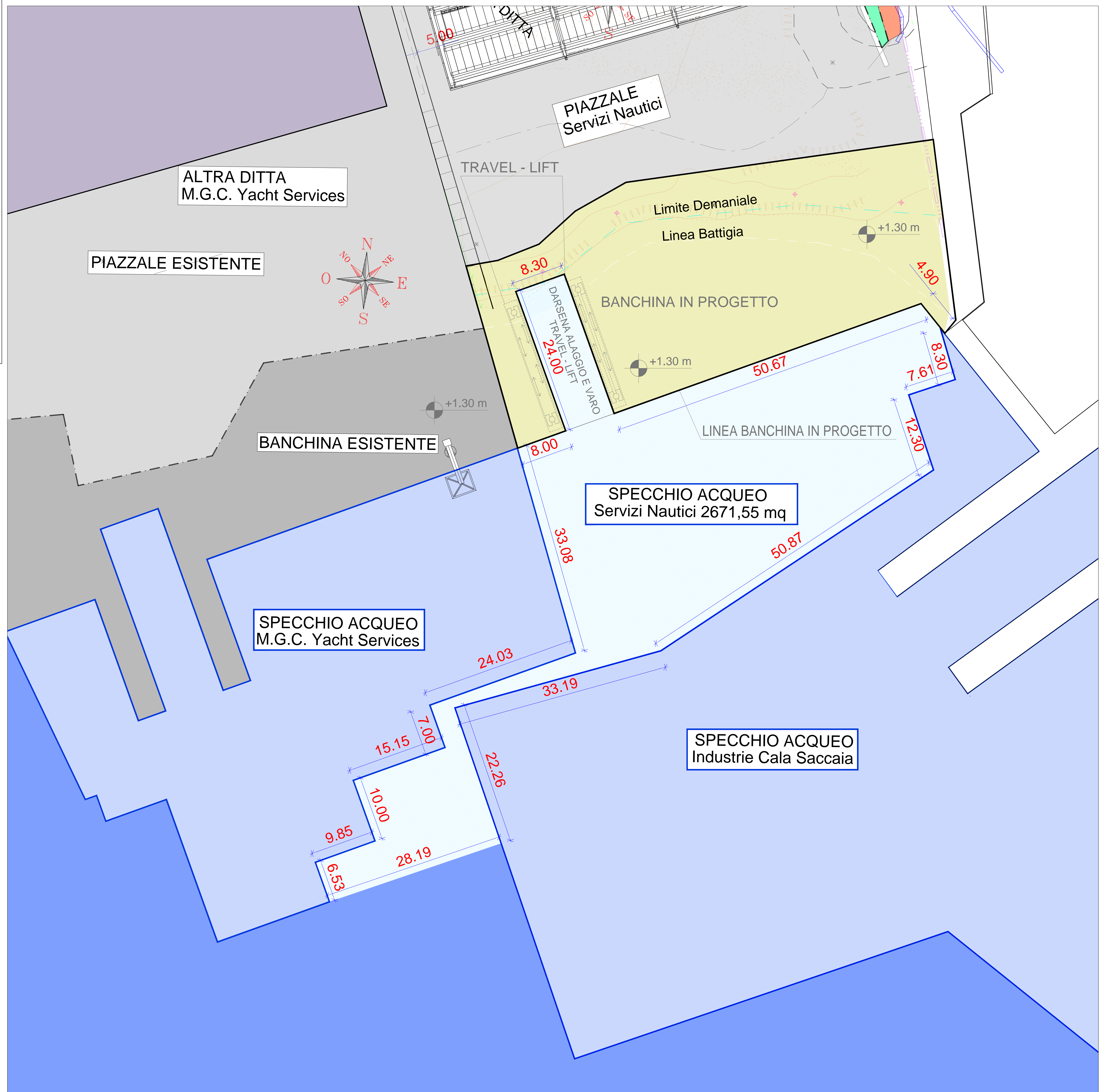
PLANIMETRIA GENERALE DI PROGETTO
