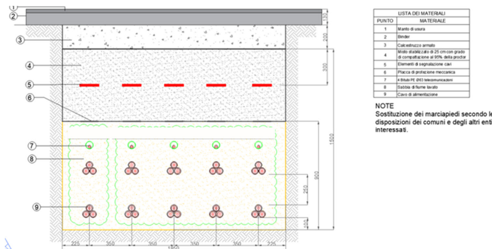
Figura 5. Sezione tipo sotto sede stradale
