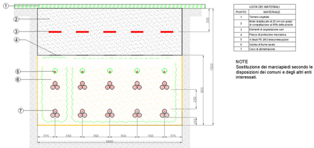
Figura 6. Sezione tipo in terreno vegetale
