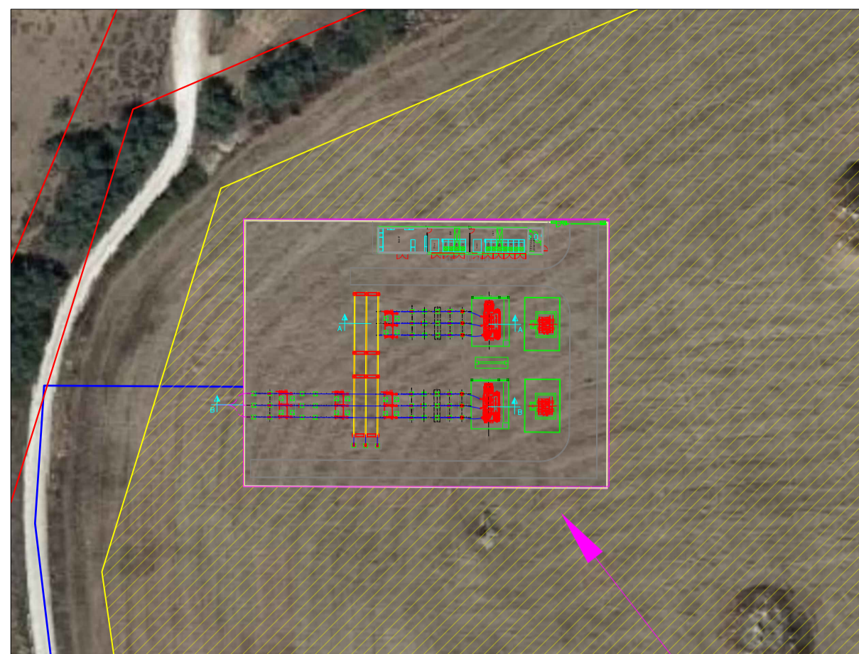
Particolare Stazione utente MT/AT Scala 1:1000
