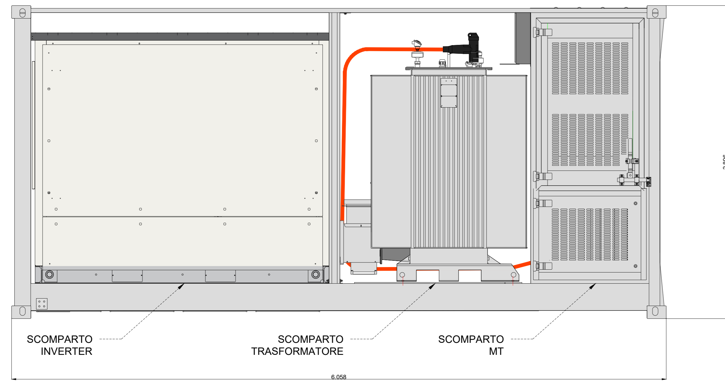
PROSPETTO LATERALE SPS (VISTA CON COMPONENTI)
