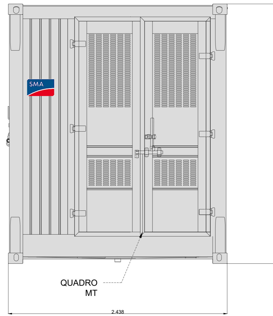
PROSPETTO FRONTALE SPS
