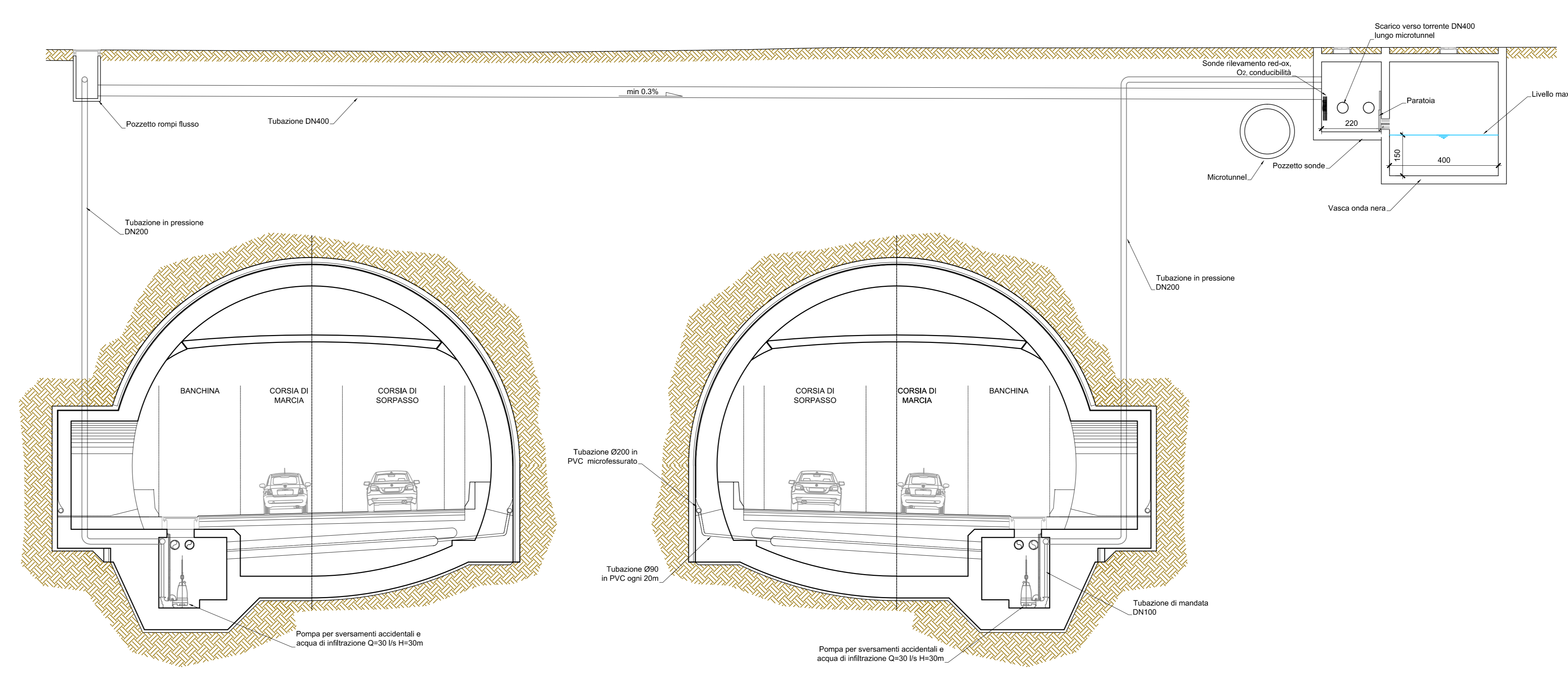
SEZIONE Scala 1:100
