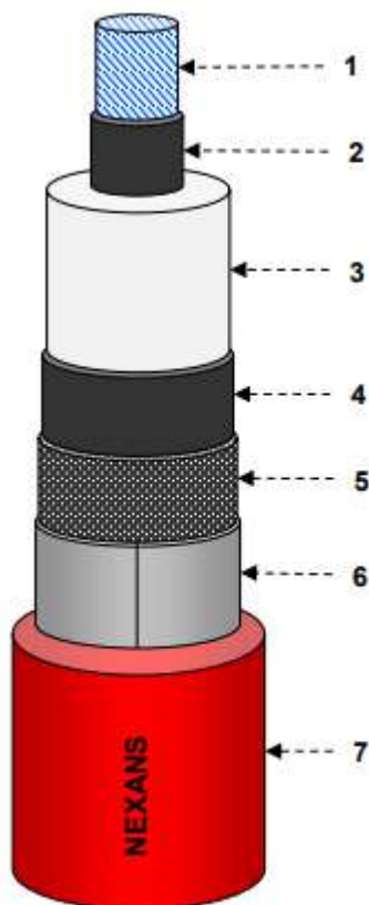
Figura 4 Configurazione tipica dei cavi unipolari previsti
