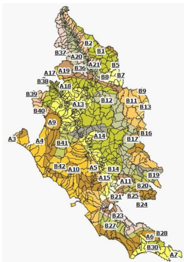
Figura 2: Sottozone omogenee del rapporto VAPI Roma- Pescara
