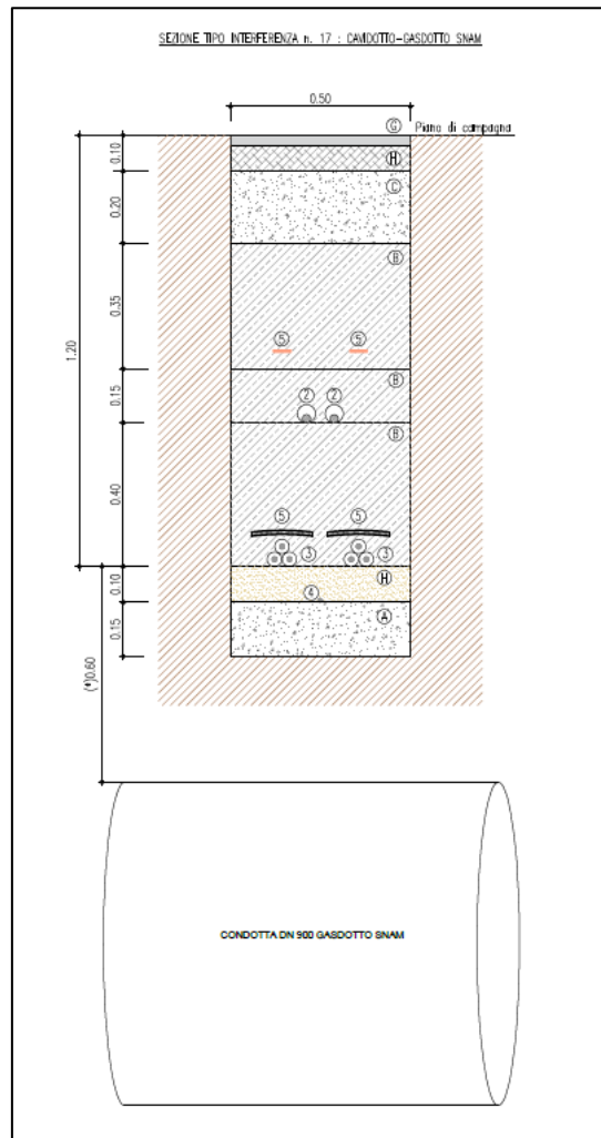
Figura 5: sezione tipologica dell'interferenza tra cavidotto-gasdotta SNAM
