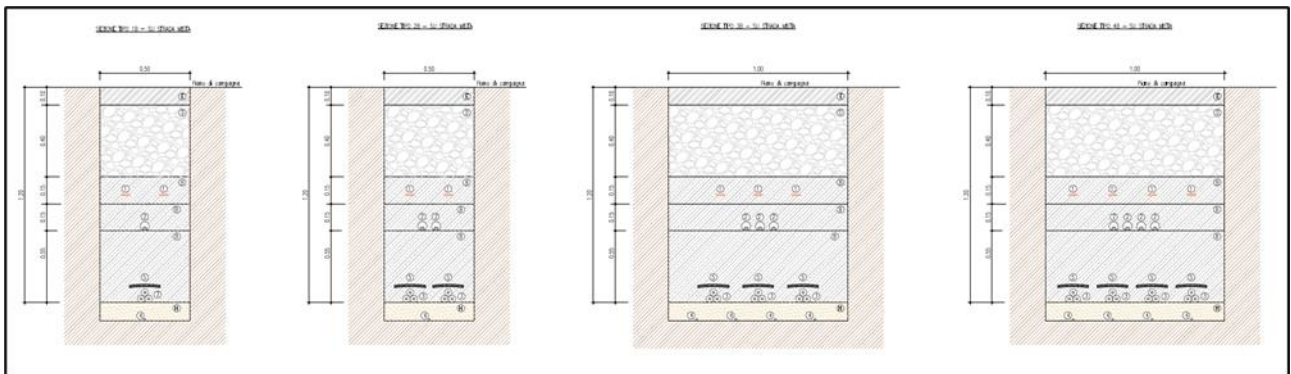
Figura 5: sezioni tipologiche del cavidotto su strada mista
