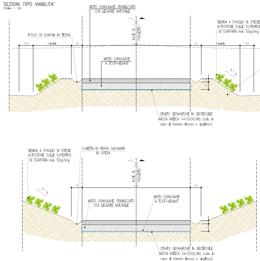
Figura 3: sezione tipologica viabilità di parco
