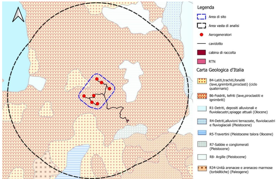
Figura 7: Stralcio Carta Geologica d'Italia (Fonte: Geoportale Nazionale).
