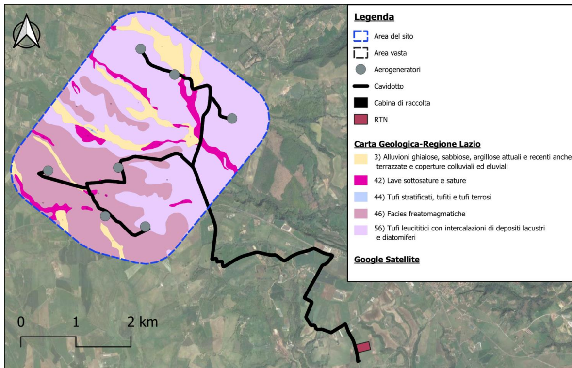
Figura 8: Stralcio Carta Geologica Regione Lazio (Fonte: Geoportale Lazio, 2012).
