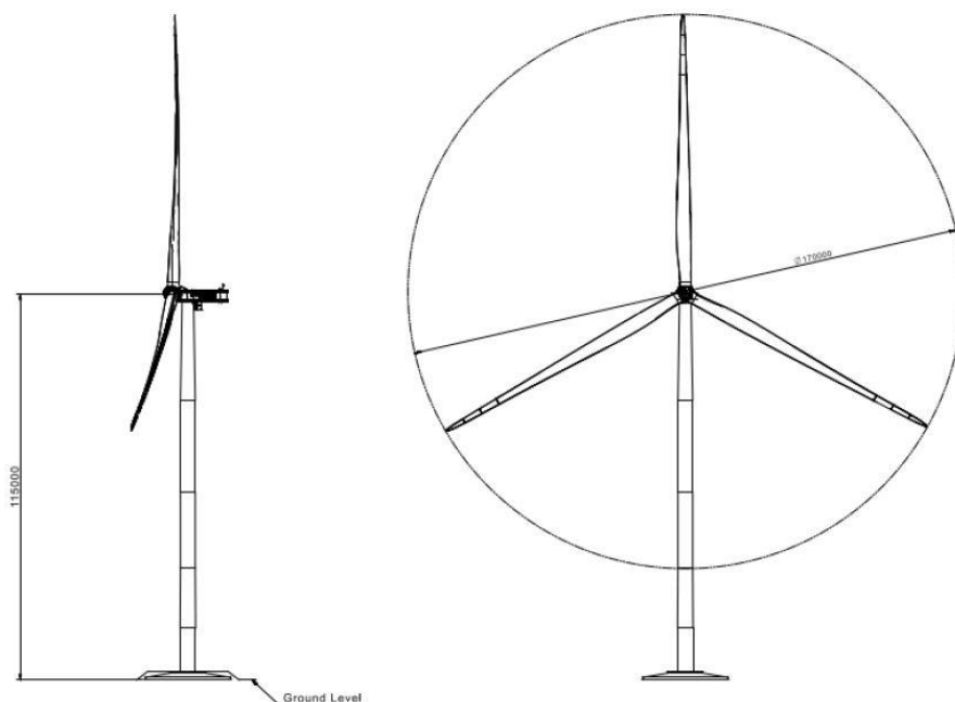
Figura 1: Vista aerogeneratore
