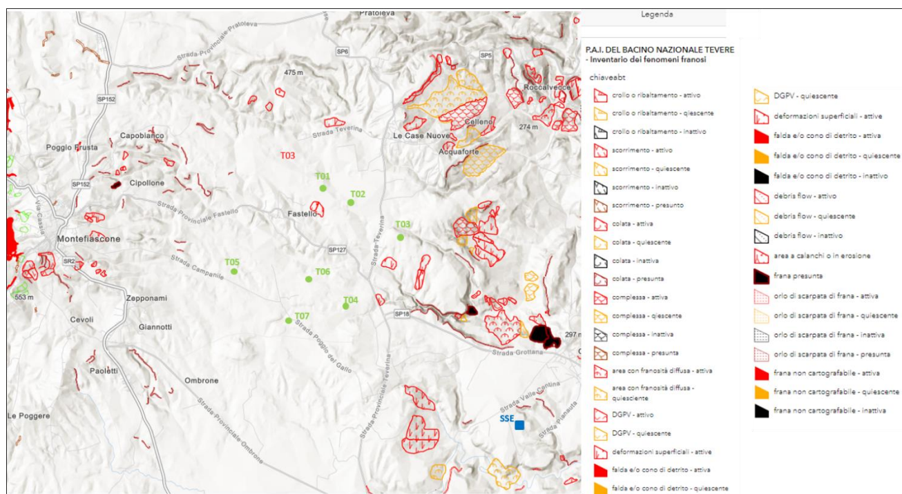
Fig. 03: PAI dell'Autorità di Bacino distrettuale dell'Appennino Centrale - Bacino del Fiume Tevere, relativo al sito di progetto (in verde l'area di imposta degli aerogeneratori ed in blu l'area di imposta della sottostazione)
