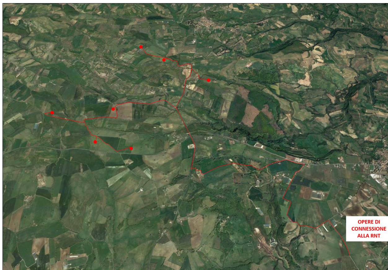
Fig 01: Inquadramento su ortofoto dei siti d'imposta degli aerogeneratori e delle opere di connessione alla RNT
