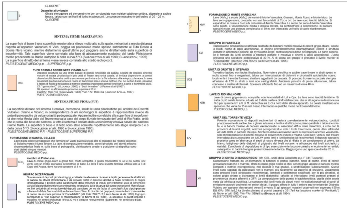
Fig. 02: Stralcio del Foglio 345 "Viterbo" della Carta Geologica d'Italia, scala 1:50.000 relativo al sito di progetto (in rosso area di imposta degli aereogeneratori ed in blu area di imposta della sottostazione)
