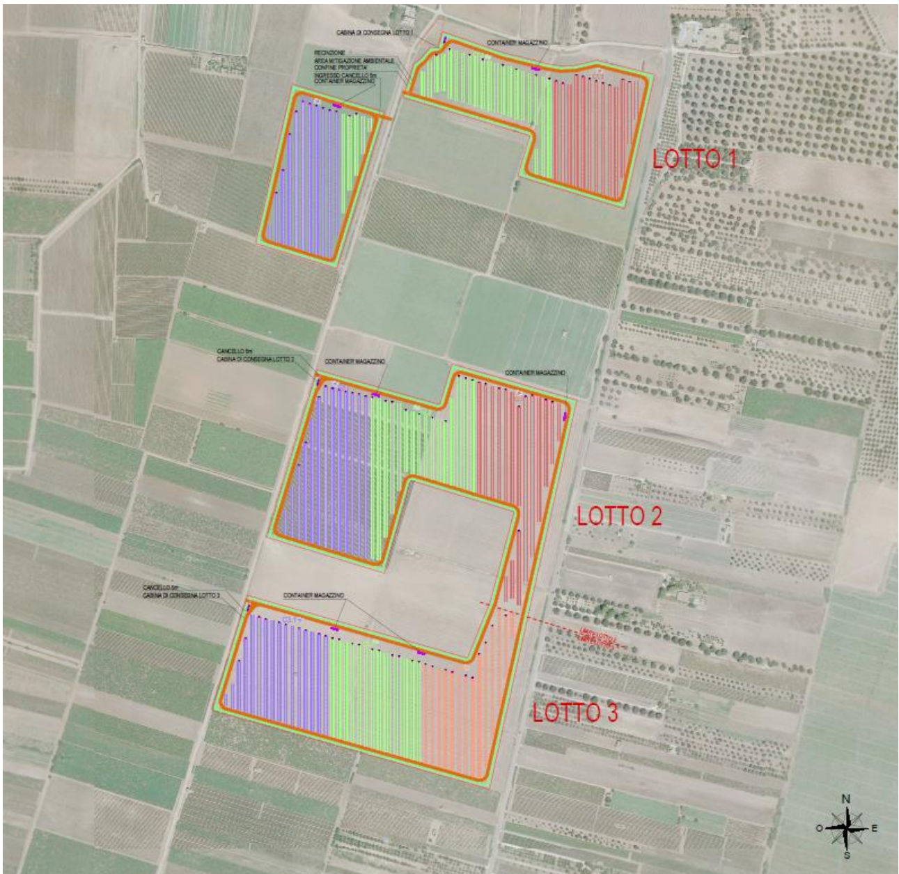
Figura 2-e - Layout d'impianto
