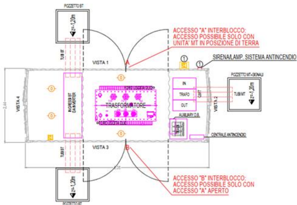
Figura 3-c – Immagine esemplificativa della cabina di trasformazione BT/MT
