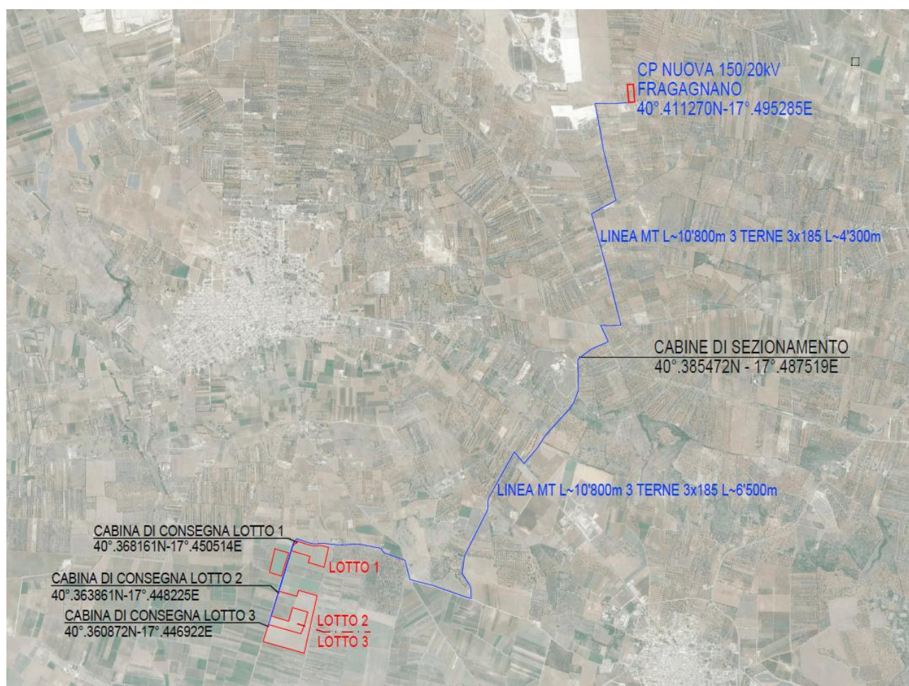
Figura 2-d – Inquadramento dell'impianto FV ed opere di connessione su ortofoto
