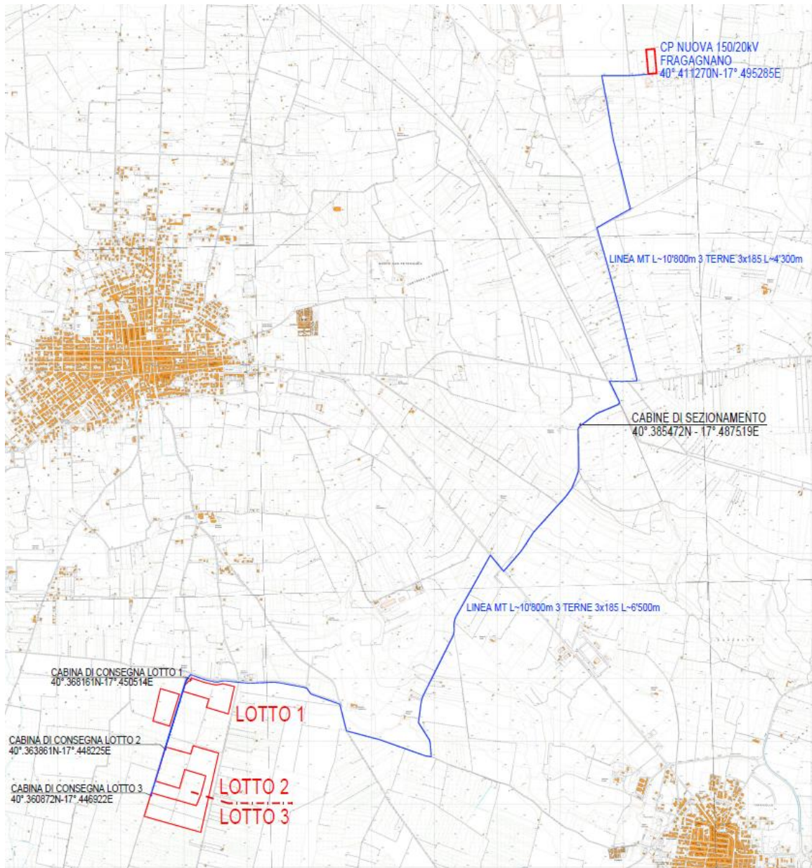
Figura 3-g - Percorso dell'elettrodotto MT su CTR
