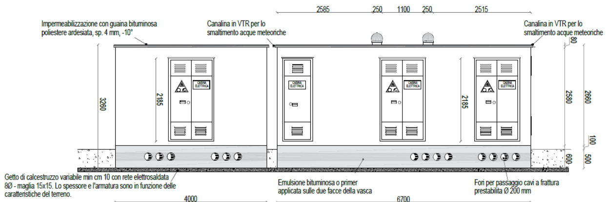
Figura 3-e - Cabina di consegna - Vista laterale
