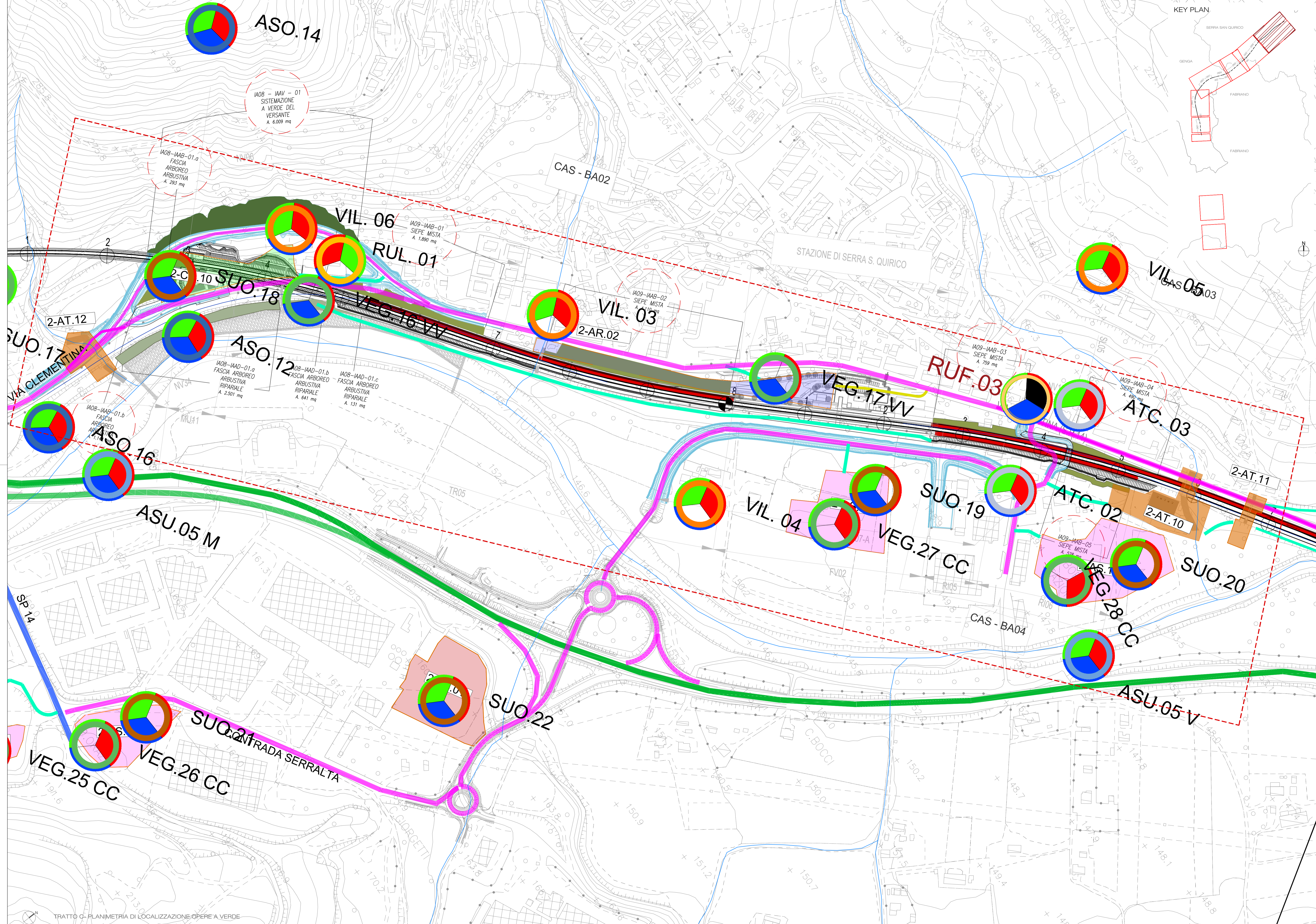
TRATTO C - PLANIMETRIA DI LOCALIZZAZIONE OPERE A VERDE
