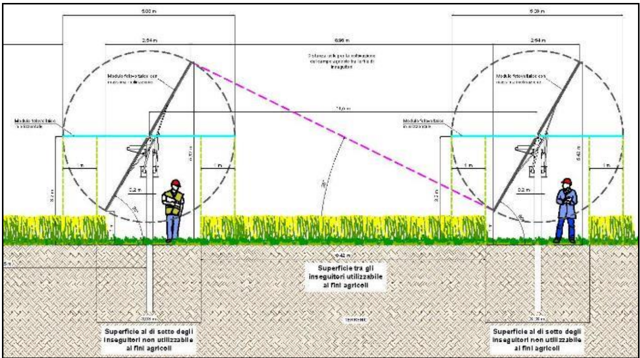
Figura 3: Altezza media dei moduli fotovoltaici e superficie destinata alle coltivazioni agricole
