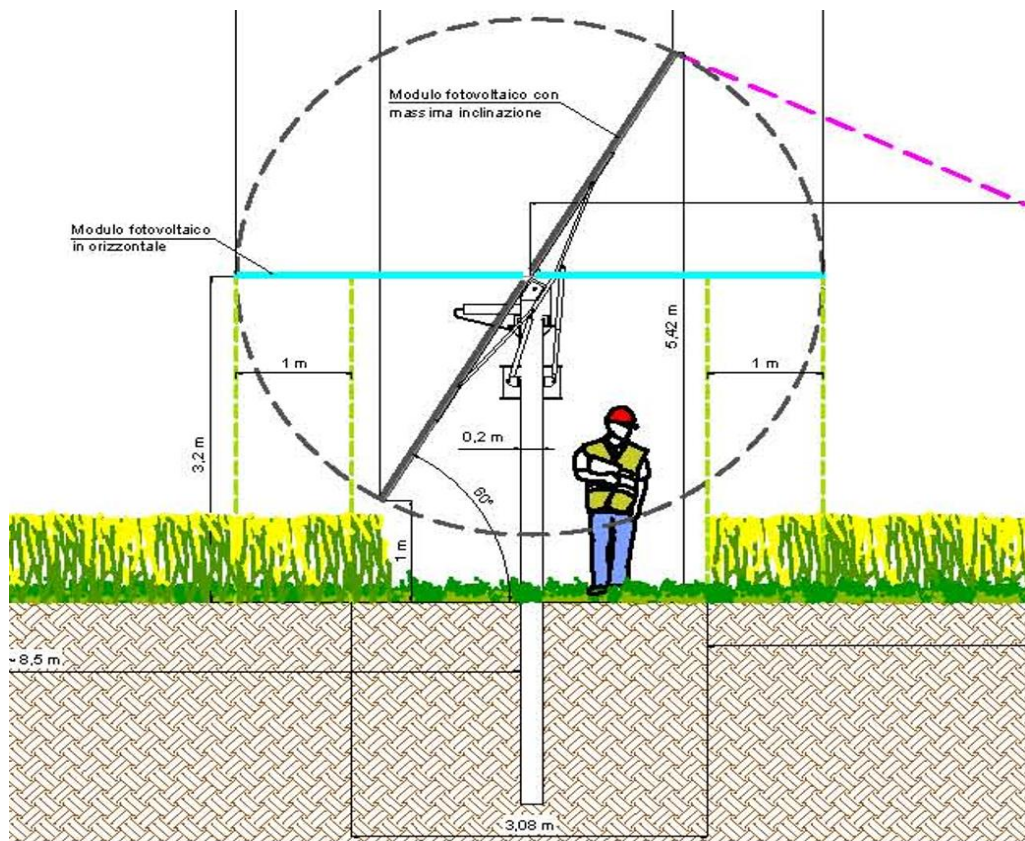
Figura 4: Particolare dei moduli fotovoltaici e dei relativi ingombri rispetto alla superficie agricola coltivata
