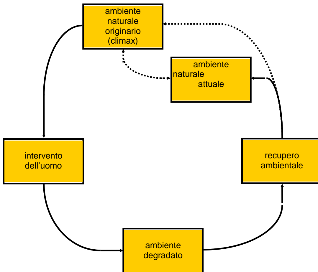
Figura 22: Ciclo ecologico naturale e azione antropica
