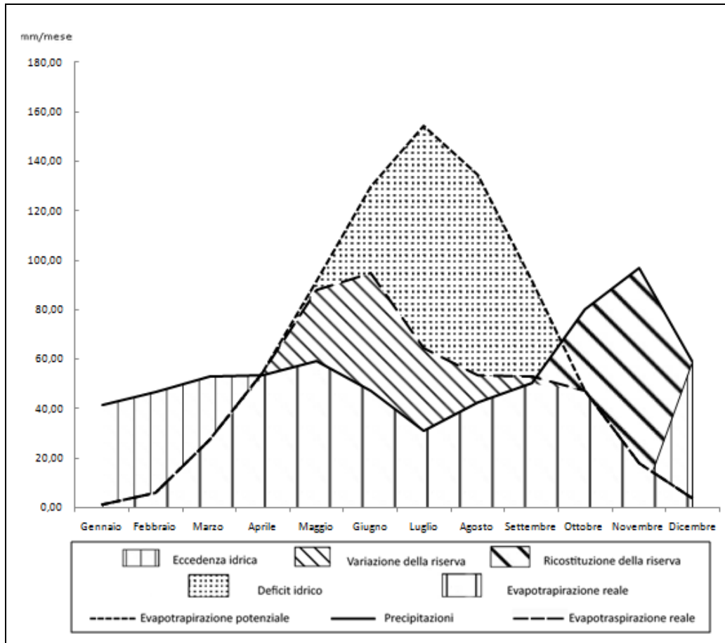
Figura 17: Evapotraspirazione reale e bilancio idrico
