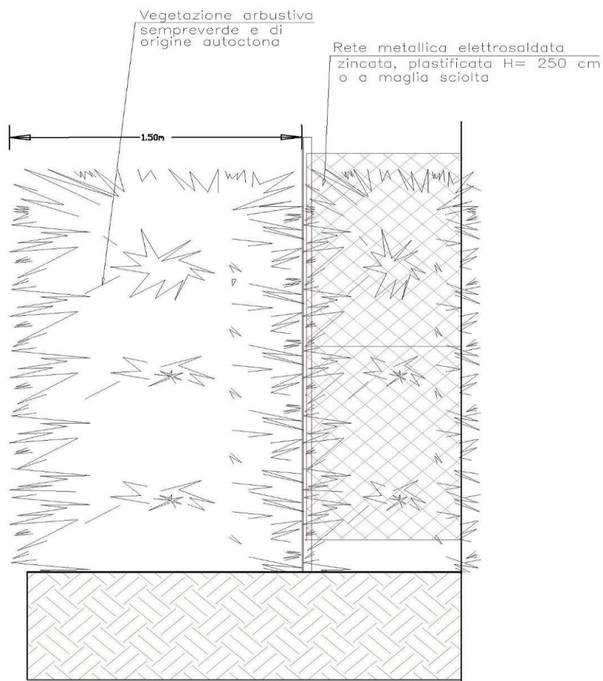
Figura 8: Particolare della recinzione
