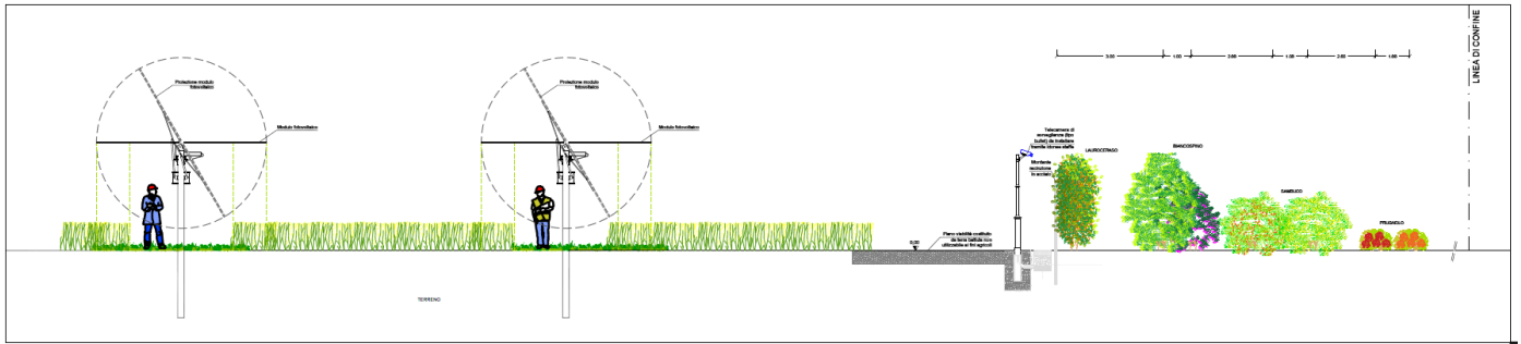
Figura 27: Schema di siepe – Sezione trasversale
