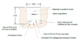
SCAVO PER CAVI DC
