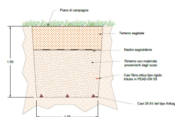
SCAVO SU TERRENO VEGETALE
