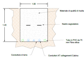
SCAVO PER CAVI AT
