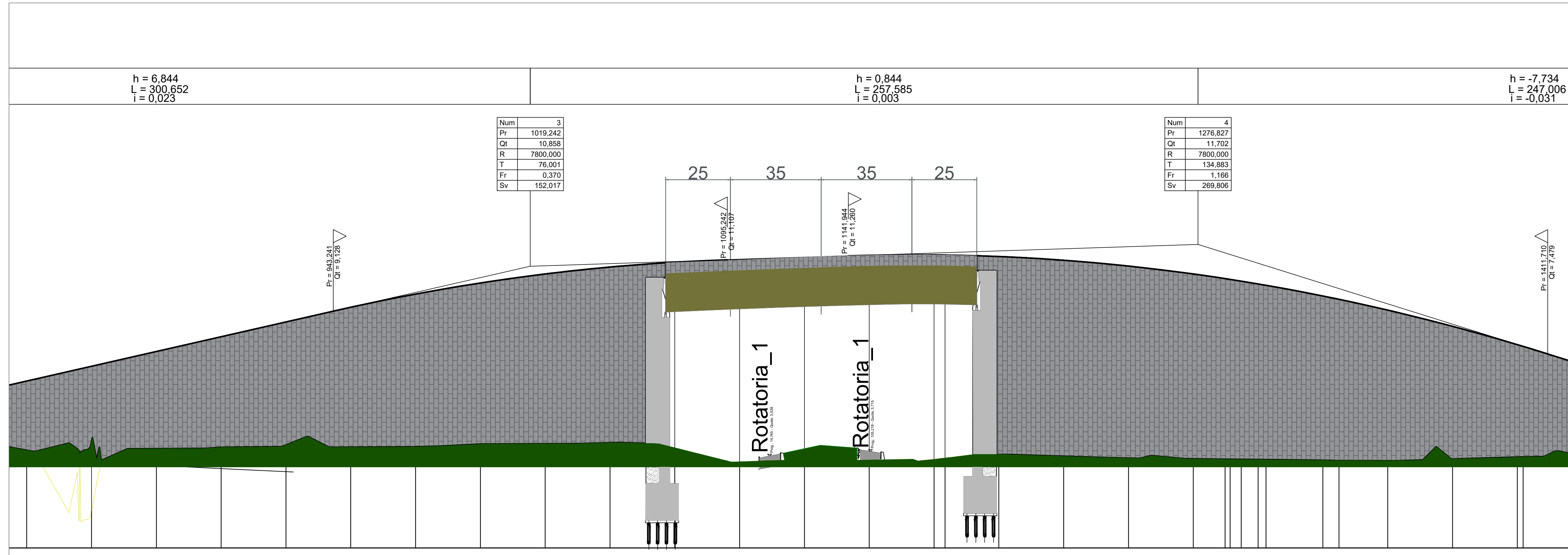
PROFILO - scala 1:1000 / 1:100
