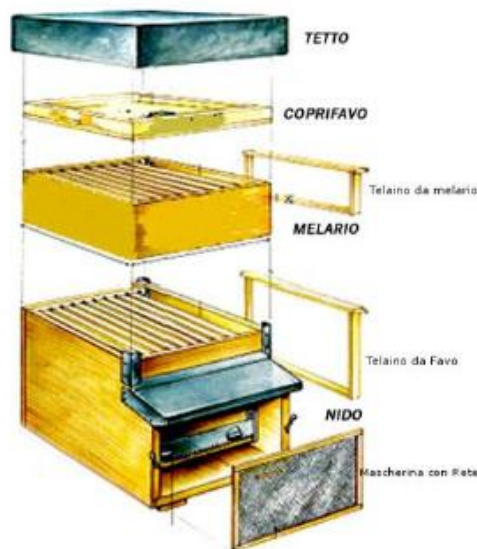
Figura 48 – Componenti dell'arnia
