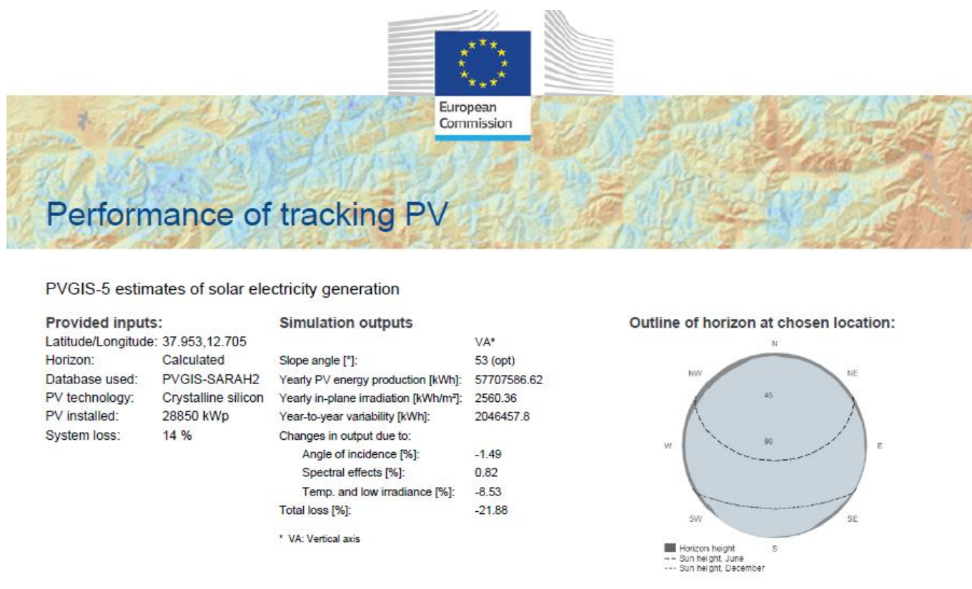
Figura 20 – Dati di irraggiamento per ogni kW installato (fonte: PVGIS)
