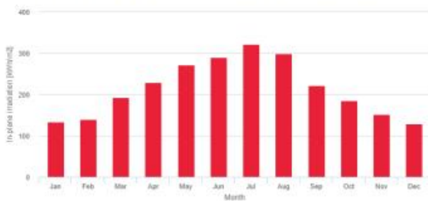
Figura 35 - Rendimento dell'impianto (fonte: PVGIS)
