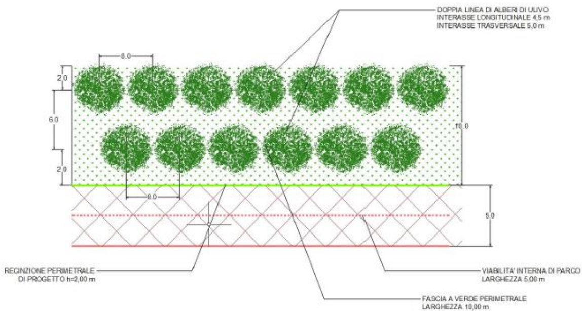
Figura 47 – Dettagli fascia perimetrale
