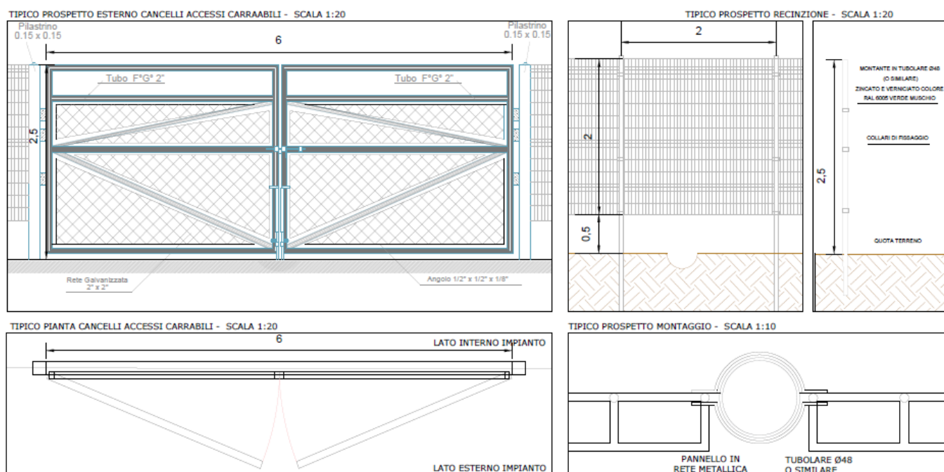
Figura 32 - Particolare Recinzione e cancello di accesso
