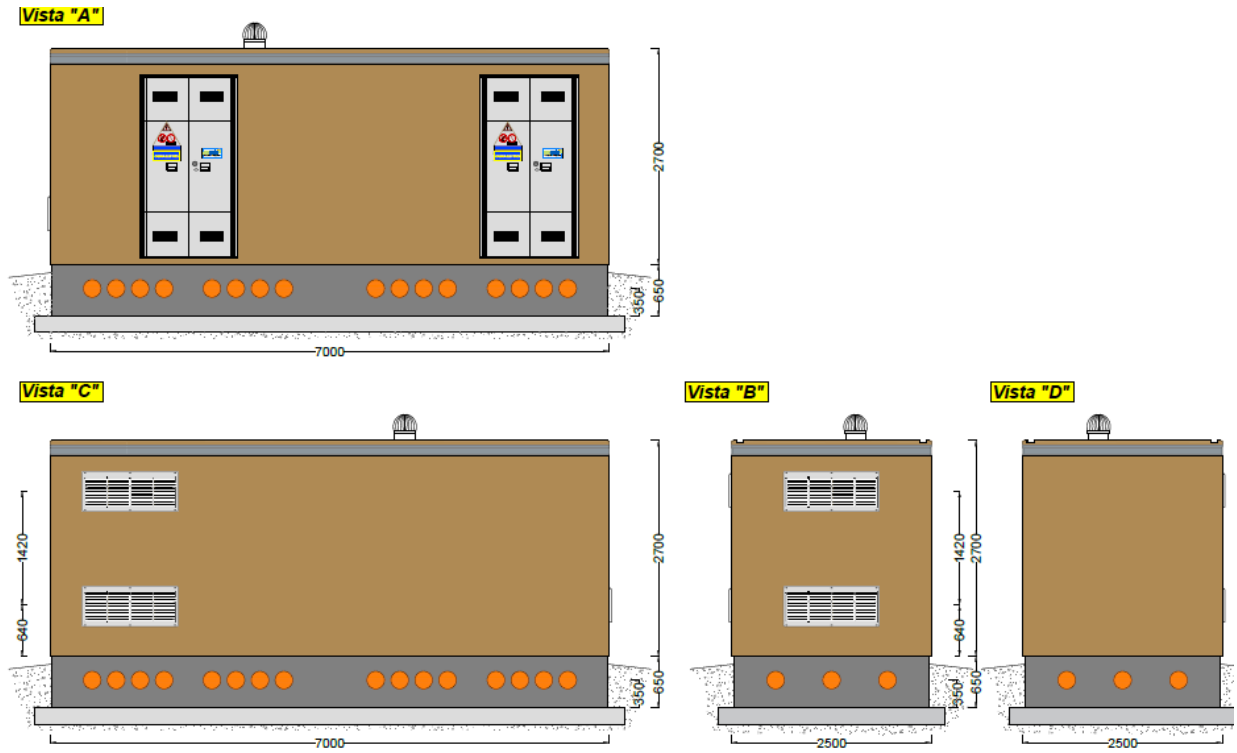
Figura 29 -Cabina utente – prospetti
