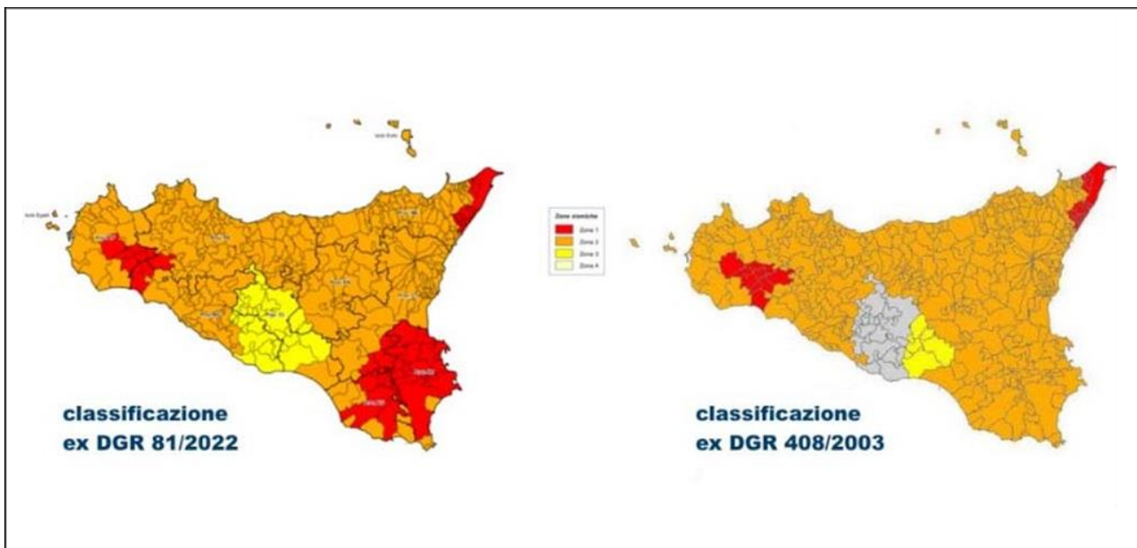
Fig. 44 - Classificazione
