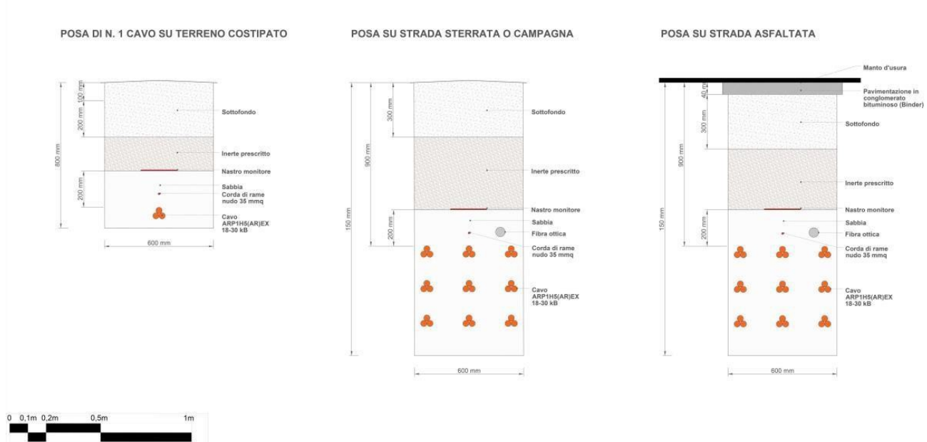
Figura 5 - Sezione tipica di posa della linea in cavo
