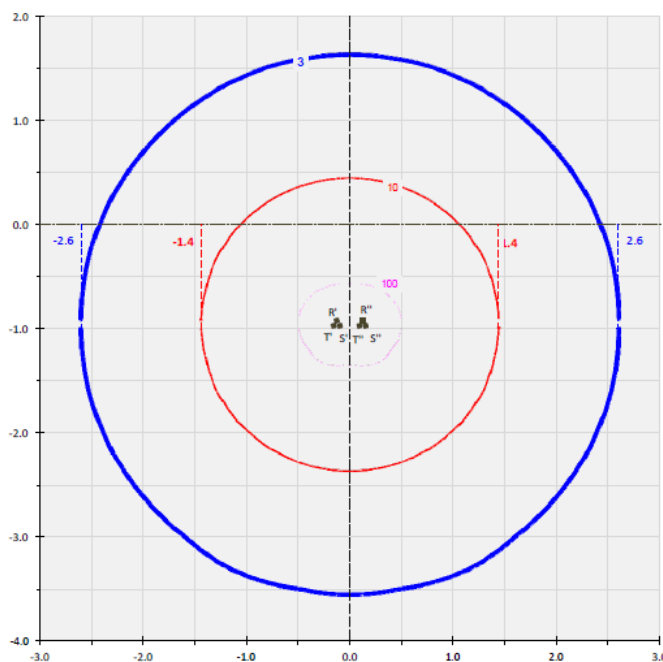
Figura 8 - Curve di equilivello per il campo di induzione magnetica generato da una linea MT posata a trifoglio ( I_{\text{max}}=710\text{A} ; formazione (3x1x630))
