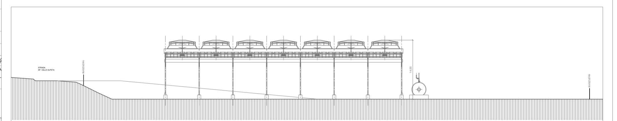
PROFILO A - A' SCALA 1 : 500
