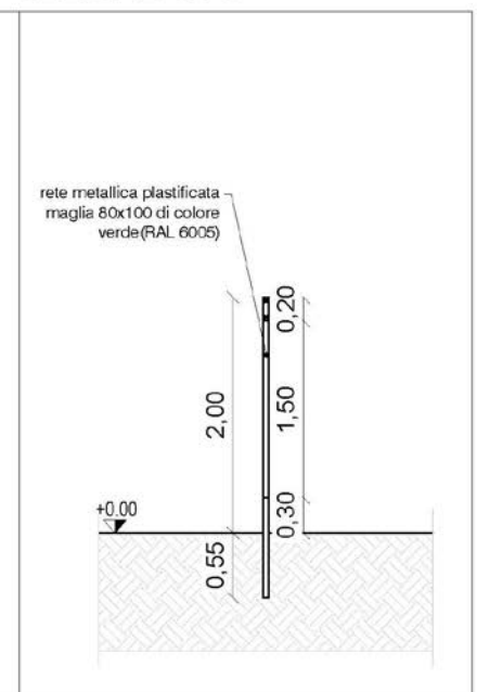
SEZIONE TIPO
