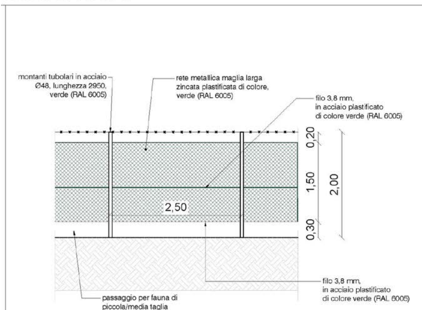
PROSPETTO TIPO
