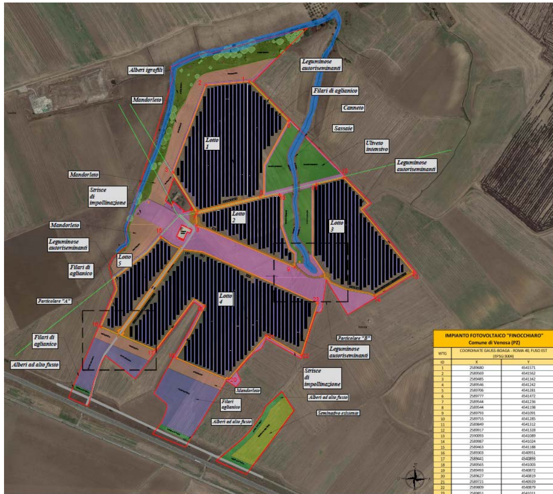
Figura 0.4 Layout impianto agrovoltaico
