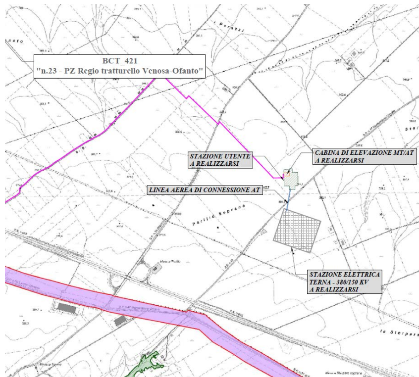
Figura 1. 3 Ubicazione stazione utente e stazione elettrica rispetto ai vincoli del PPR
