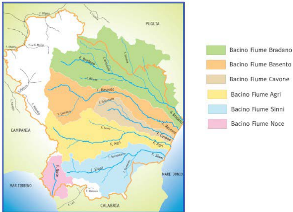
Figura 1. 8 I bacini imbriferi dei principali fiumi lucani.
