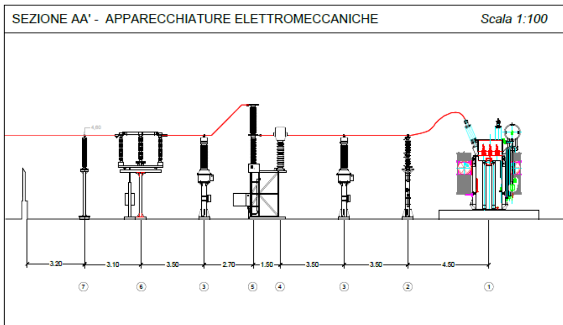
Figura 0.8 Sezione A-A' - Sistema di sbarre di raccolta AT
