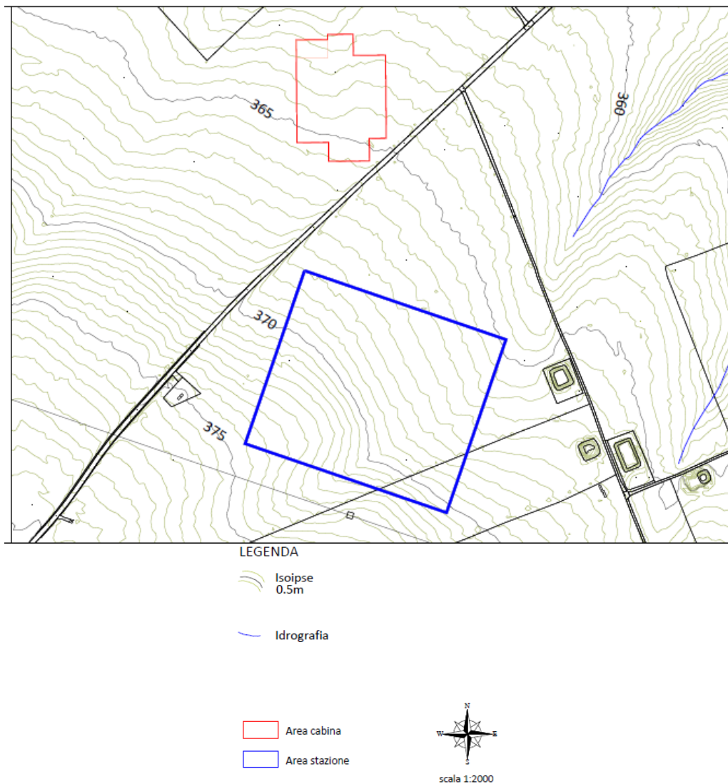
Figura 1. 5 Carta geomorfologica dell'area occupata dalla futura stazione elettrica e dalla stazione utente
