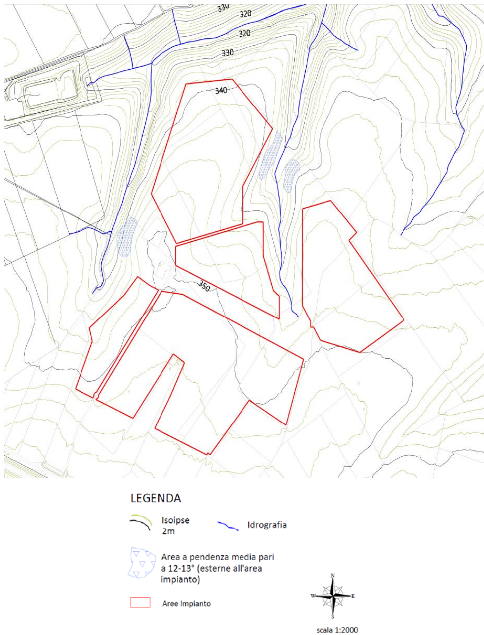
Figura 1. 4 Carta geomorfologica nell'area di impianto
