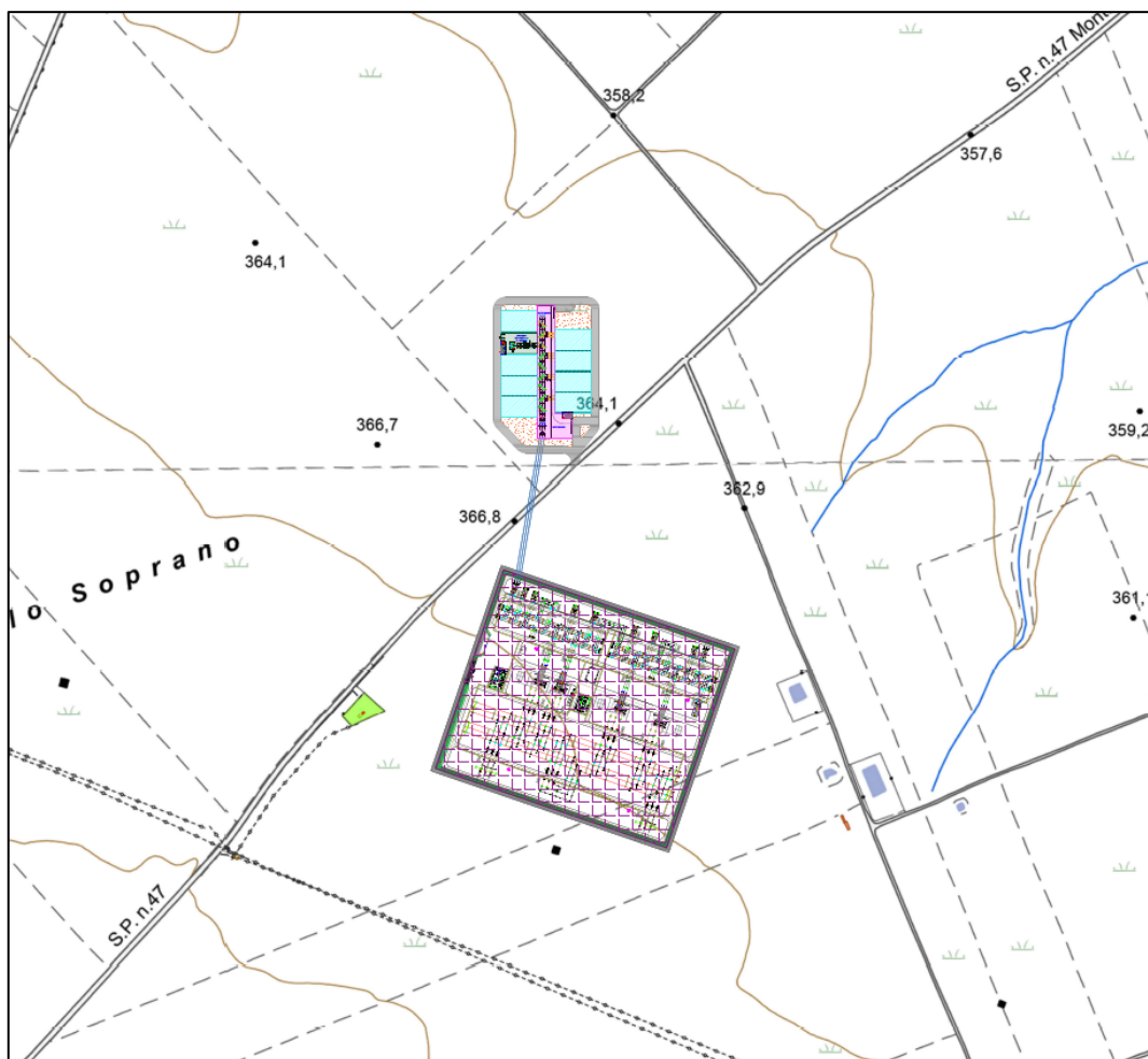
Figura 0.11 Stazione utente
