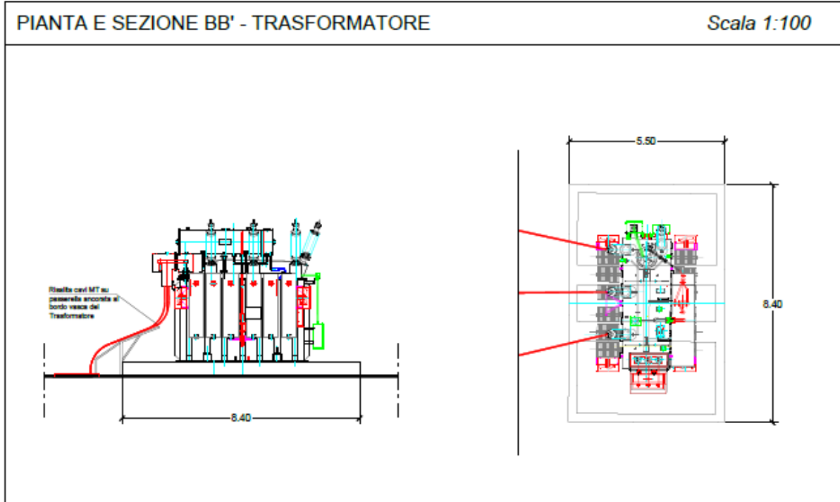
Figura 0.9 Sezione B-B' - Trasformatore
