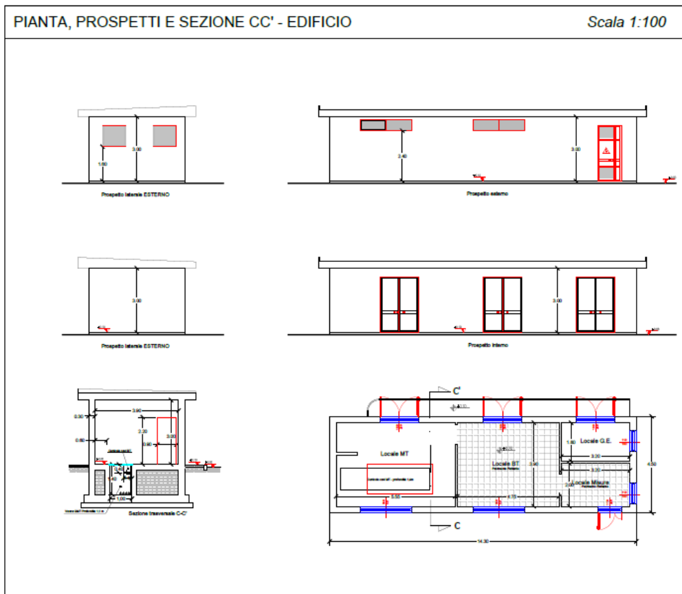
Figura 0.10 Locali tecnici stallo di elevazione AT/MT
