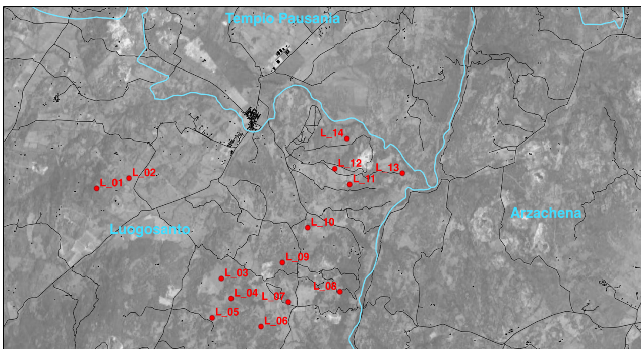
FIGURA 1 – Inquadramento territoriale dell'impianto eolico di 14 WTG (in rosso)
