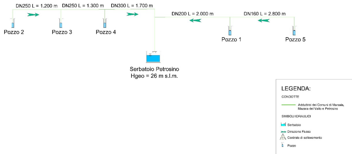
Schema approvvigionamento idrico comune di Petrosino
