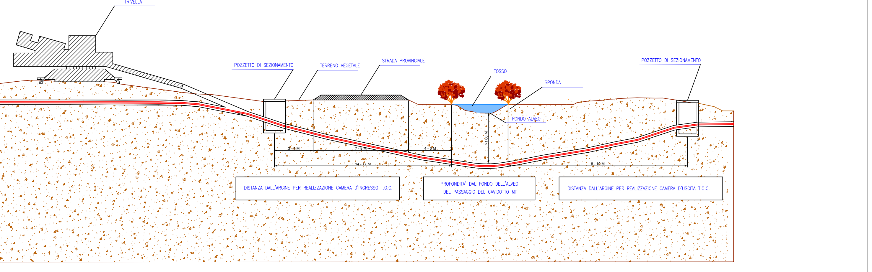
"SEZIONE TRASVERSALE TIPO (A-A) - ATTRAVERSAMENTO FOSSO e PROVINCIALE CON T.O.C." - INTERSEZIONE n.7
