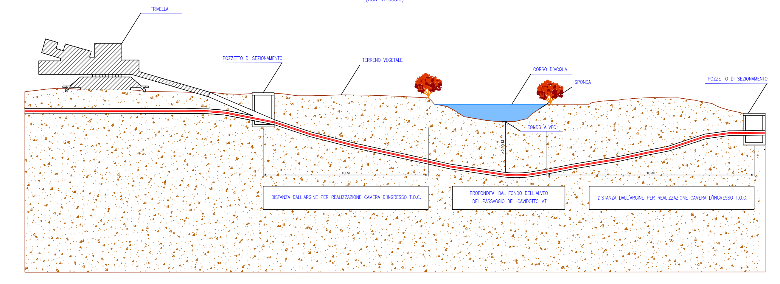
"SEZIONE TRASVERSALE - ATTRAVERSAMENTI FOSSI CON T.O.C." - INTERSEZIONE da n.2 a n.6
