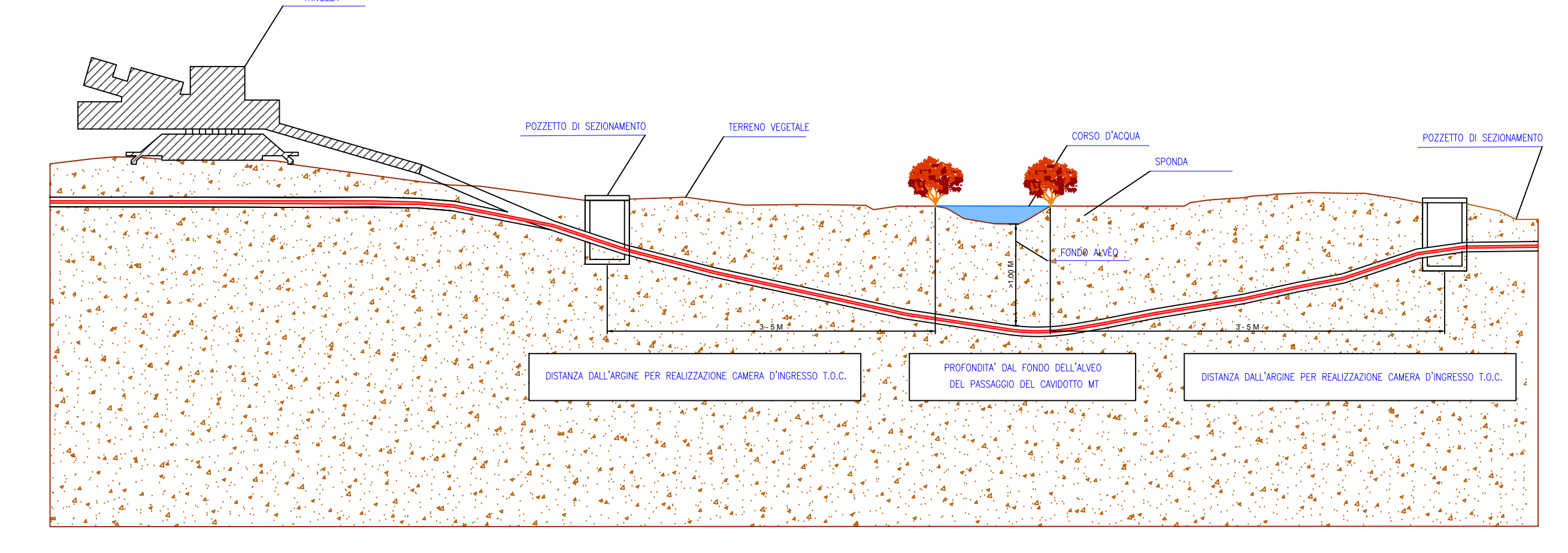
"SEZIONE TRASVERSALE - ATTRAVERSAMENTI FOSSI CON T.O.C." - INTERSEZIONE da n.2 a n.6
