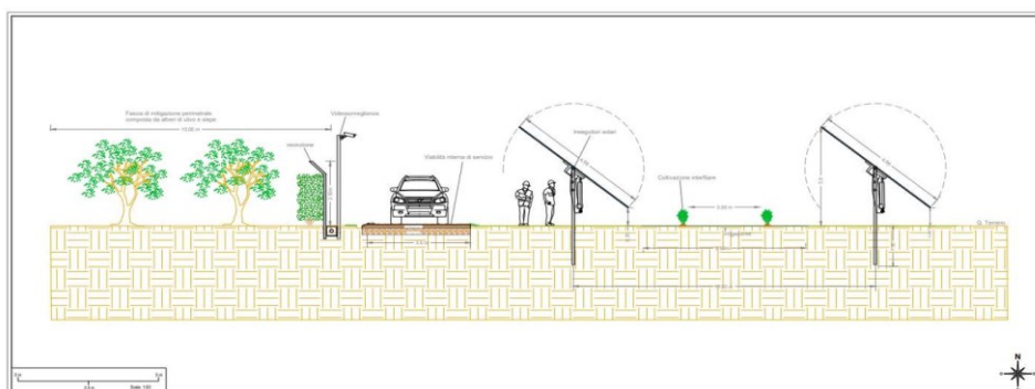
Figura 8 – Schema mitigazione visiva percettiva del progettato
