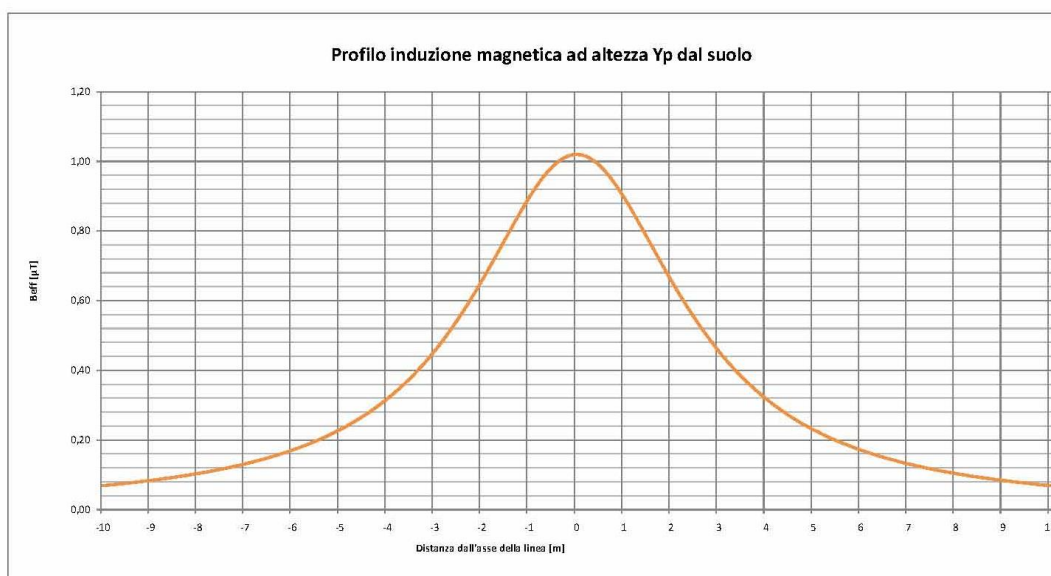
Figura 2: Profilo dell'induzione magnetica calcolata a Y_p=1,5 m di altezza dal suolo.
