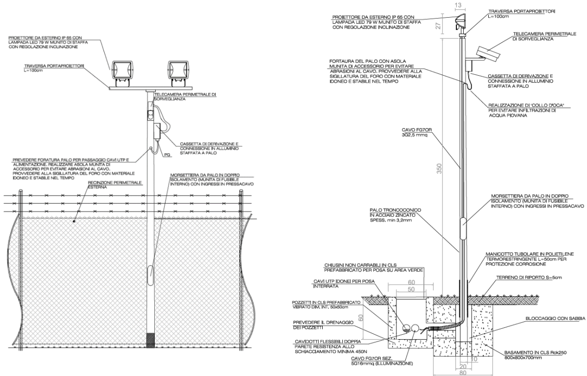
Particolari costruttivi palo di illuminazione perimetrale nell'area di impianto
