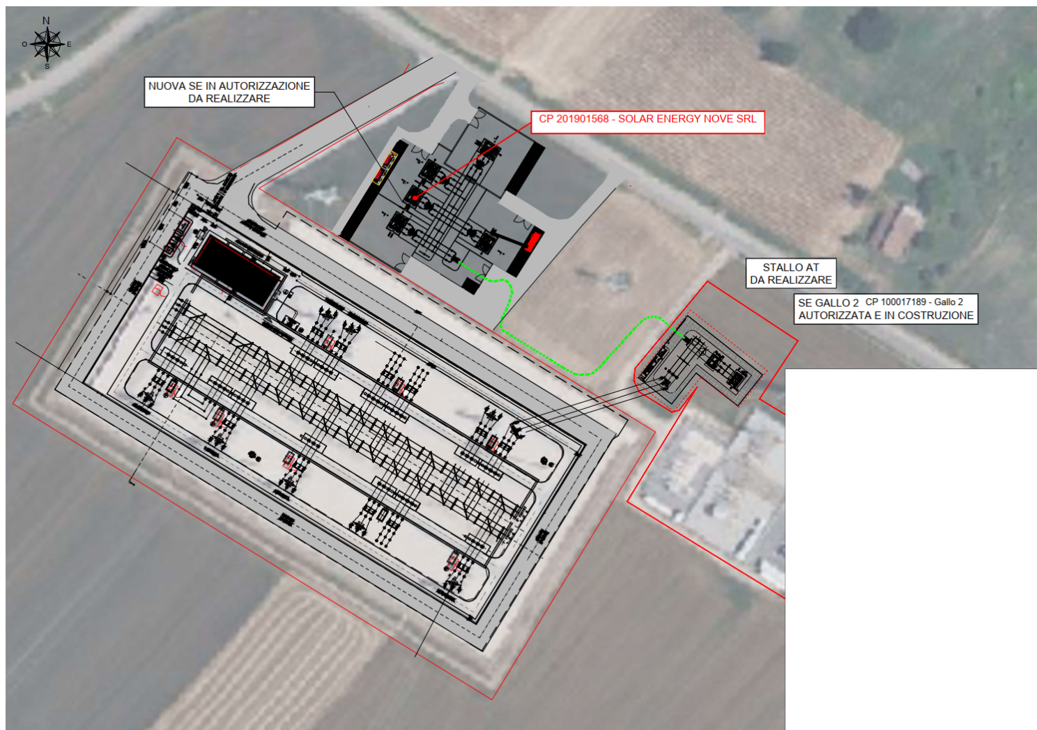
Figura 1 - Inquadramento su ortofoto delle opere di connessione alla RTN
