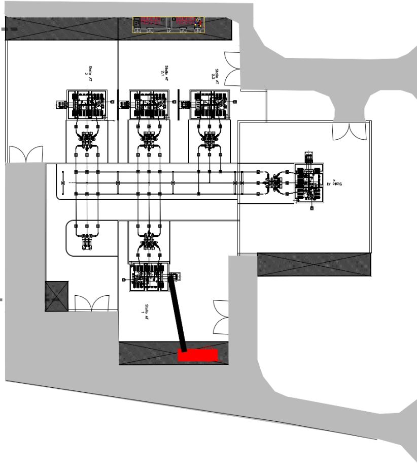
Figura 2 - Layout della sottostazione condivisa
