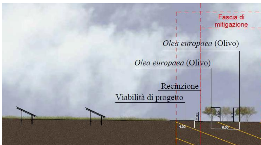
Figura 2: Sezione della fascia di mitigazione perimetrale.
