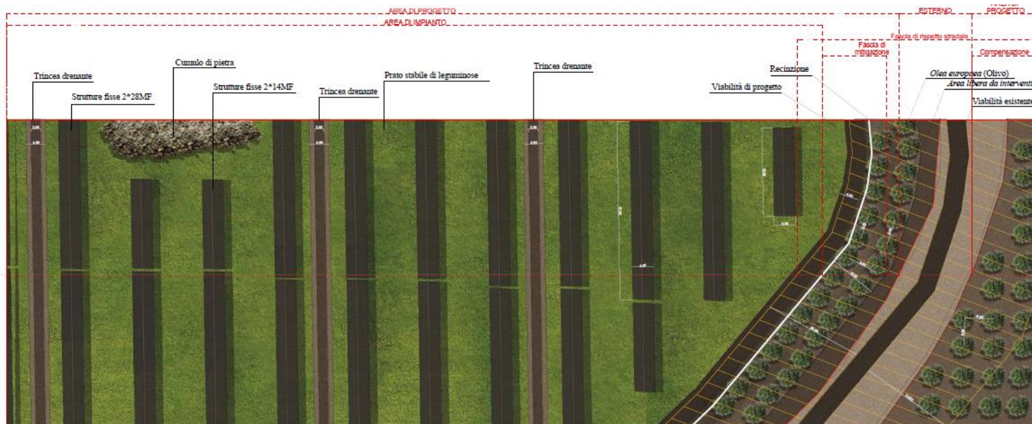
Figura 3: planimetria delle aree di impianto.
