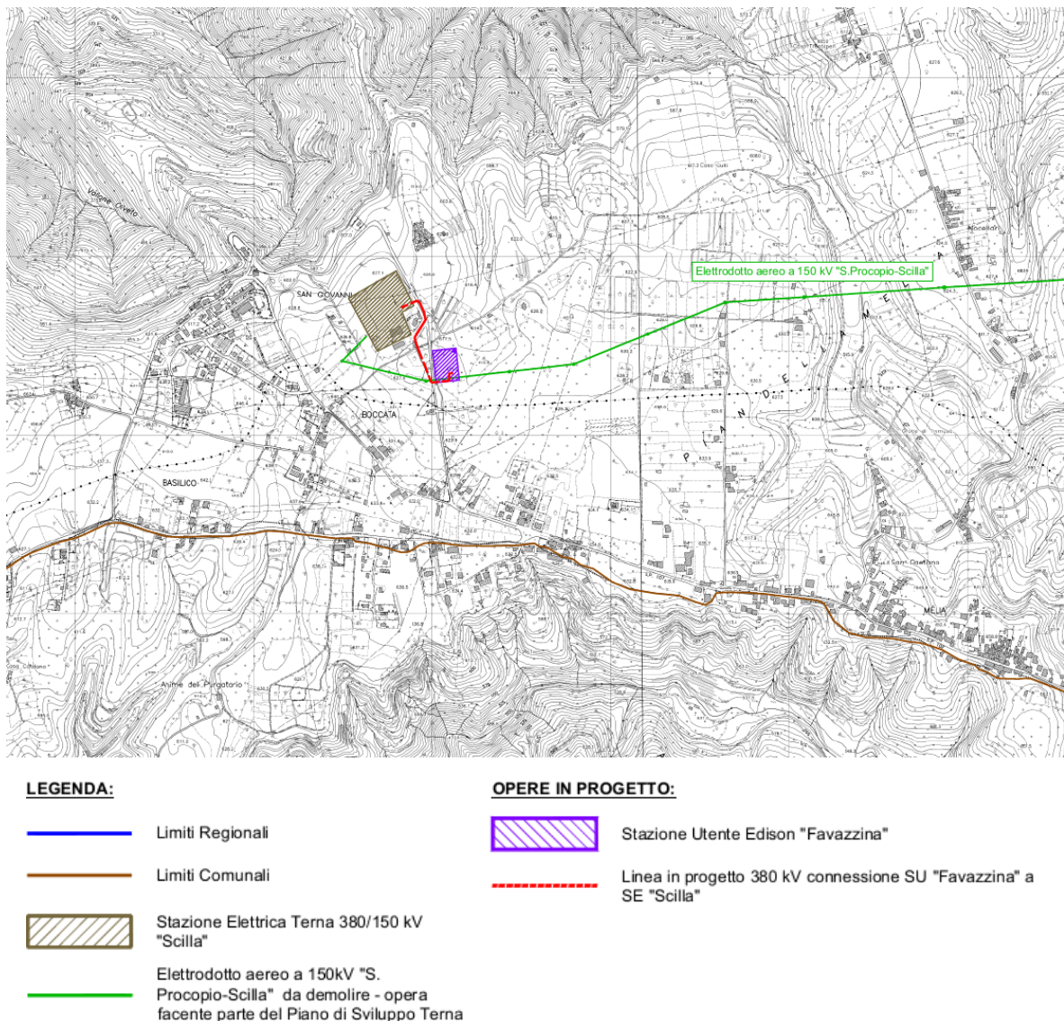
Figura 2.2: Inquadramento su CTR delle opere di connessione alla RTN
