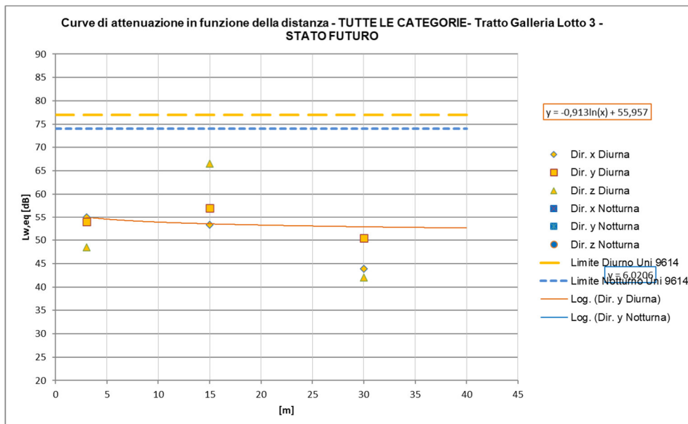
Figura 27 – Curve di attenuazione in funzione della distanza relativa al traffico ferroviario di progetto – tratti al coperto, Treni TUTTE LE CATEGORIE
