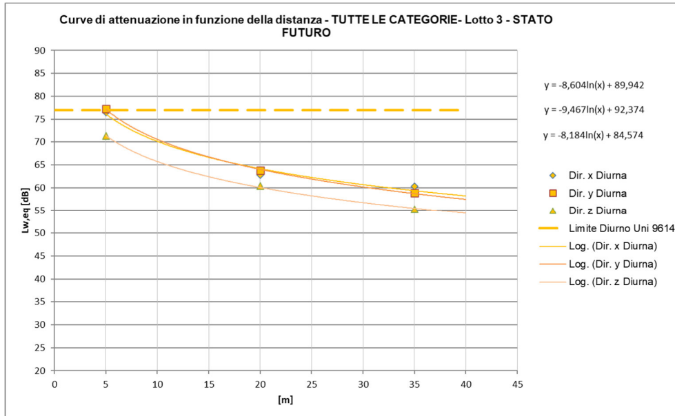
Figura 66 – Curve di attenuazione in funzione della distanza relativa al traffico ferroviario di progetto – tratti allo scoperto INTERNO AGLI EDIFICI, Treni TUTTE LE CATEGORIE, periodo diurno
