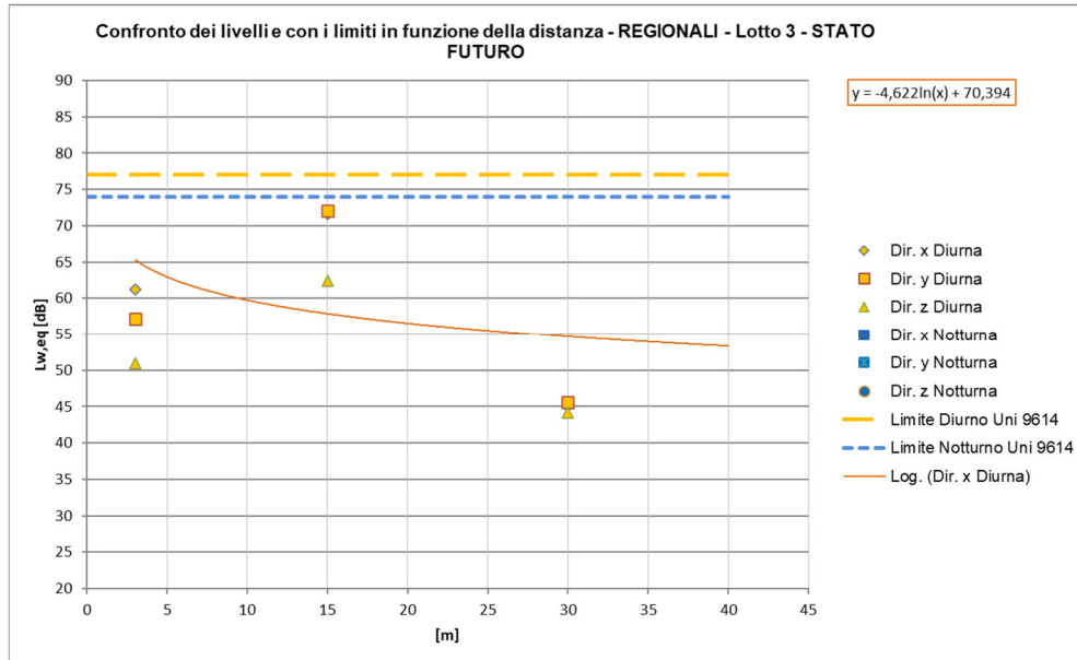
Figura 36 – Curve di attenuazione in funzione della distanza relativa al traffico ferroviario di progetto – tratti allo scoperto, TRENI REGIONALI a 140km/h
