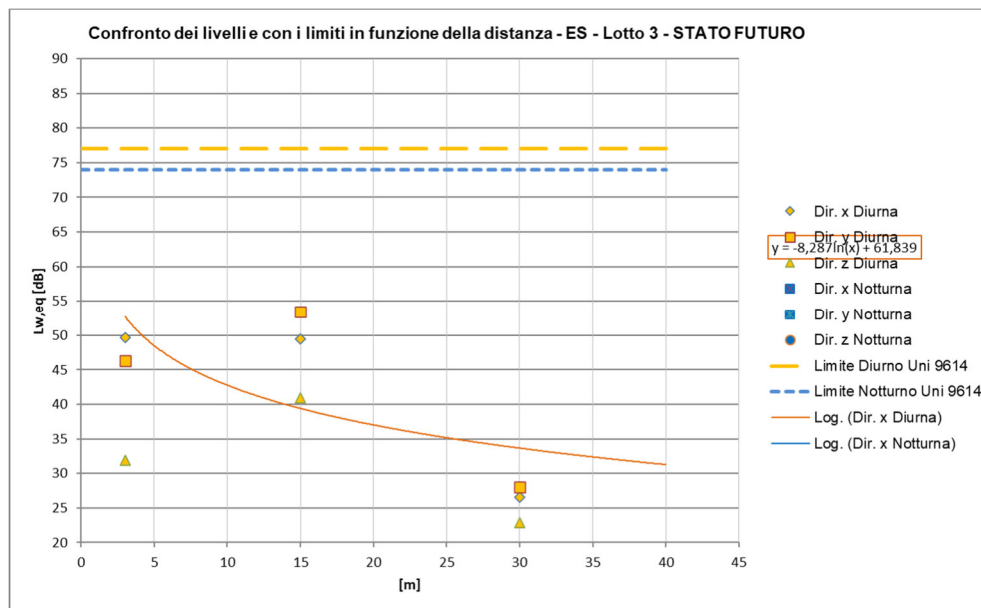
Figura 54 – Curve di attenuazione in funzione della distanza relativa al traffico ferroviario di progetto – tratti allo scoperto, TRENI ES a 105 km/h
