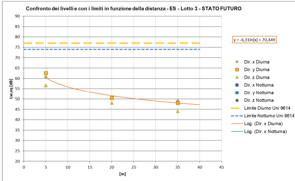
Figura 60 – Curve di attenuazione in funzione della distanza relativa al traffico ferroviario di progetto – tratti allo scoperto, TRENI ES a 140 km/h
