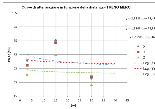
Figura 14 - Curva di attenuazione del Lw,eq in funzione della distanza dal binario, ricavata dai rilievi sperimentali sull'attuale linea in esercizio lungo gli assi x, y e z, in corrispondenza delle SEZ. 2 e valutata considerando le velocità di progetto – TIPOLOGIA TRENO MERCI per t. scoperto/viadotto a 100 km/h
