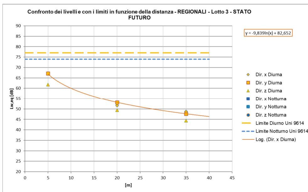
Figura 48 – Curve di attenuazione in funzione della distanza relativa al traffico ferroviario di progetto – tratti allo scoperto, TRENI REGIONALI a 100 km/h
