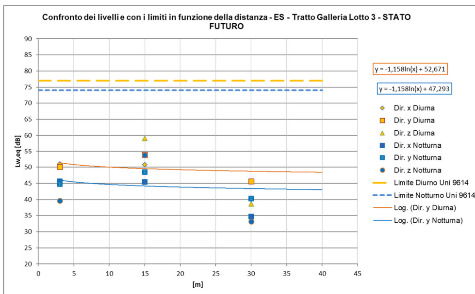
Figura 30 – Curve di attenuazione in funzione della distanza relativa al traffico ferroviario di progetto – tratti al coperto, TRENI ES a 100km/h
