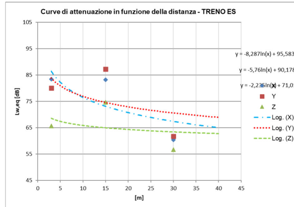
Figura 13 - Curva di attenuazione del Lw,eq in funzione della distanza dal binario, ricavata dai rilievi sperimentali sull'attuale linea in esercizio lungo gli assi x, y e z, in corrispondenza delle SEZ. 2 e valutata considerando le velocità di progetto – TIPOLOGIA TRENO ES per t. scoperto/viadotto a 105 km/h
