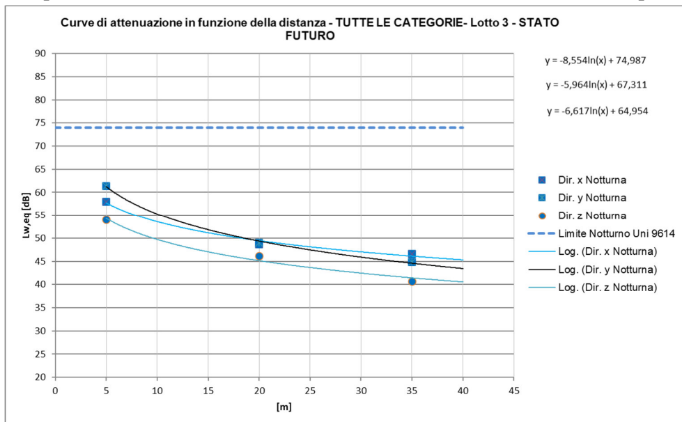
Figura 67 – Curve di attenuazione in funzione della distanza relativa al traffico ferroviario di progetto – tratti allo scoperto INTERNO AGLI EDIFICI, Treni TUTTE LE CATEGORIE, periodo notturno
