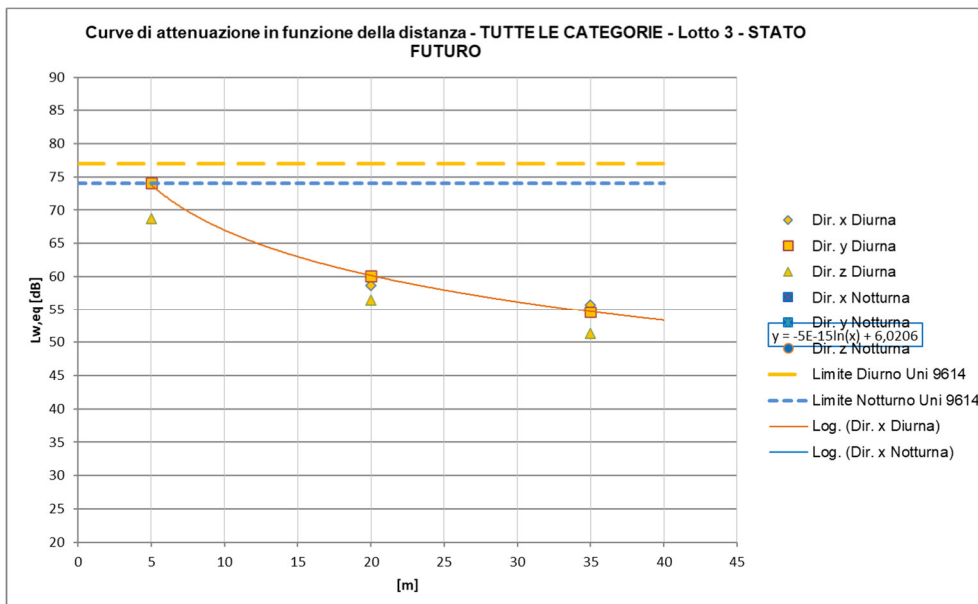
Figura 40 – Curve di attenuazione in funzione della distanza relativa al traffico ferroviario di progetto – tratti allo scoperto, Treni TUTTE LE CATEGORIE
