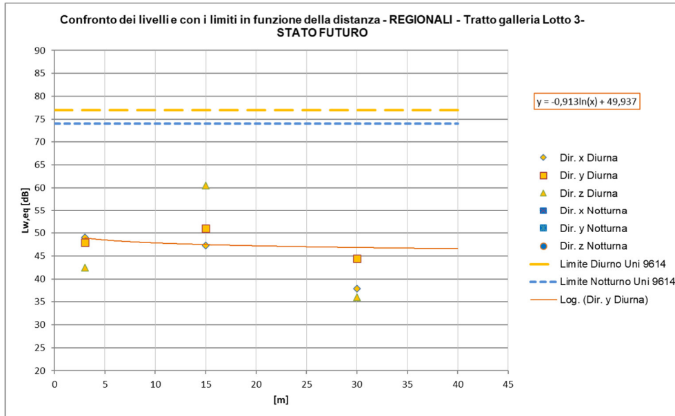
Figura 29 – Curve di attenuazione in funzione della distanza relativa al traffico ferroviario di progetto – tratti al coperto, TRENI REGIONALI a 100km/h
