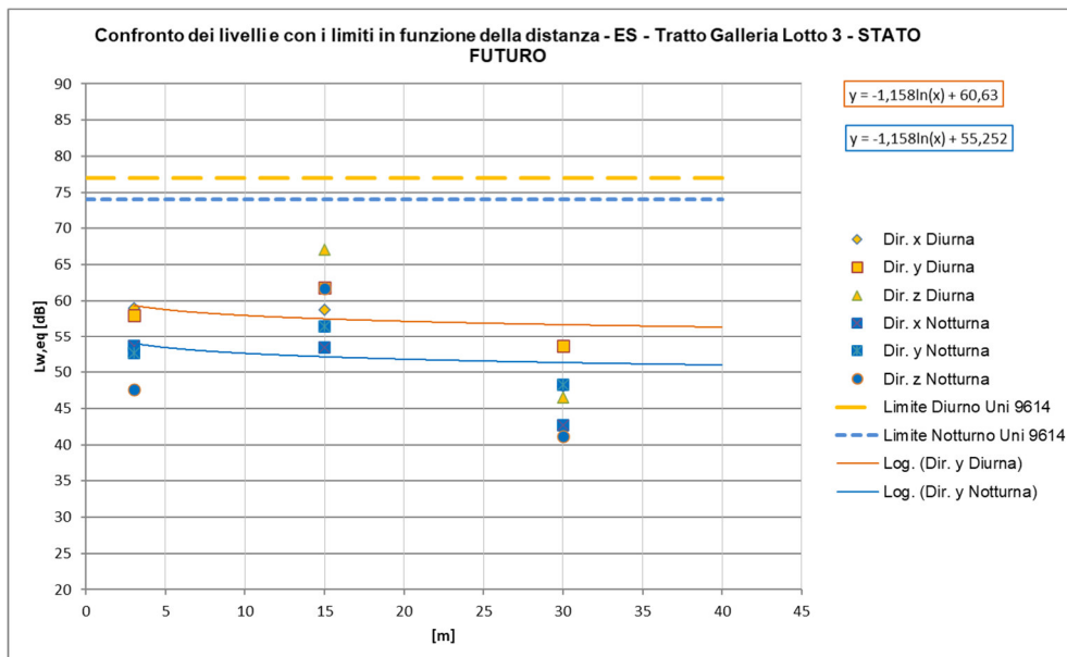
Figura 21 – Curve di attenuazione in funzione della distanza relativa al traffico ferroviario di progetto – tratti al coperto, TRENI ES a 250km/h
