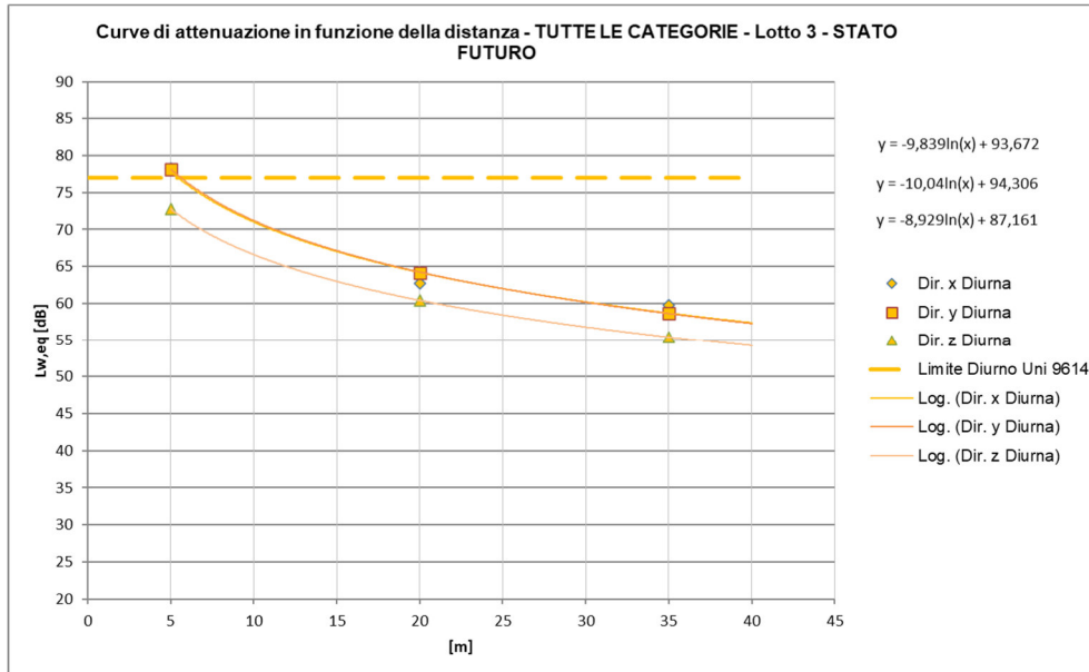
Figura 47 – Curve di attenuazione in funzione della distanza relativa al traffico ferroviario di progetto – tratti allo scoperto INTERNO AGLI EDIFICI, Treni TUTTE LE CATEGORIE, periodo diurno
