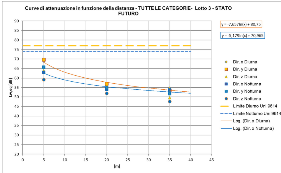
Figura 51 – Curve di attenuazione in funzione della distanza relativa al traffico ferroviario di progetto – tratti allo scoperto, Treni TUTTE LE CATEGORIE
