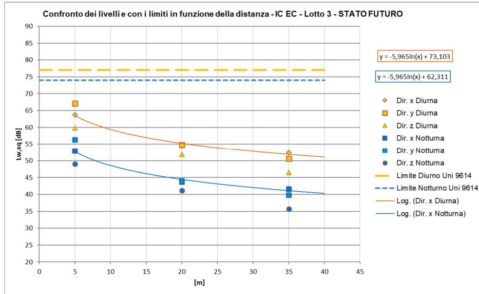
Figura 64 – Curve di attenuazione in funzione della distanza relativa al traffico ferroviario di progetto – tratti allo scoperto, TRENI IC a 105 km/h
