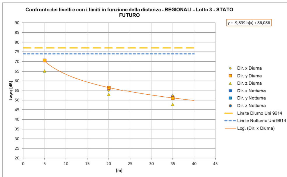
Figura 63 – Curve di attenuazione in funzione della distanza relativa al traffico ferroviario di progetto – tratti allo scoperto, TRENI REGIONALI a 105 km/h
