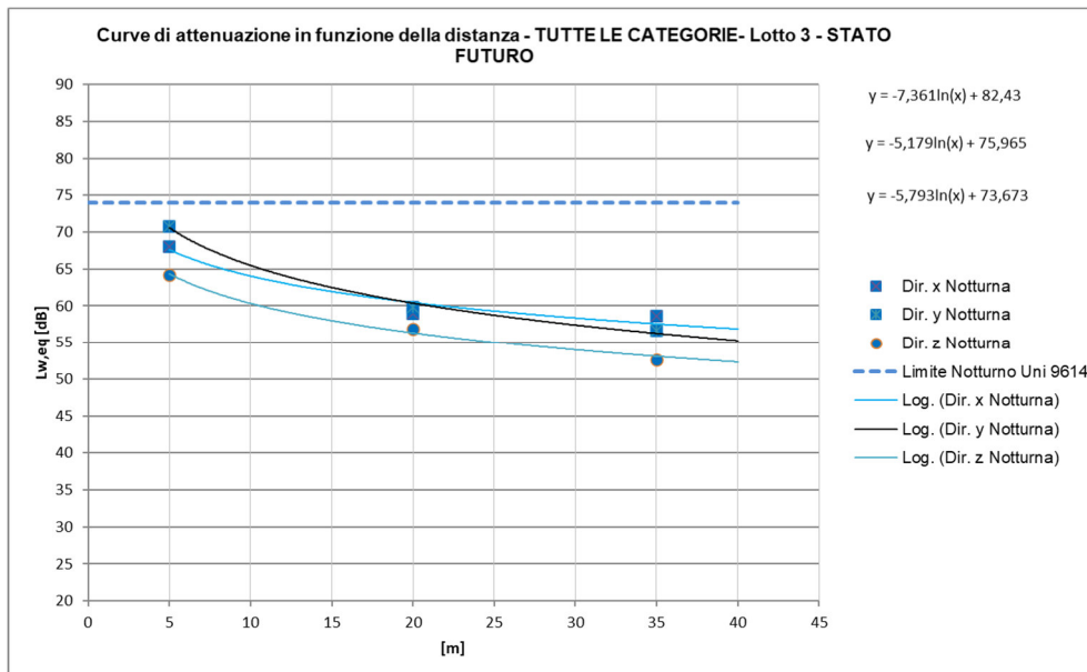
Figura 53 – Curve di attenuazione in funzione della distanza relativa al traffico ferroviario di progetto – tratti allo scoperto INTERNO AGLI EDIFICI, Treni TUTTE LE CATEGORIE, periodo notturno
