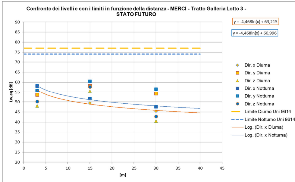
Figura 22 – Curve di attenuazione in funzione della distanza relativa al traffico ferroviario di progetto – tratti al coperto, TRENI MERCI a 100km/h
