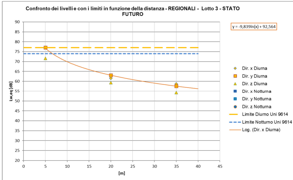
Figura 42 – Curve di attenuazione in funzione della distanza relativa al traffico ferroviario di progetto – tratti allo scoperto, TRENI REGIONALI a 140 km/h
