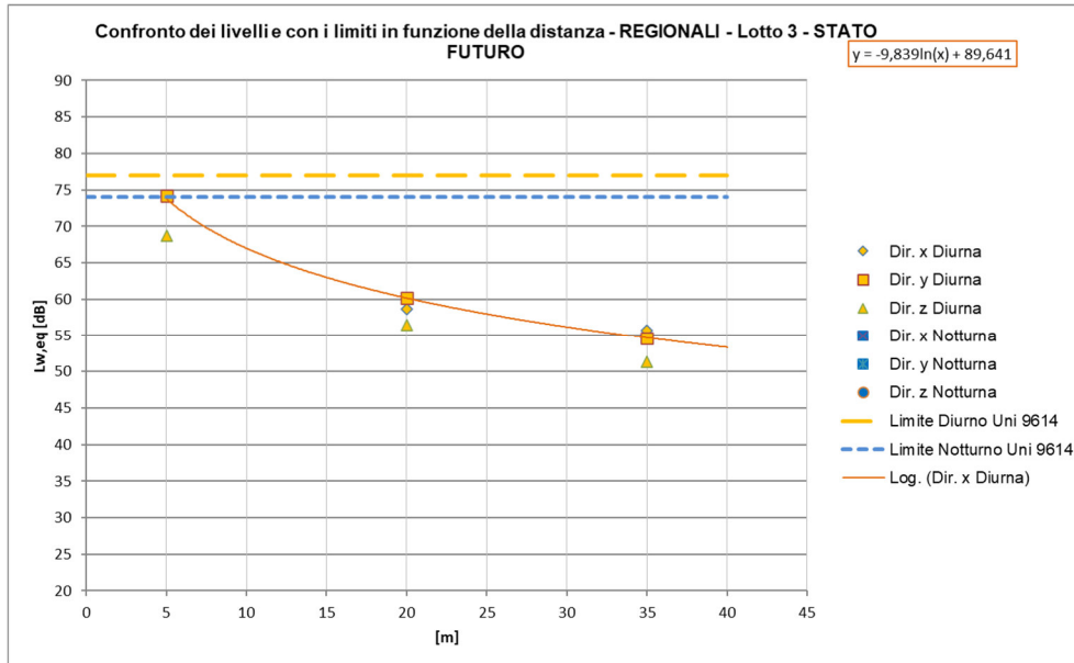
Figura 39 – Curve di attenuazione in funzione della distanza relativa al traffico ferroviario di progetto – tratti allo scoperto, TRENI REGIONALI a 100 km/h
