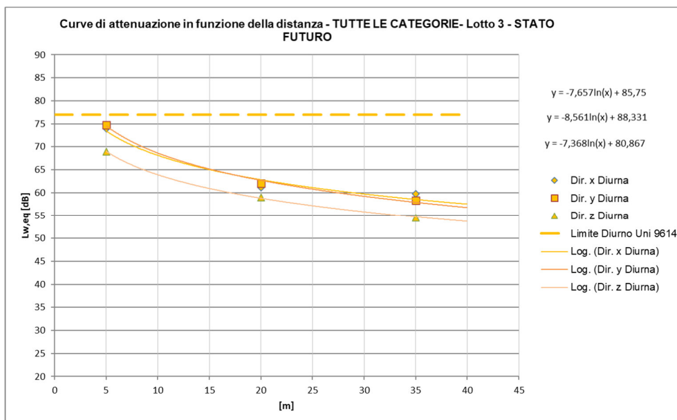
Figura 52 – Curve di attenuazione in funzione della distanza relativa al traffico ferroviario di progetto – tratti allo scoperto INTERNO AGLI EDIFICI, Treni TUTTE LE CATEGORIE, periodo diurno
