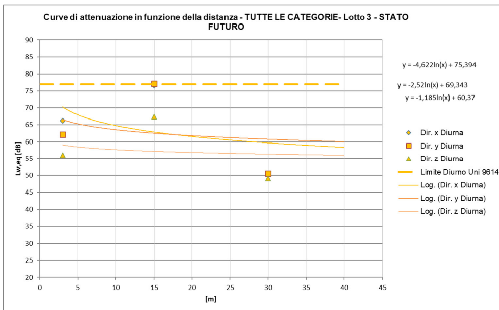
Figura 38 – Curve di attenuazione in funzione della distanza relativa al traffico ferroviario di progetto – tratti allo scoperto INTERNO AGLI EDIFICI, Treni TUTTE LE CATEGORIE, periodo diurno
