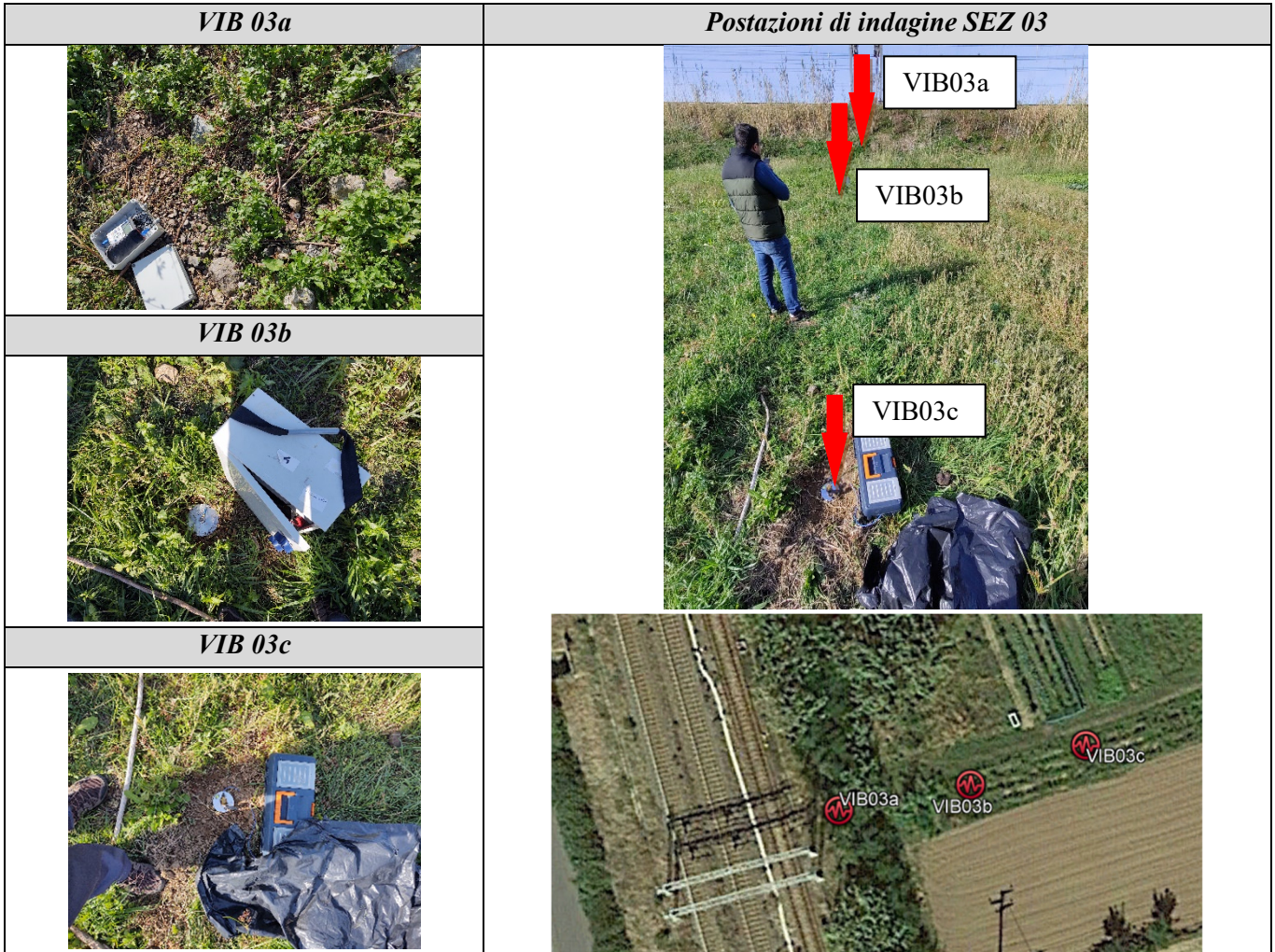
Figura 8 - Report fotografico postazioni di misura (Asse x: parallelo alla linea; Asse Y: ortogonale alla linea; Asse Z verticale)
