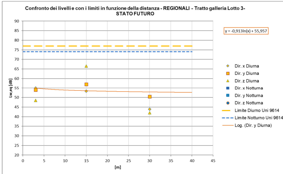
Figura 26 – Curve di attenuazione in funzione della distanza relativa al traffico ferroviario di progetto – tratti al coperto, TRENI REGIONALI a 100km/h
