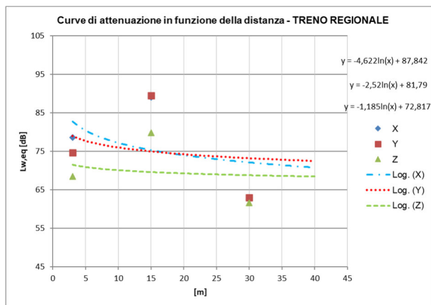
Figura 12 - Curva di attenuazione del Lw,eq in funzione della distanza dal binario, ricavata dai rilievi sperimentali sull'attuale linea in esercizio lungo gli assi x, y e z, in corrispondenza delle SEZ. 2 e valutata considerando le velocità di progetto – TIPOLOGIA TRENO REGIONALE per t. scoperto/viadotto a 140 km/h
