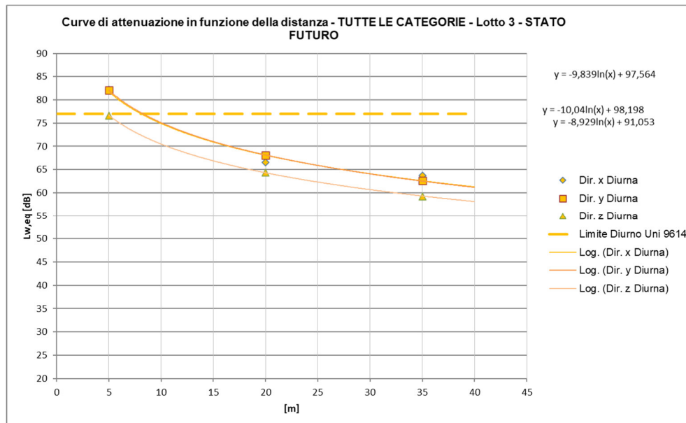
Figura 44 – Curve di attenuazione in funzione della distanza relativa al traffico ferroviario di progetto – tratti allo scoperto INTERNO AGLI EDIFICI, Treni TUTTE LE CATEGORIE, periodo diurno
