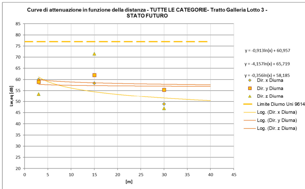
Figura 28 – Curve di attenuazione in funzione della distanza relativa al traffico ferroviario di progetto – tratti al coperto INTERNO AGLI EDIFICI, Treni TUTTE LE CATEGORIE, periodo diurno
