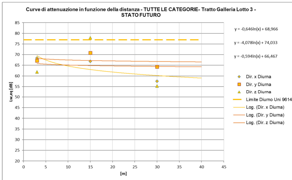
Figura 24 – Curve di attenuazione in funzione della distanza relativa al traffico ferroviario di progetto – tratti al coperto INTERNO AGLI EDIFICI, Treni TUTTE LE CATEGORIE, periodo diurno
