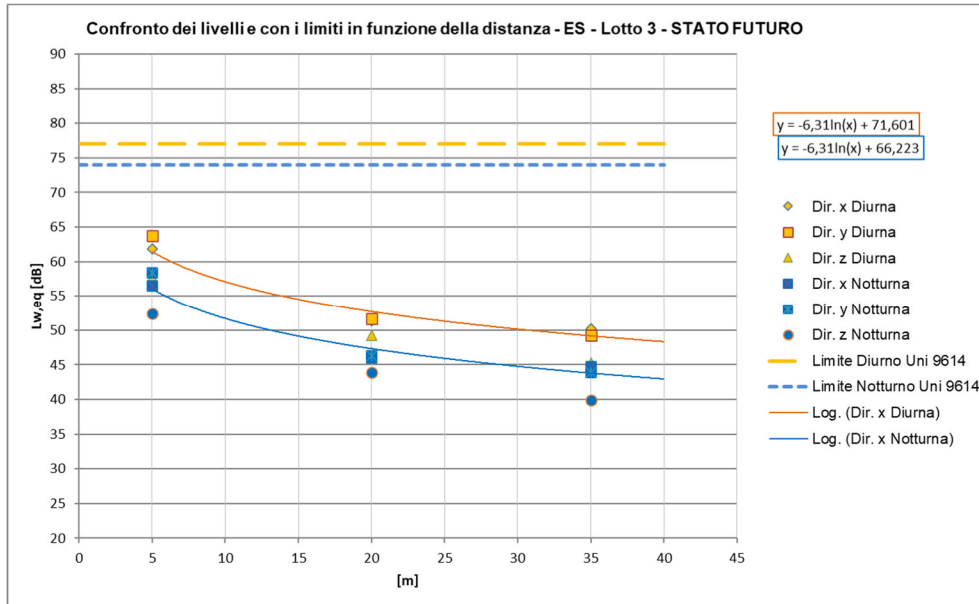
Figura 49 – Curve di attenuazione in funzione della distanza relativa al traffico ferroviario di progetto – tratti allo scoperto, TRENI ES a 100 km/h
