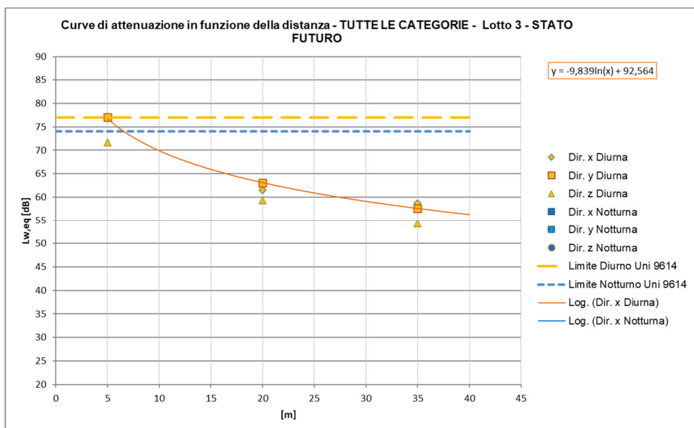
Figura 43 – Curve di attenuazione in funzione della distanza relativa al traffico ferroviario di progetto – tratti allo scoperto, Treni TUTTE LE CATEGORIE
