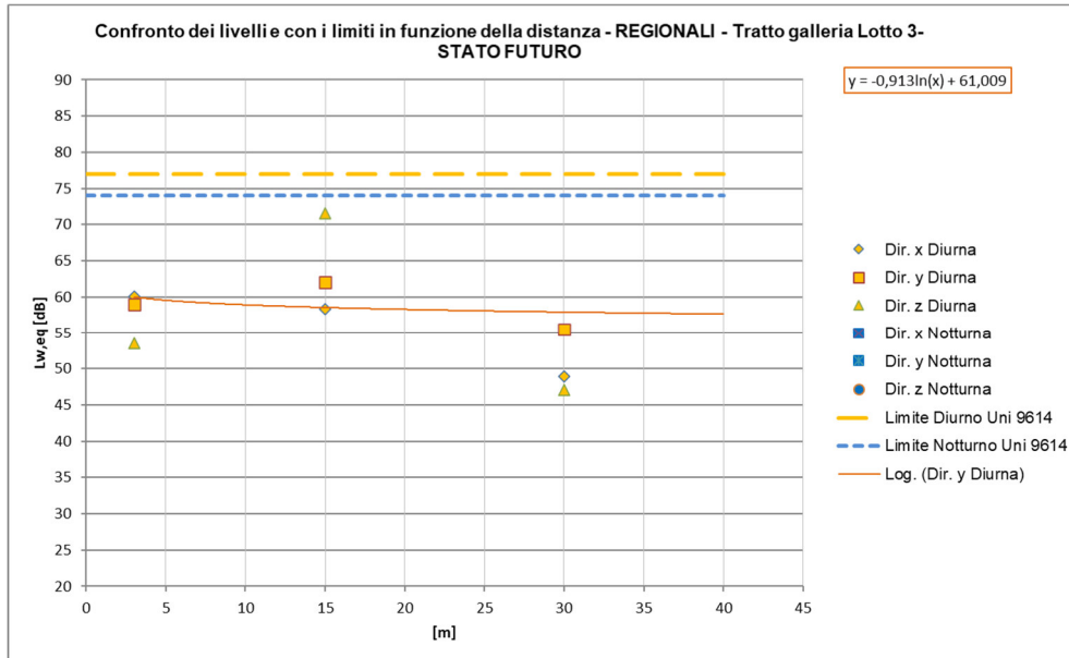
Figura 20 – Curve di attenuazione in funzione della distanza relativa al traffico ferroviario di progetto – tratti al coperto, TRENI REGIONALI a 160km/h
