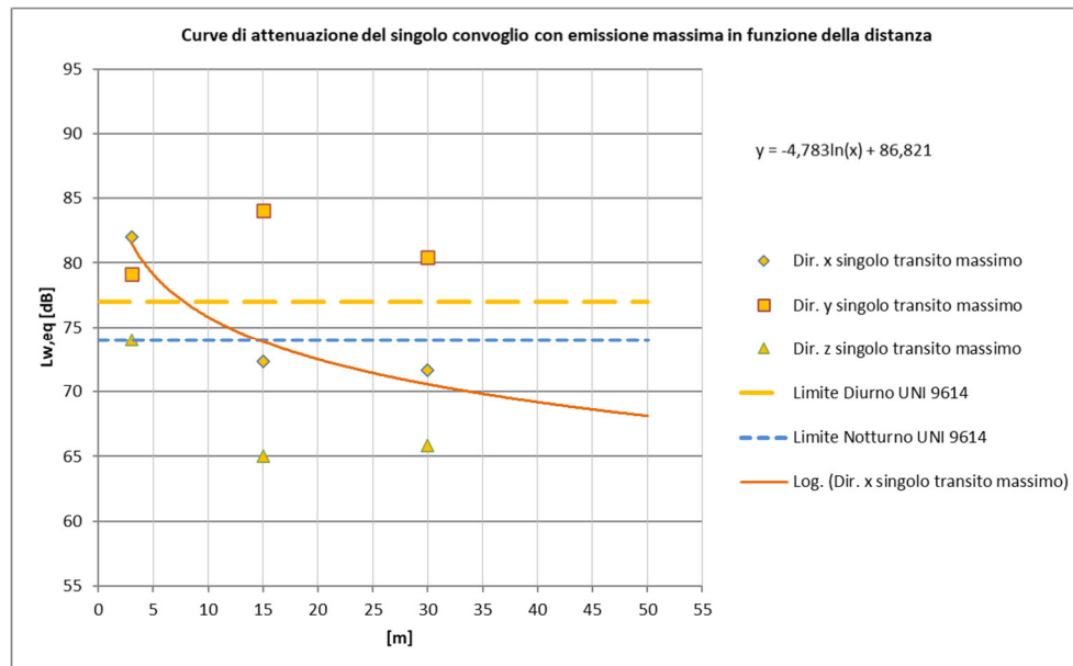
Figura 35 – Curva di attenuazione in funzione della distanza relativa al transito massimo – tratti al coperto
