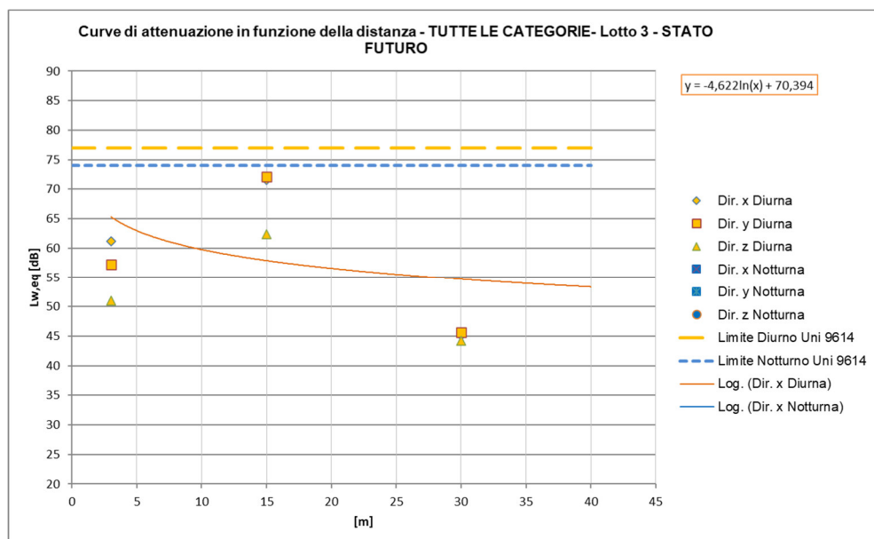
Figura 37 – Curve di attenuazione in funzione della distanza relativa al traffico ferroviario di progetto – tratti allo scoperto, Treni TUTTE LE CATEGORIE
