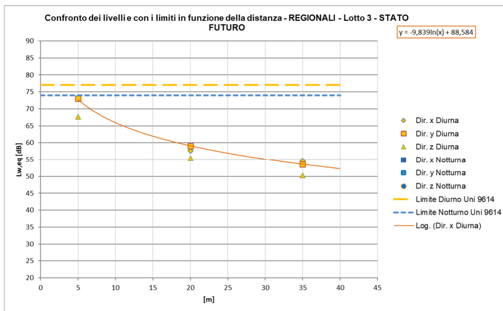
Figura 59 – Curve di attenuazione in funzione della distanza relativa al traffico ferroviario di progetto – tratti allo scoperto, TRENI REGIONALI a 140 km/h
