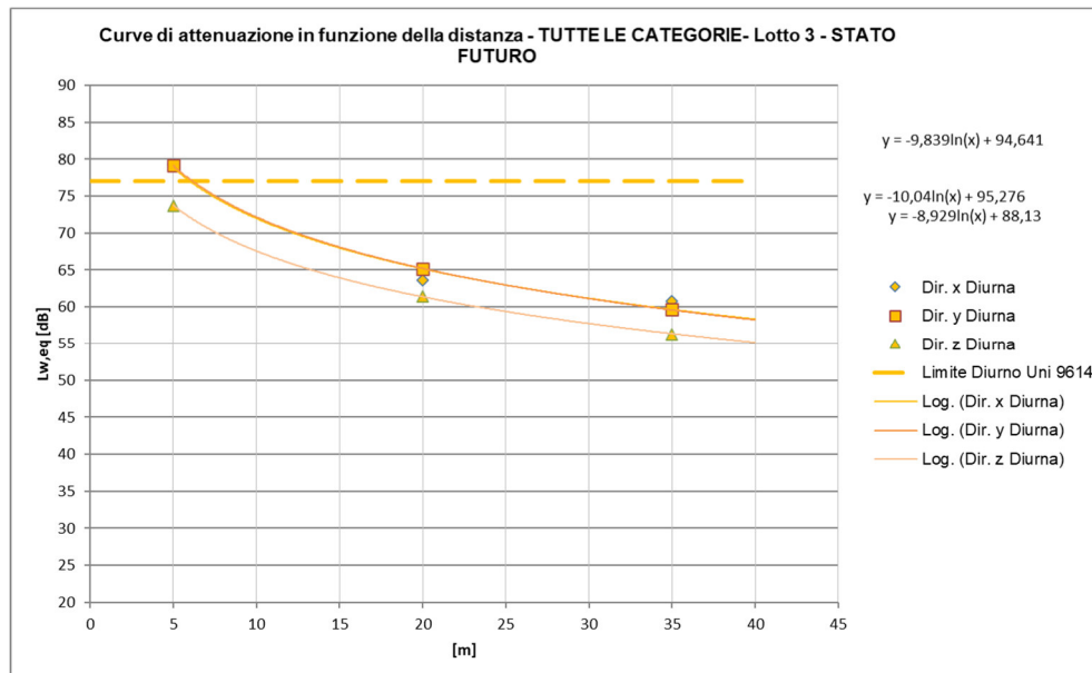
Figura 41 – Curve di attenuazione in funzione della distanza relativa al traffico ferroviario di progetto – tratti allo scoperto INTERNO AGLI EDIFICI, Treni TUTTE LE CATEGORIE, periodo diurno
