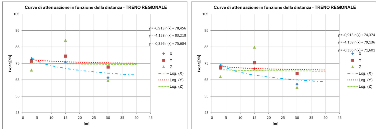
Figura 9 - Curva di attenuazione del L_{w,eq} in funzione della distanza dal binario, ricavata dai rilievi sperimentali sull'attuale linea in esercizio lungo gli assi x, y e z, in corrispondenza delle SEZ. 1 e valutata considerando le velocità di progetto a sinistra a 160 km/h a destra a 100 km/h – TIPOLOGIA TRENO REGIONALE per t. coperto
