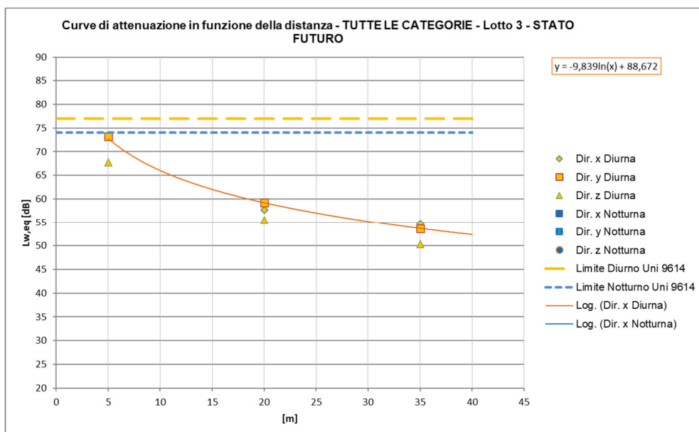
Figura 46 – Curve di attenuazione in funzione della distanza relativa al traffico ferroviario di progetto – tratti allo scoperto, Treni TUTTE LE CATEGORIE
