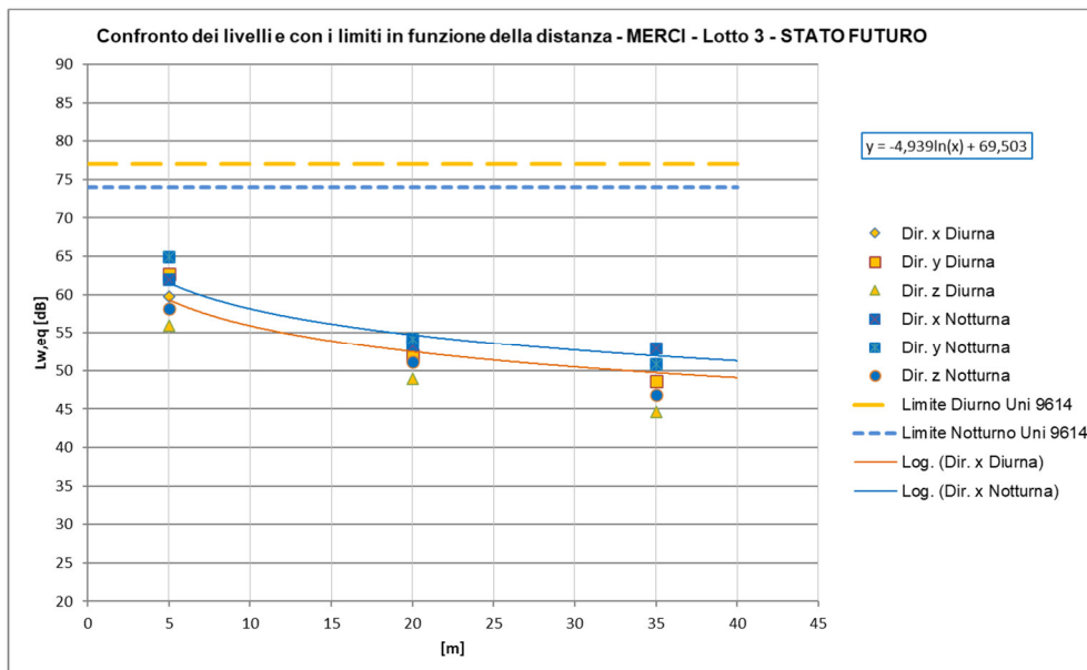
Figura 50 – Curve di attenuazione in funzione della distanza relativa al traffico ferroviario di progetto – tratti allo scoperto, TRENI MERCI a 100 km/h
