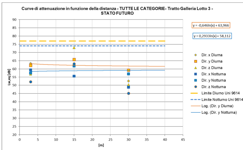
Figura 23 – Curve di attenuazione in funzione della distanza relativa al traffico ferroviario di progetto – tratti al coperto, Treni TUTTE LE CATEGORIE
