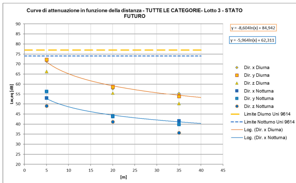
Figura 65 – Curve di attenuazione in funzione della distanza relativa al traffico ferroviario di progetto – tratti allo scoperto, Treni TUTTE LE CATEGORIE
