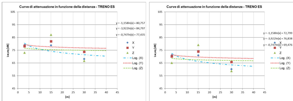
Figura 10 - Curva di attenuazione del L_{w,eq} in funzione della distanza dal binario, ricavata dai rilievi sperimentali sull'attuale linea in esercizio lungo gli assi x, y e z, in corrispondenza delle SEZ. 1 e valutata considerando le velocità di progetto a sinistra a 250 km/h a destra a 100 km/h – TIPOLOGIA TRENO ES per t. coperto
