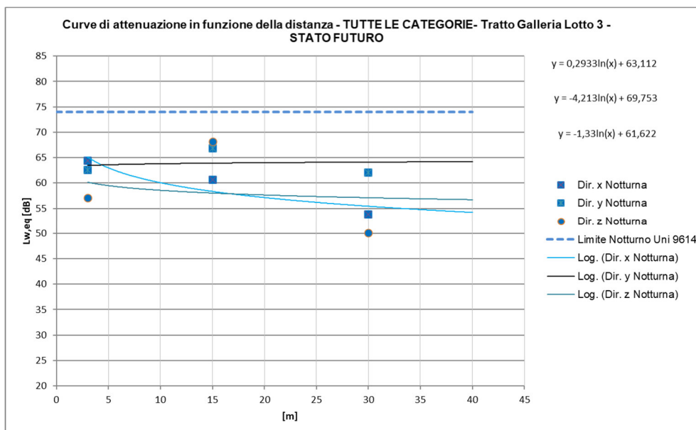
Figura 25 – Curve di attenuazione in funzione della distanza relativa al traffico ferroviario di progetto – tratti al coperto INTERNO AGLI EDIFICI, Treni TUTTE LE CATEGORIE, periodo notturno
