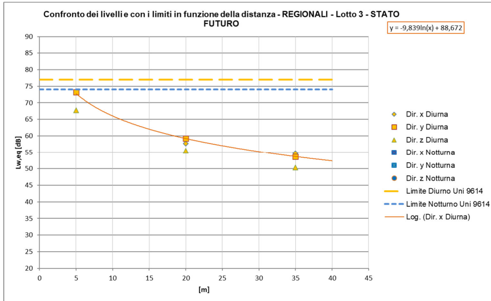
Figura 45 – Curve di attenuazione in funzione della distanza relativa al traffico ferroviario di progetto – tratti allo scoperto, TRENI REGIONALI a 100 km/h
