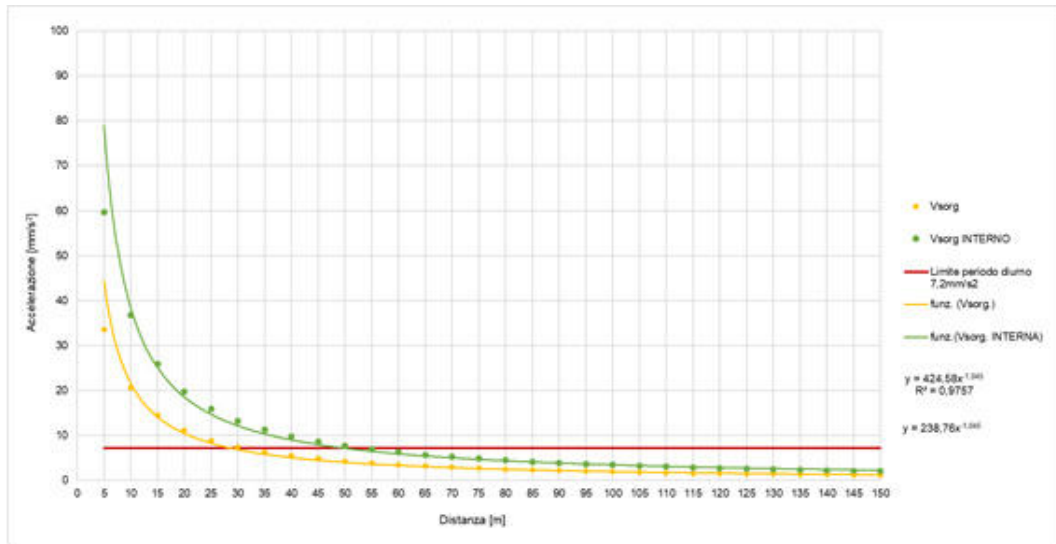
Figura 6-35– Propagazione dei livelli di accelerazione stimati sui ricettori residenziali per il pacchetto “GN (fase di perforazione)”
