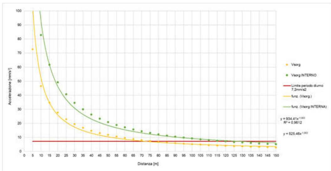
Figura 6-34– Propagazione dei livelli di accelerazione stimati sui ricettori residenziali per il pacchetto “Rilevati (fase di compattazione)”
