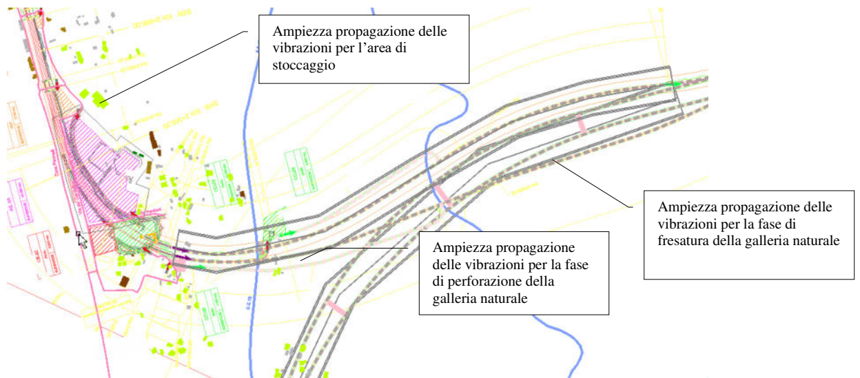
Figura 6-44- stralcio con ampiezza dell'aree di superamento interno agli edifici del limite delle vibrazioni per le aree GN02-GN03-AS.04
