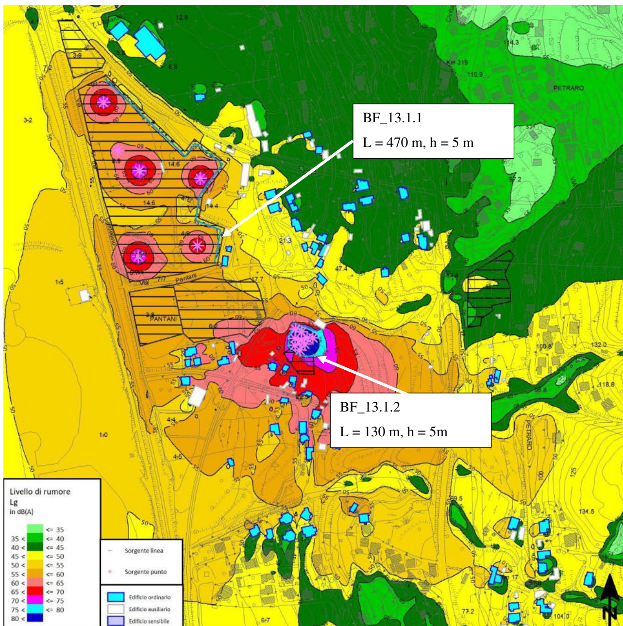
Figura 6-10 – Mappatura acustica, h=4 metri, in presenza di elementi mitigativi
