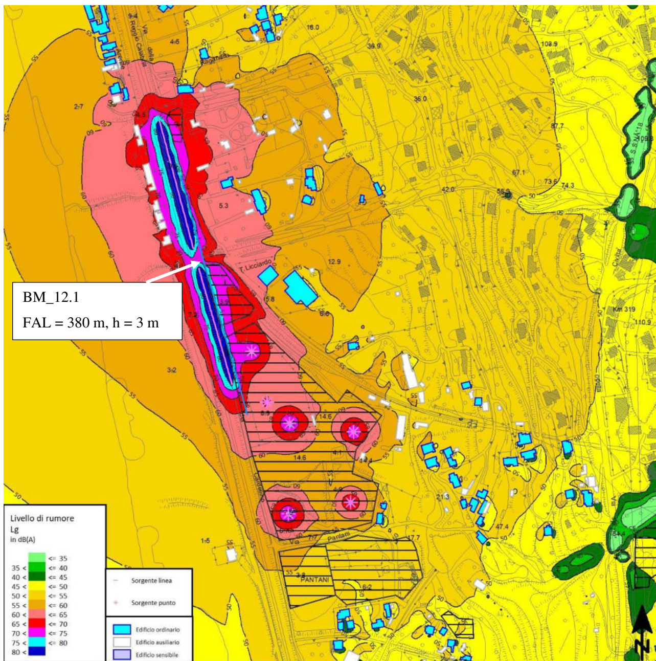
Figura 6-6 – Mappatura acustica, h=4 metri, in presenza di elementi mitigativi
