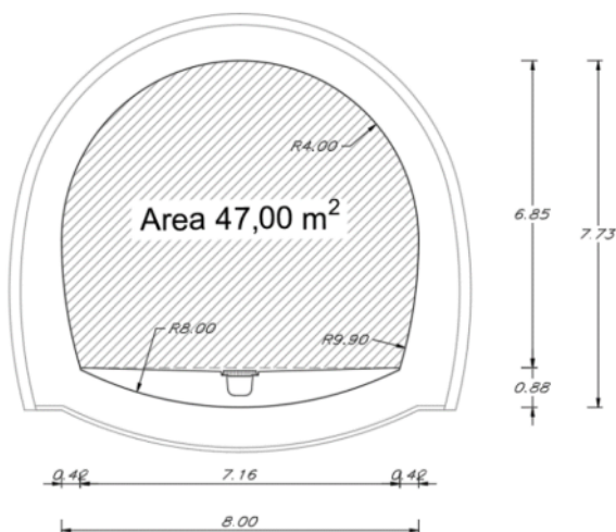
Figura 2-3 Sezione cunicolo disconnessione fumi
