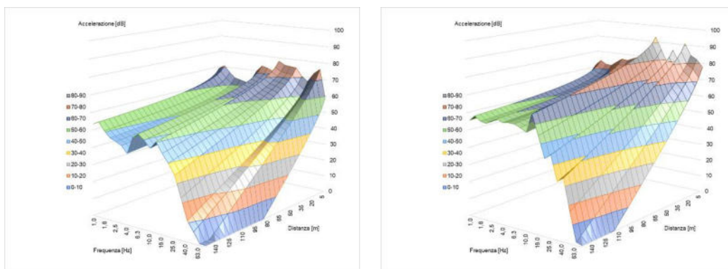
Figura 6-30– Propagazione dei livelli di accelerazione in dB (UNI 9614) per singola frequenza, a sinistra per il pacchetto AT per Nuova Stazione, a destra per il pacchetto AT per Nuova Stazione (fase di compattazione)
