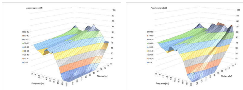
Figura 6-29– Propagazione dei livelli di accelerazione in dB (UNI 9614) per singola frequenza, a sinistra per il pacchetto Cantiere Operativo, a destra per il pacchetto AT per opere FA (Fabbricati)
