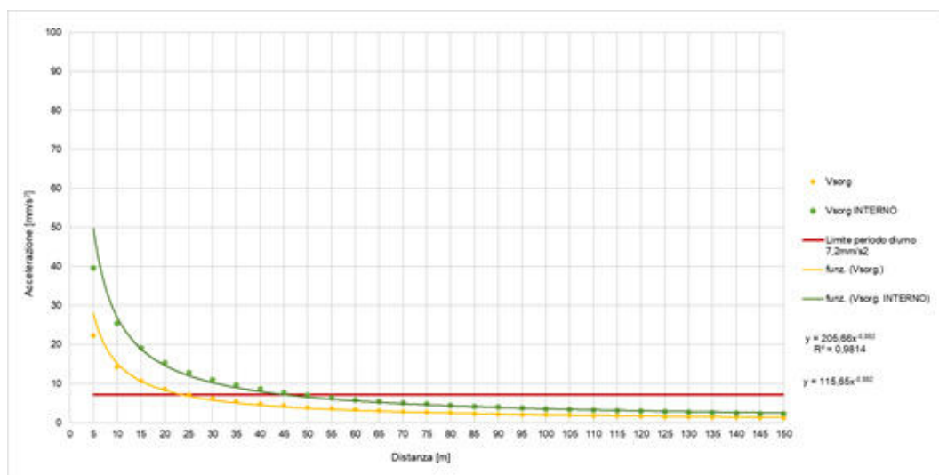
Figura 6-36– Propagazione dei livelli di accelerazione stimati sui ricettori residenziali per il pacchetto “GN (fase di fresatura)”
