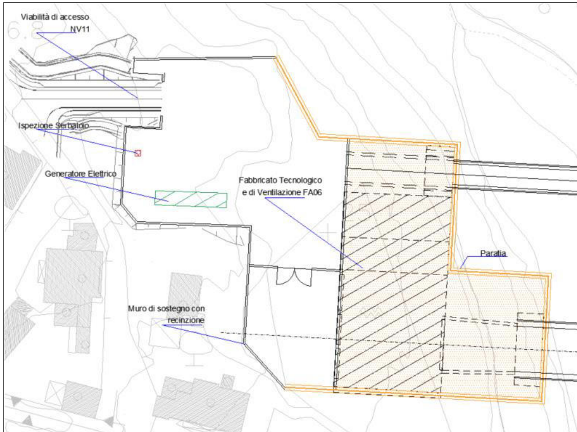
Figura 2-5 Planimetria piazzale disconnessione fumi
