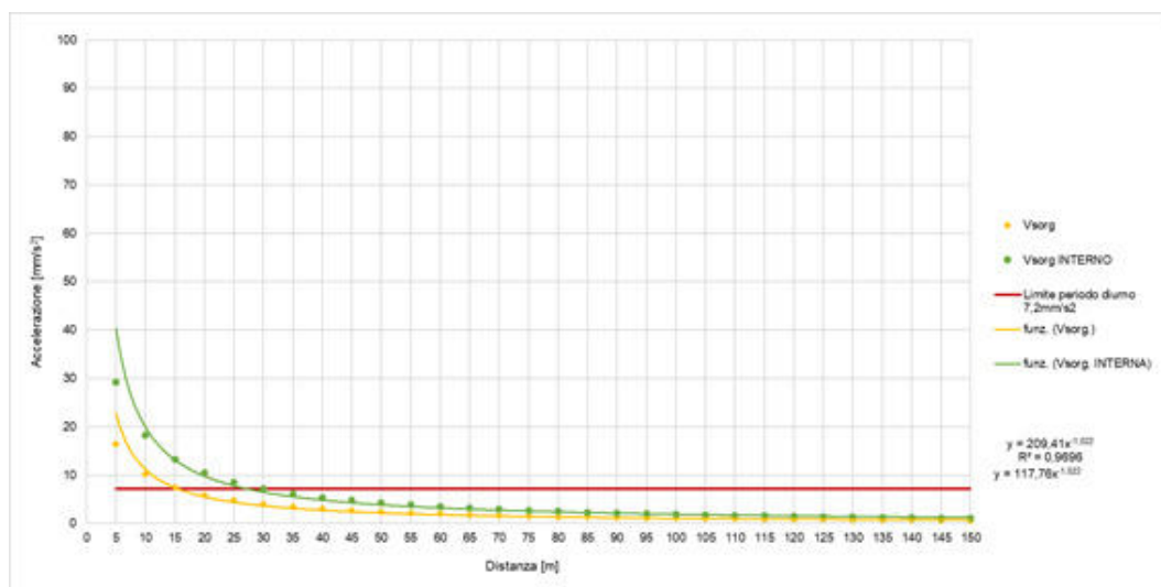
Figura 6-33– Propagazione dei livelli di accelerazione stimati sui ricettori residenziali per il pacchetto "Rilevati"
