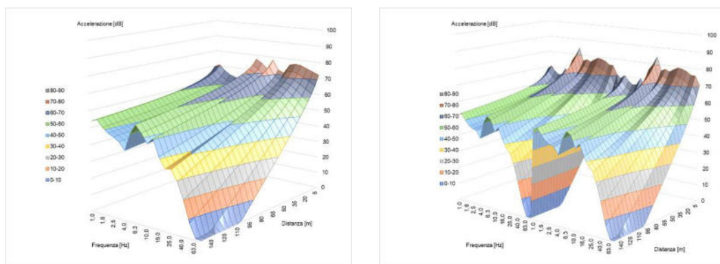
Figura 6-26– Propagazione dei livelli di accelerazione in dB (UNI 9614) per singola frequenza, a sinistra per il pacchetto Realizzazione Galleria Artificiale (fase di palificazione), a destra per il pacchetto Realizzazione Galleria Artificiale (fase di jet grouting)
