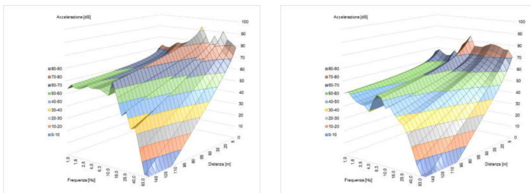
Figura 6-27– Propagazione dei livelli di accelerazione in dB (UNI 9614) per singola frequenza, a sinistra per il pacchetto Realizzazione trincea (fase di compattazione), a destra per il pacchetto Realizzazione trincea (fase di palificazione)
