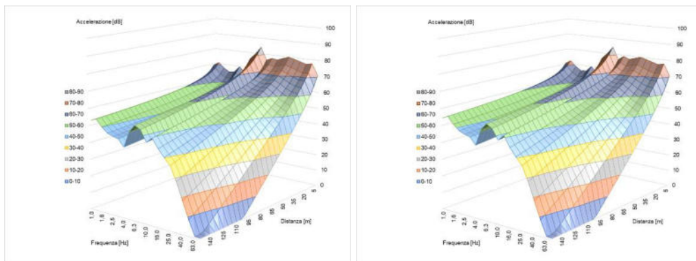
Figura 6-24 Propagazione dei livelli di accelerazione in dB (UNI 9614) per singola frequenza, a sinistra per il pacchetto Viadotto (fase di palificazione), a destra per il pacchetto Viadotto (fase di jet grouting)
