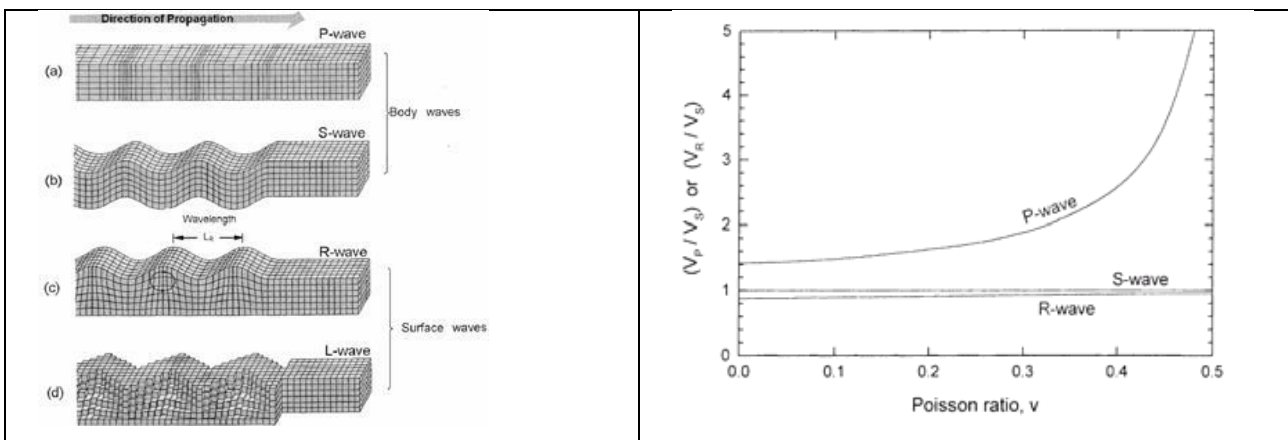
Figura 6-20 Tipi di onda di volume e di superficie (a sinistra) e velocità relativa delle onde P, R rispetto onde S (a destra)
