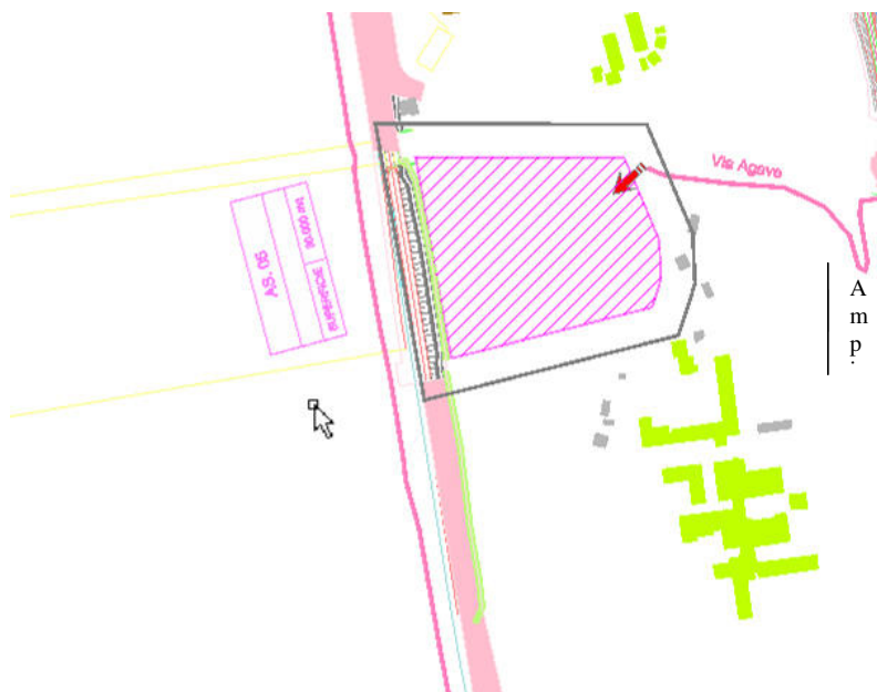
Figura 6-46- stralcio con ampiezza dell'area di superamento interno agli edifici del limite delle vibrazioni per l'area AS.05
