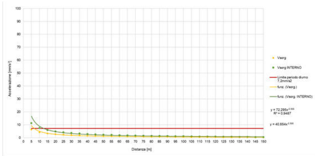
Figura 6-40 – Propagazione dei livelli di accelerazione stimati sui ricettori residenziali per il pacchetto “Cantiere Operativo”
