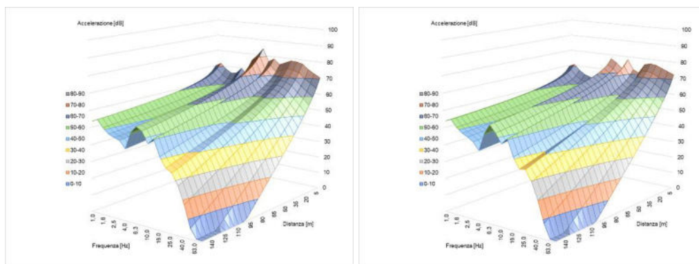
Figura 6-25 Propagazione dei livelli di accelerazione in dB (UNI 9614) per singola frequenza, a sinistra per il pacchetto Realizzazione Galleria Naturale(fase di perforazione), a destra per il pacchetto Realizzazione Galleria Naturale (fase di fresatura)
