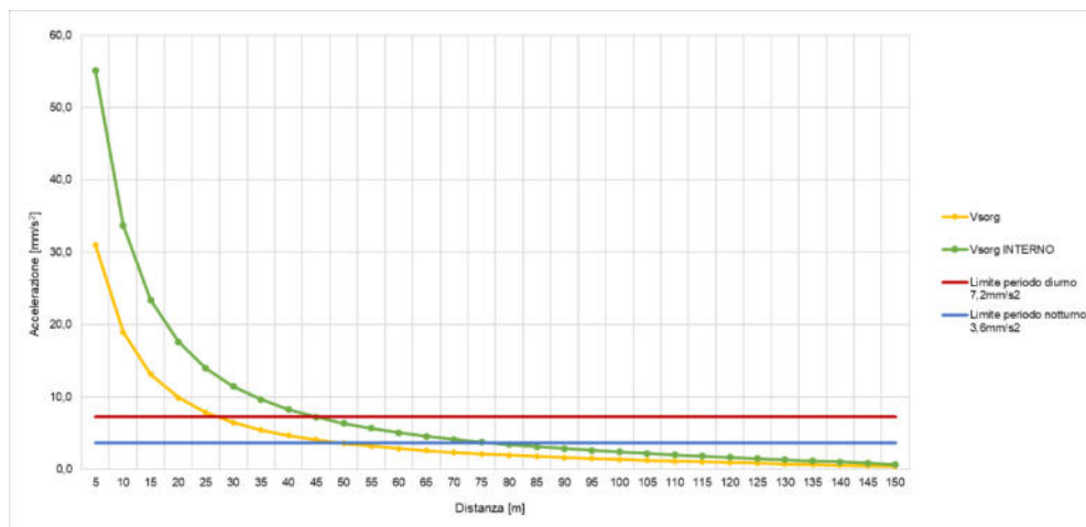
figura 6.19 valutazione della propagazione del livello di vibrazioni (vettore sorgente) a diverse distanze
