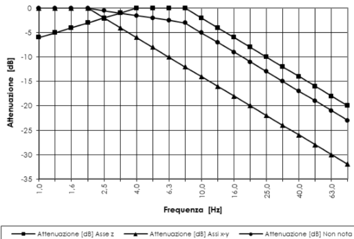
Figura 6-17 Filtri di ponderazione per i diversi assi di riferimento
