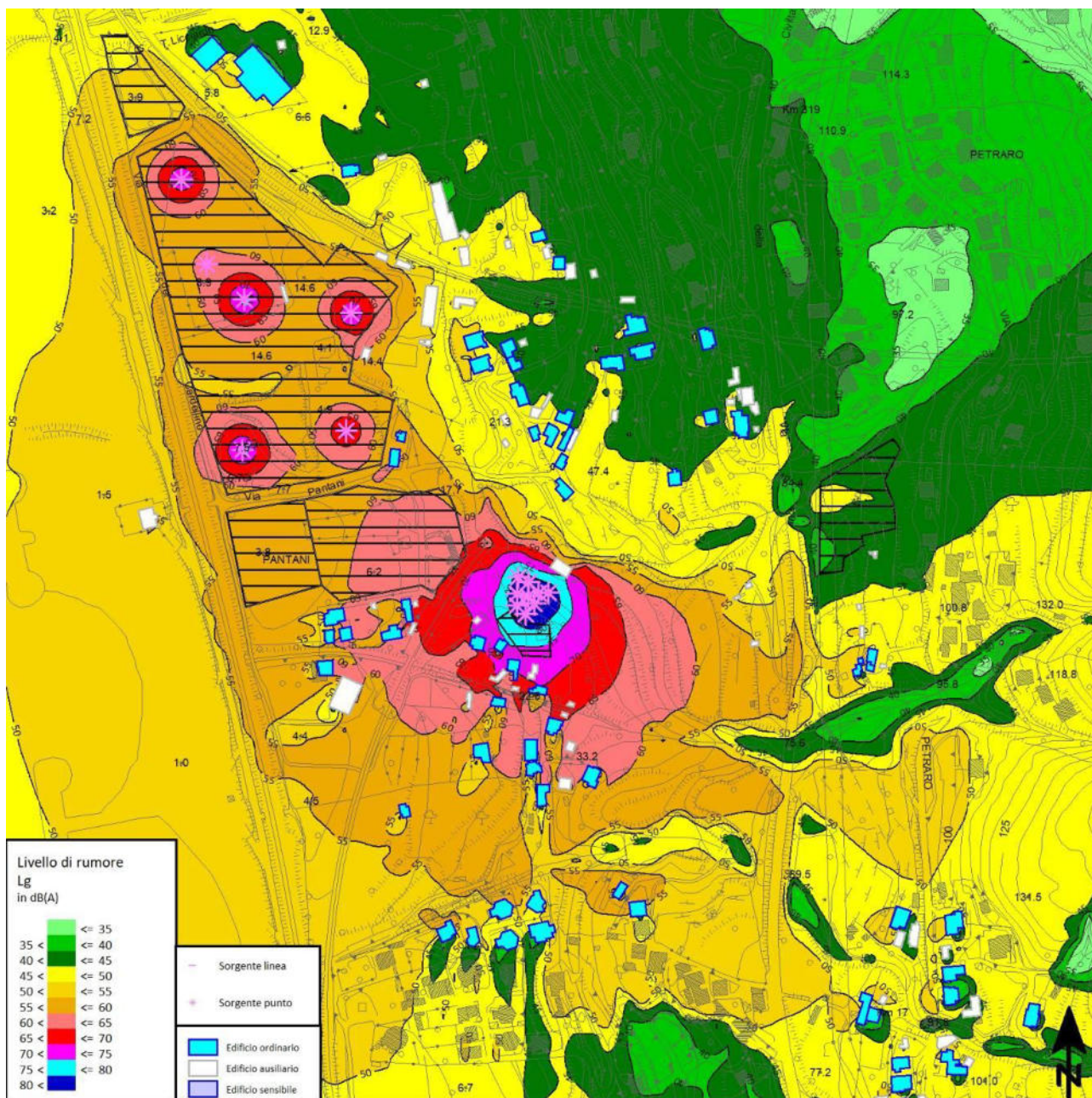
Figura 6-9 – Mappatura acustica, h=4 metri, in assenza di elementi mitigativi
