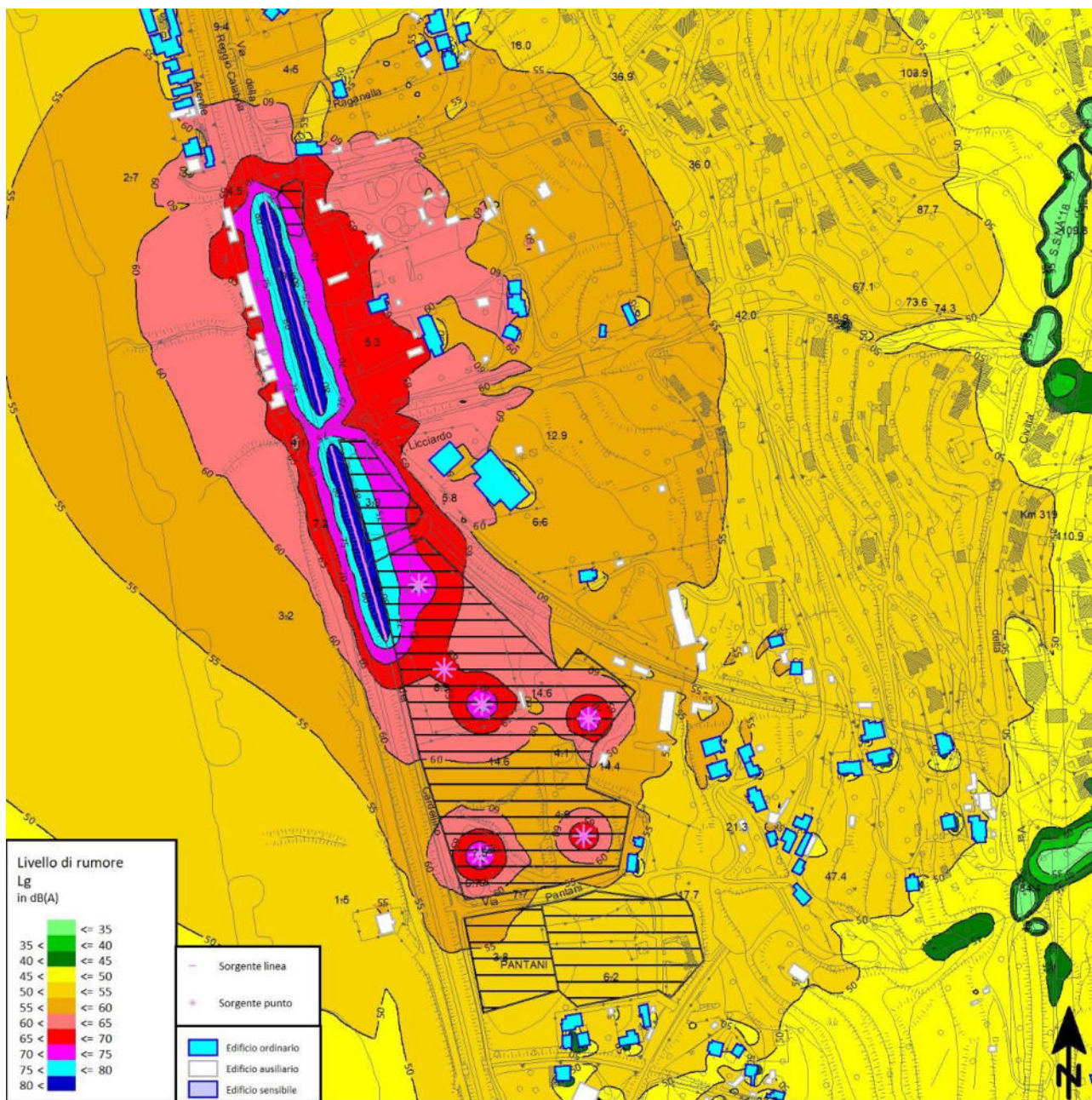
Figura 6-5 – Mappatura acustica, h=4 metri, in assenza di elementi mitigativi
