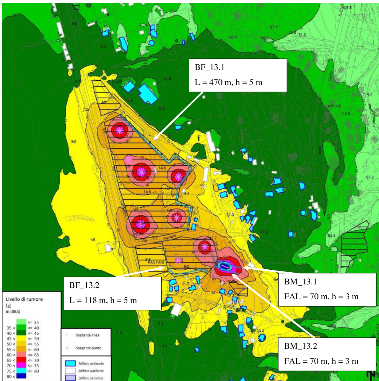
Figura 6-8 – Mappatura acustica, h=4 metri, in presenza di elementi mitigativi
