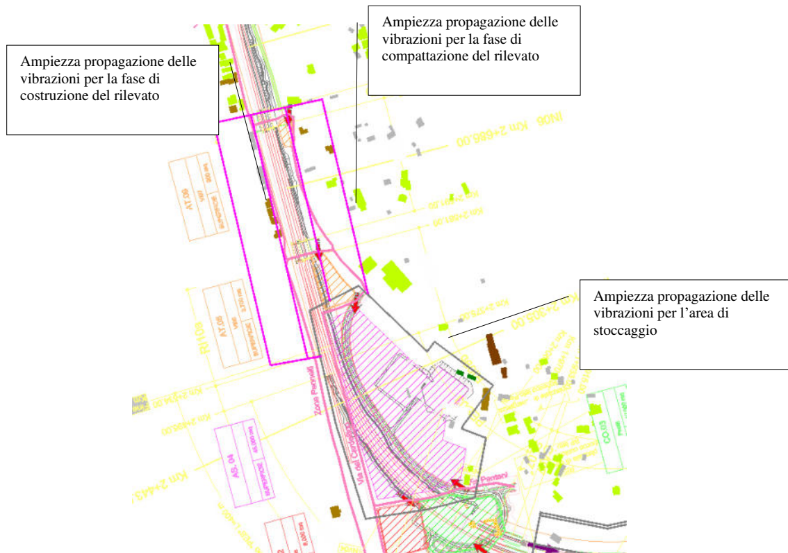
Figura 6-42- stralcio con ampiezza dell'aree di superamento interno agli edifici del limite delle vibrazioni per le aree RI10b-RI11b-AS.04
