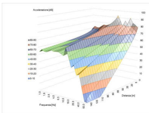
Figura 6-32– Propagazione dei livelli di accelerazione in dB (UNI 9614) per singola frequenza, per il pacchetto Cantiere Nuova Viabilità (fase di compattazione)
