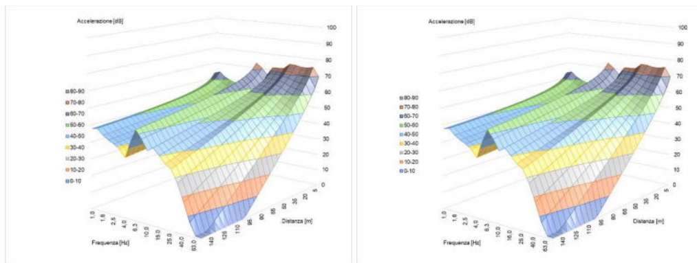
Figura 6-23 Propagazione dei livelli di accelerazione in dB (UNI 9614) per singola frequenza, a sinistra per il pacchetto Rilevati, a destra per il pacchetto Rilevati (fase di compattazione)
