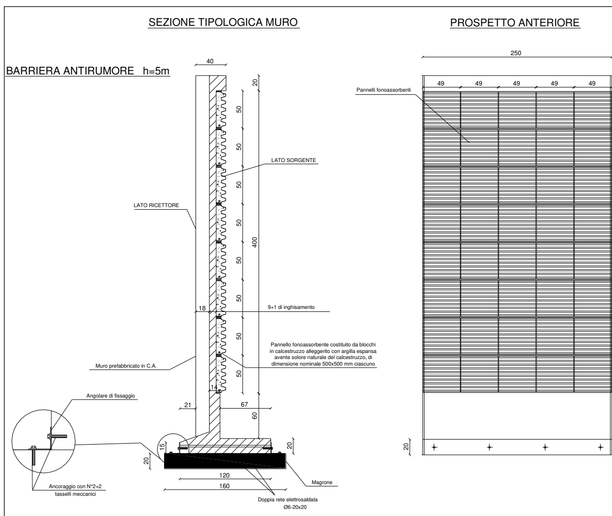
Figura 6-15 Barriere antirumore
