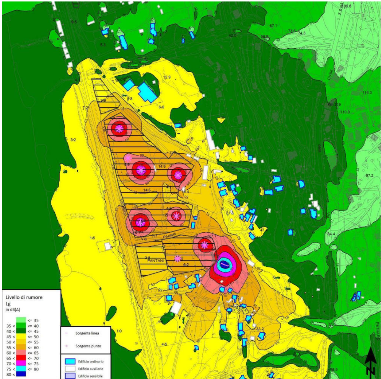
Figura 6-7 – Mappatura acustica, h=4 metri, in assenza di elementi mitigativi
