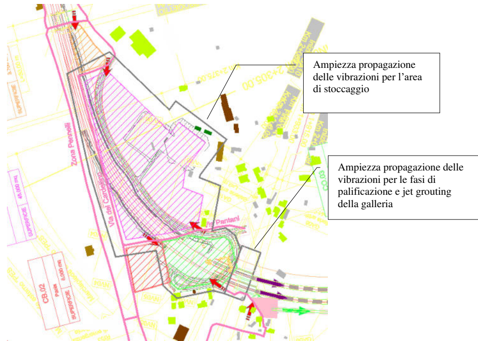
Figura 6-43- stralcio con ampiezza dell'aree di superamento interno agli edifici del limite delle vibrazioni per le aree GA01-CO.03-AS.04
