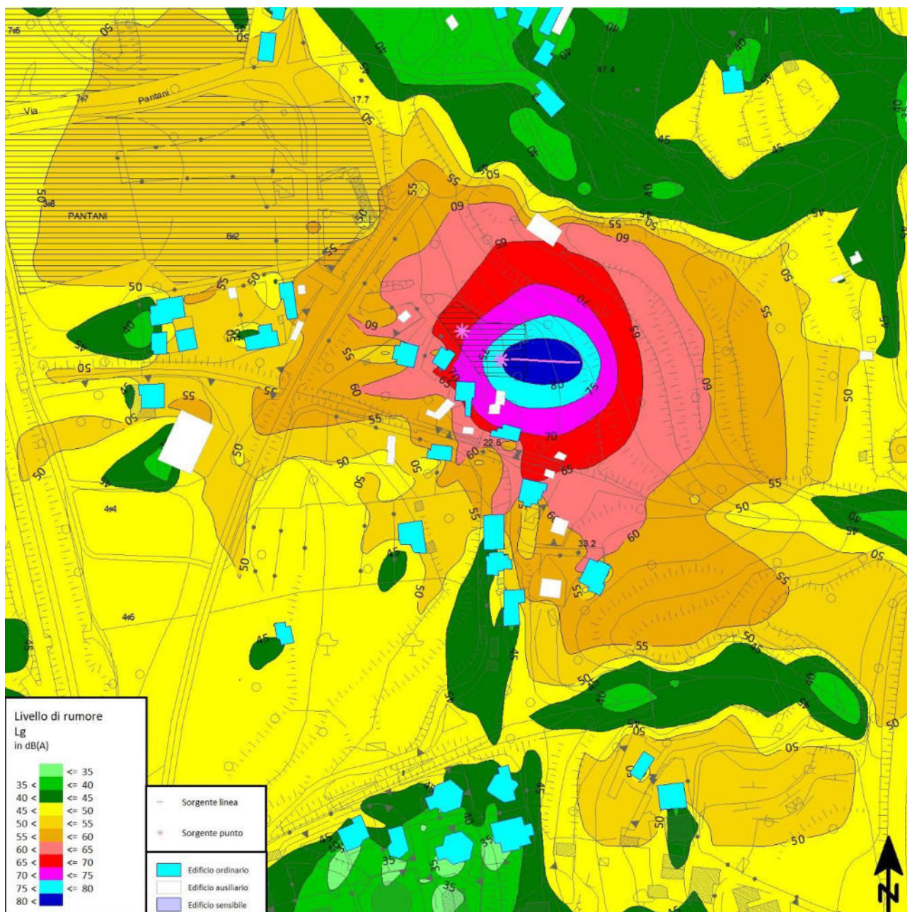
Figura 6-11 – Mappatura acustica, h=4 metri, in assenza di elementi mitigativi
