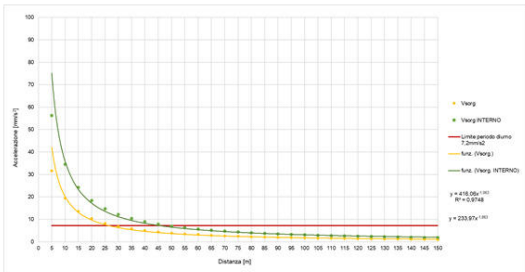
Figura 6-37– Propagazione dei livelli di accelerazione stimati sui ricettori residenziali per il pacchetto “GA (fase di palificazione)”
