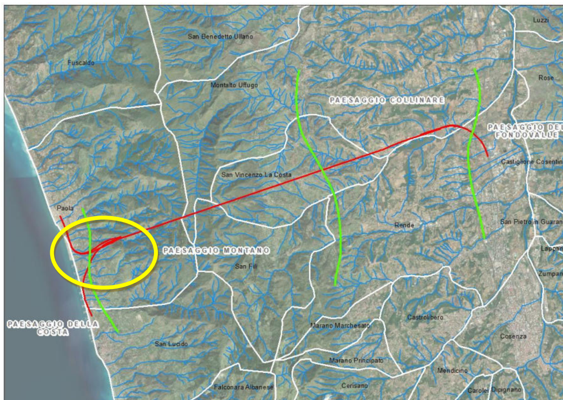
Figura 7-4. Definizione delle Unità del cunicolo disconnessione fumi
