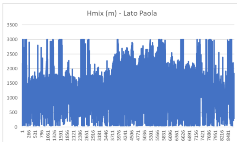
Figura 6-64 Altezza media di mescolamento per l'anno 2019 calcolata da CALMET estratta in prossimità del tracciato di progetto
