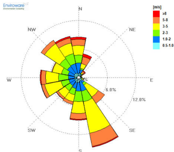
Figura 6-53 Rosa dei venti per l'anno 2019 dati modello WRF LaMMA
