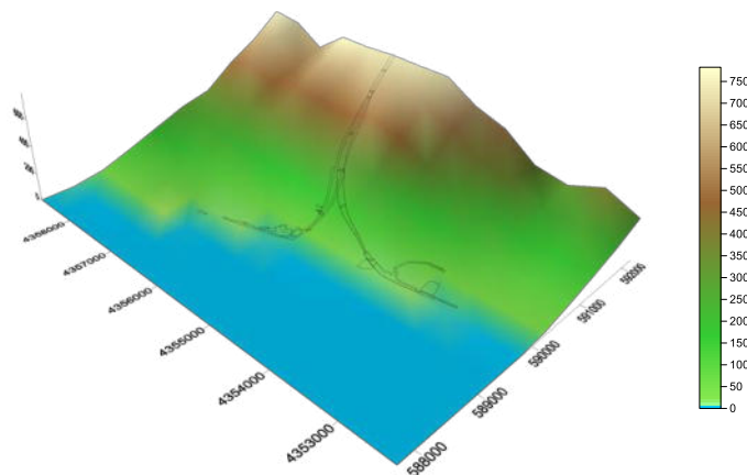
Figura 6-60 orografia area di studio (mslm)
