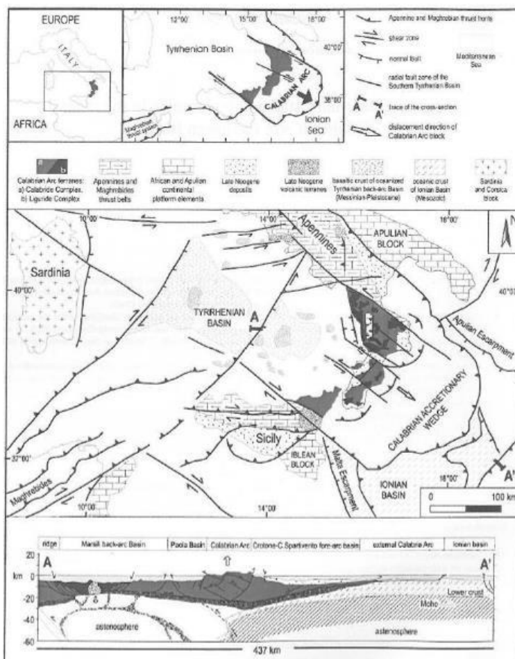
Figura 5-2 Schema geologico-strutturale semplificato del Mediterraneo centrale e dell'Arco Calabro-Peloritano (da Tansi et al. 2007)
