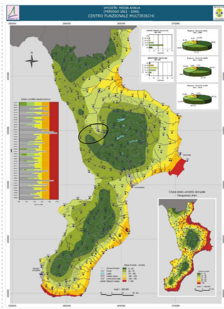
Figura 6-49 umidità relativa media annua 1921-2000 in Calabria (fonte ARPACAL)
