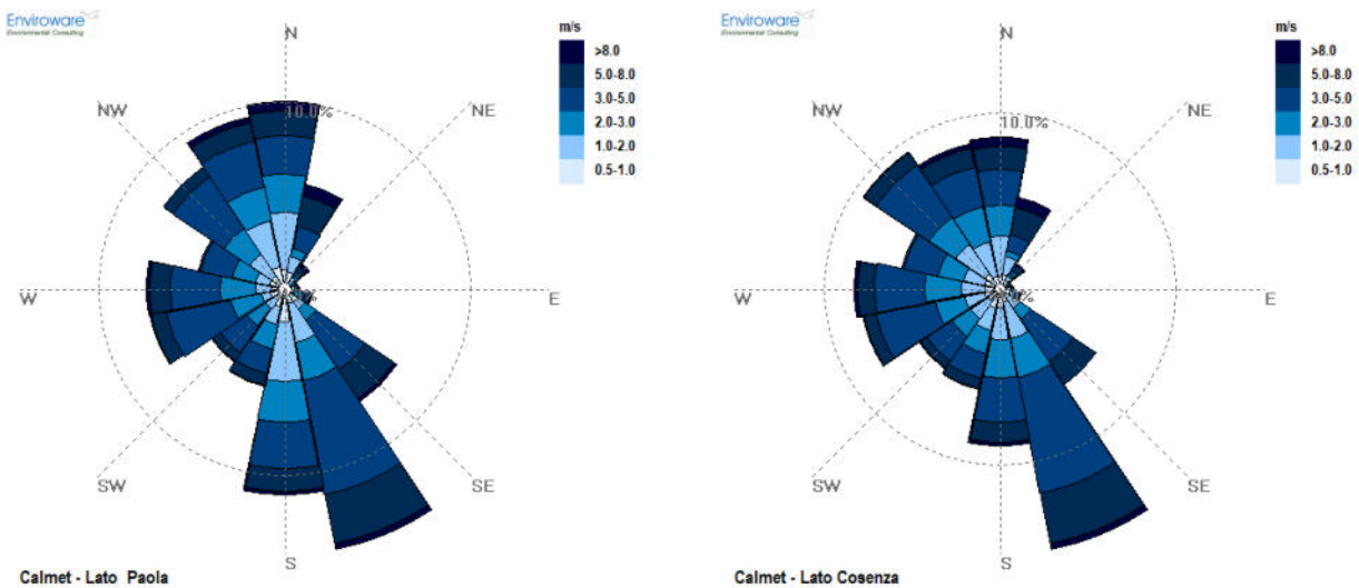
Figura 6-63 rosa dei venti per l'anno 2019 calcolata da CALMET estratta in prossimità del tracciato di progetto nel lato Paola e lato Cosenza
