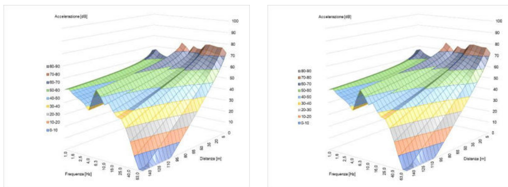
Figura 6-31– Propagazione dei livelli di accelerazione in dB (UNI 9614) per singola frequenza, a sinistra per il pacchetto Cantiere Nuova Viabilità, a destra per il pacchetto Cantiere Nuova Viabilità (utilizzo finitrice)
