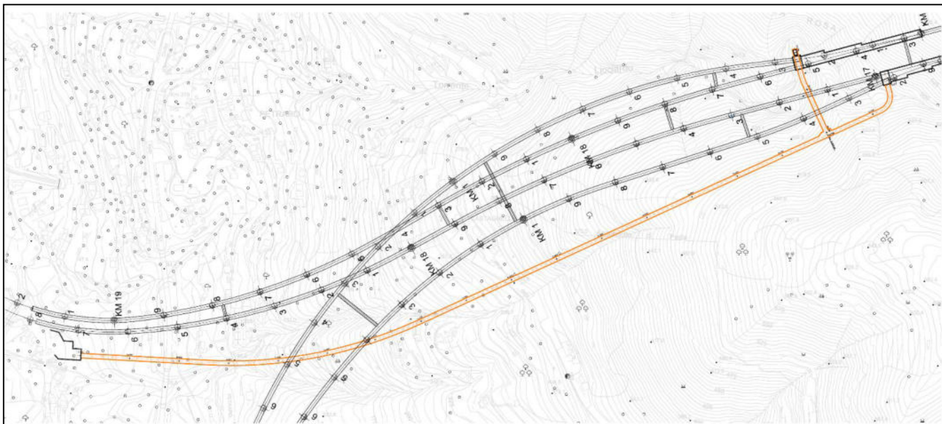
Figura 2-2 Tracciato del cunicolo di disconnessione fumi (in rosso).
