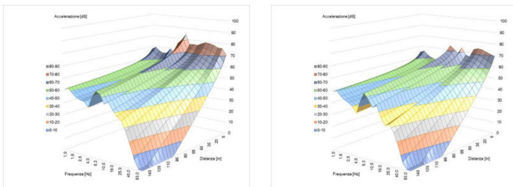
Figura 6-28– Propagazione dei livelli di accelerazione in dB (UNI 9614) per singola frequenza, a sinistra per il pacchetto Realizzazione trincea (fase di jet grouting), a destra per il pacchetto Area Stoccaggio
