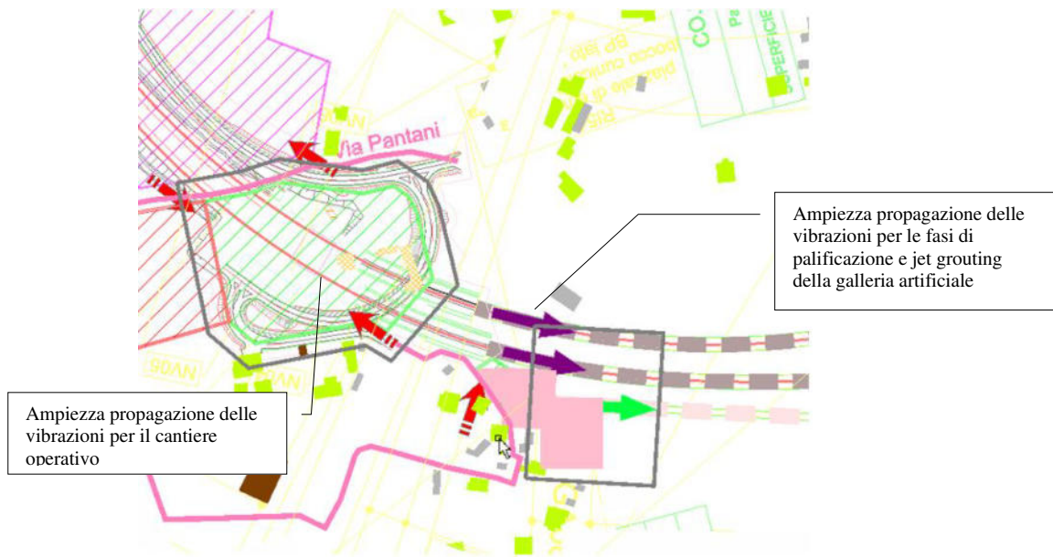
Figura 6-45- stralcio con ampiezza dell'area di superamento interno agli edifici del limite delle vibrazioni per le aree GA08 -CO.05
