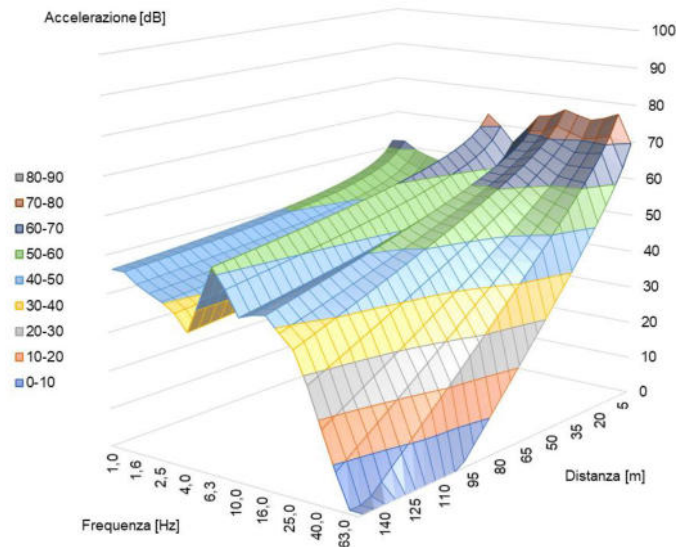
Figura 6-18 Propagazione dello spettro di vibrazione
