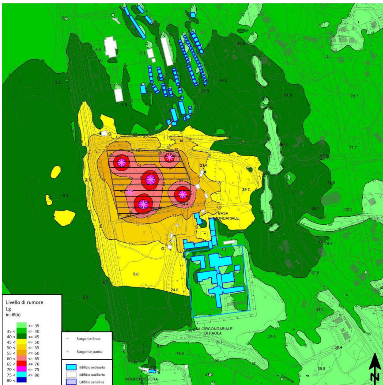
Figura 6-13 – Mappatura acustica, h=4 metri, in assenza di elementi mitigativi
