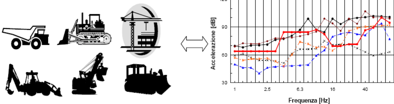
Figura 6-16 relazione tra mezzi d'opera e spettro di emissione di vibrazioni
