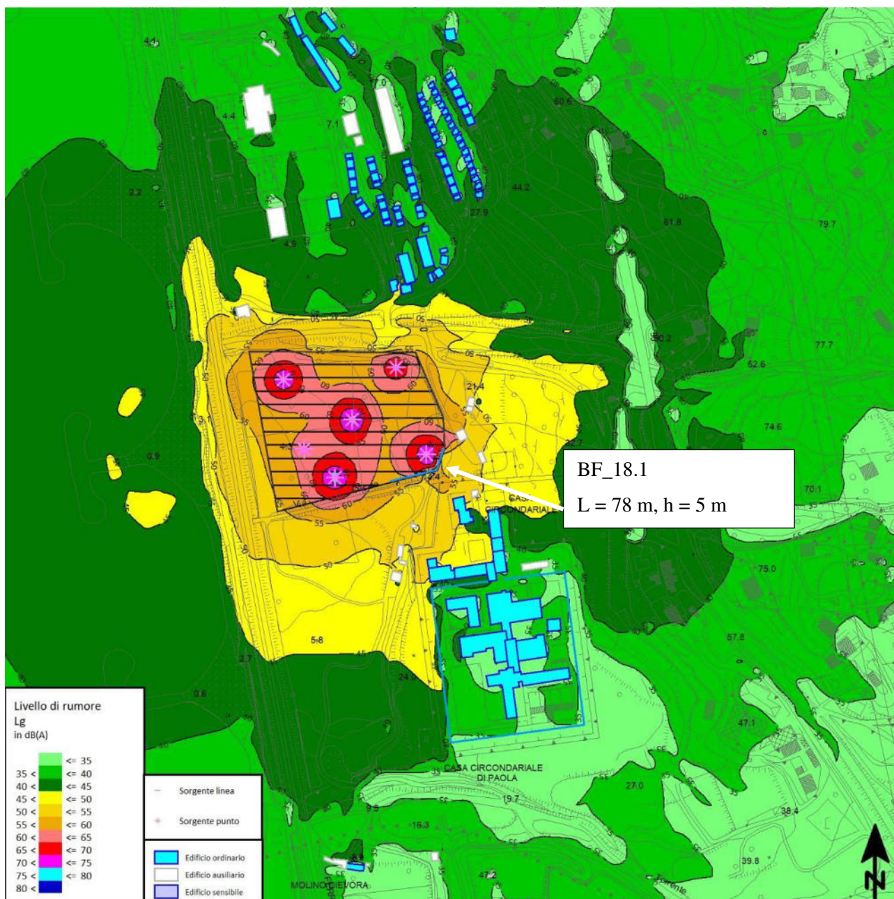
Figura 6-14 – Mappatura acustica, h=4 metri, in presenza di elementi mitigativi
