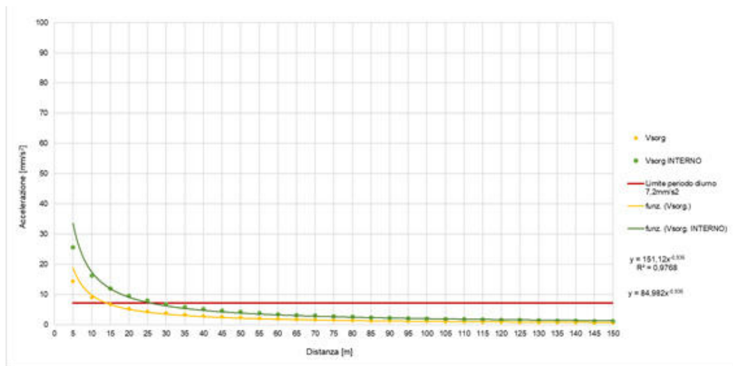
Figura 6-39– Propagazione dei livelli di accelerazione stimati sui ricettori residenziali per il pacchetto “Area Stoccaggio”
