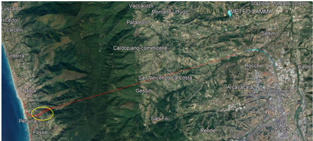
Figura 6-52 – localizzazione estrazione dataset Lamma
