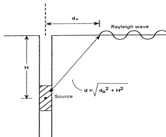
Figura 6-21 Schema della propagazione a partire da una sorgente profonda
