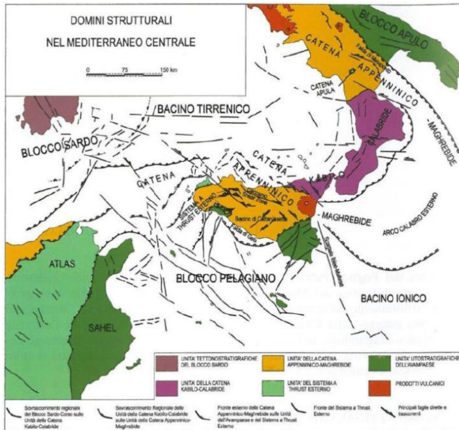
Figura 5-1 Schema dei principali domini strutturali nel Mediterraneo centrale (da Lentini et al. 1995)
