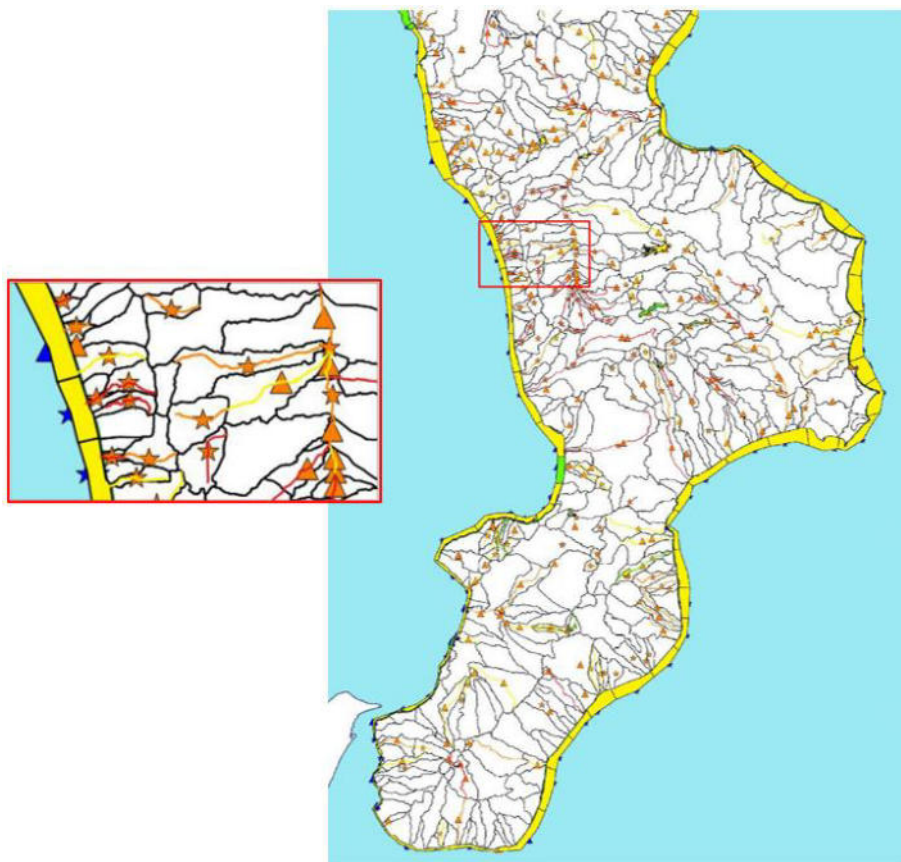
Figura 5-9 Stato ecologico dei corpi idrici superficiali (Stralcio tavola 6.1.1 del Progetto di Piano di Gestione delle Acque Ciclo 2021-2027)
