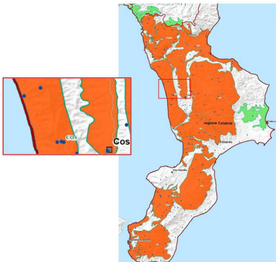
Figura 5-12 Stato quantitativo dei corpi idrici sotterranei (Stralcio tavola 6_2_2 del Progetto di Piano di Gestione delle Acque Ciclo 2021-2027)
