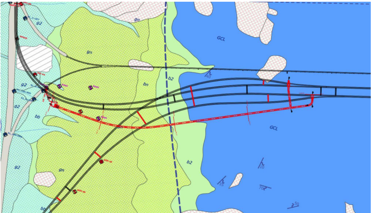
Figura 5-3 – Stralcio carta geologica
