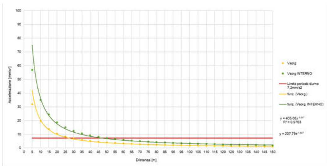
Figura 6-38– Propagazione dei livelli di accelerazione stimati sui ricettori residenziali per il pacchetto “GA (fase di jet grouting)”
