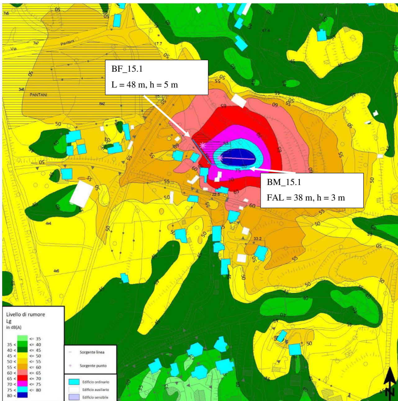
Figura 6-12 – Mappatura acustica, h=4 metri, in presenza di elementi mitigativi
