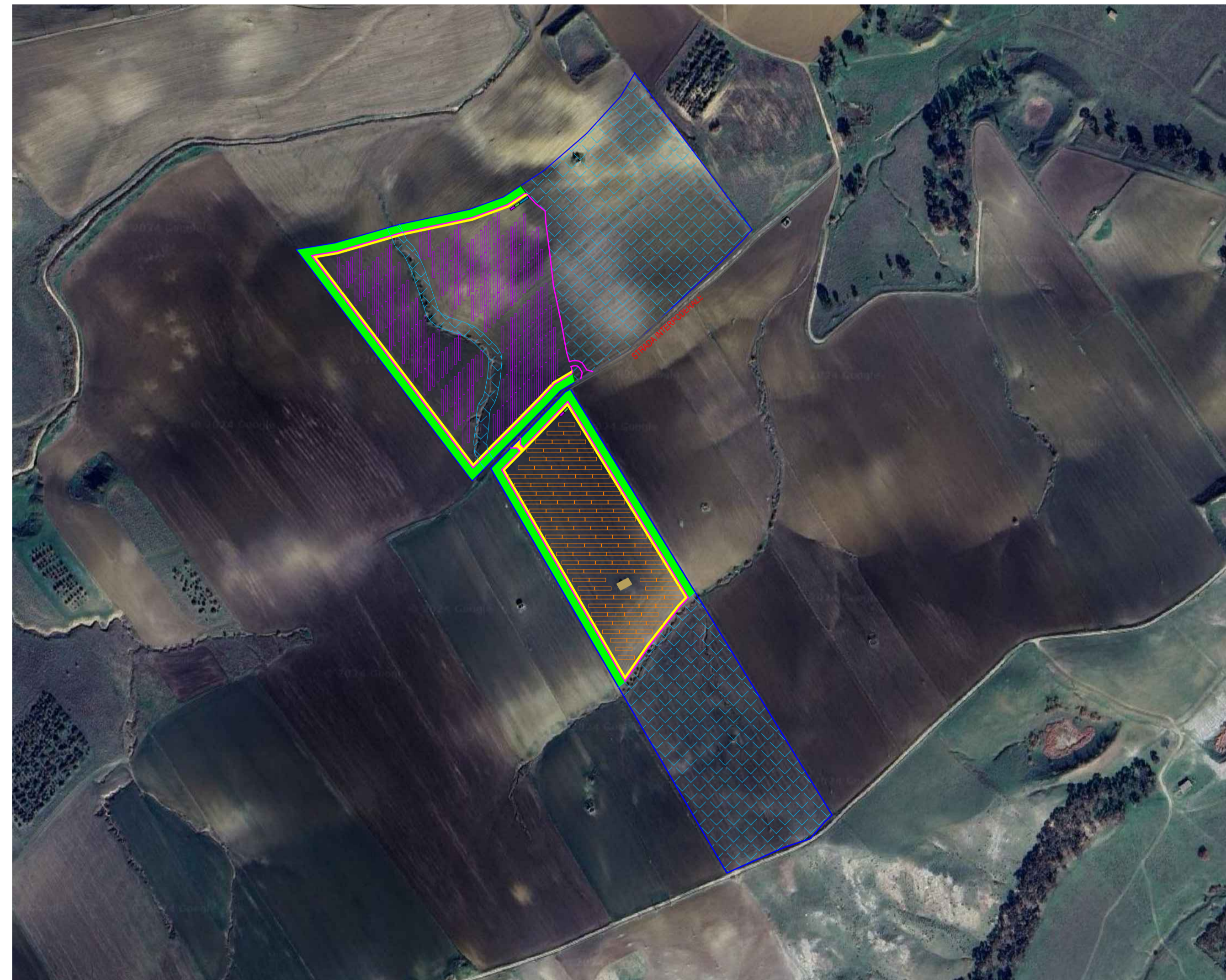
LAYOUT D'IMPIANTO IN FASE DI ESERCIZIO SCALA 1:4.000
