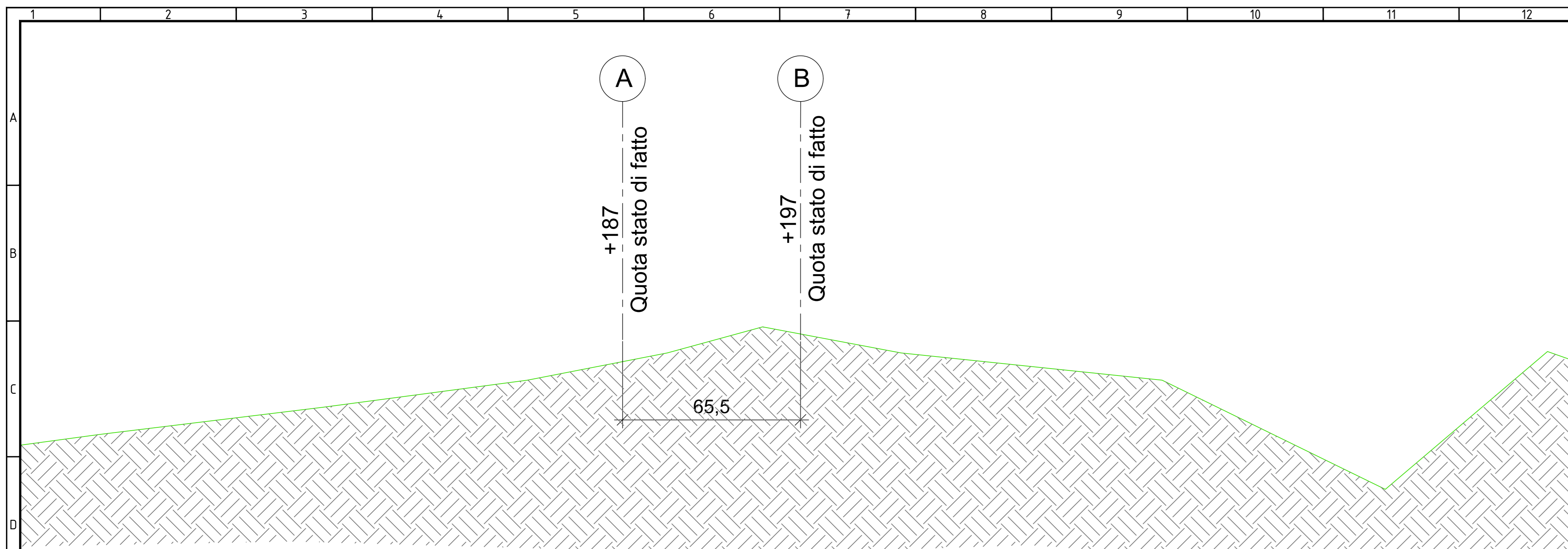
SEZIONE A-A - STATO DI FATTO scala 1:100
