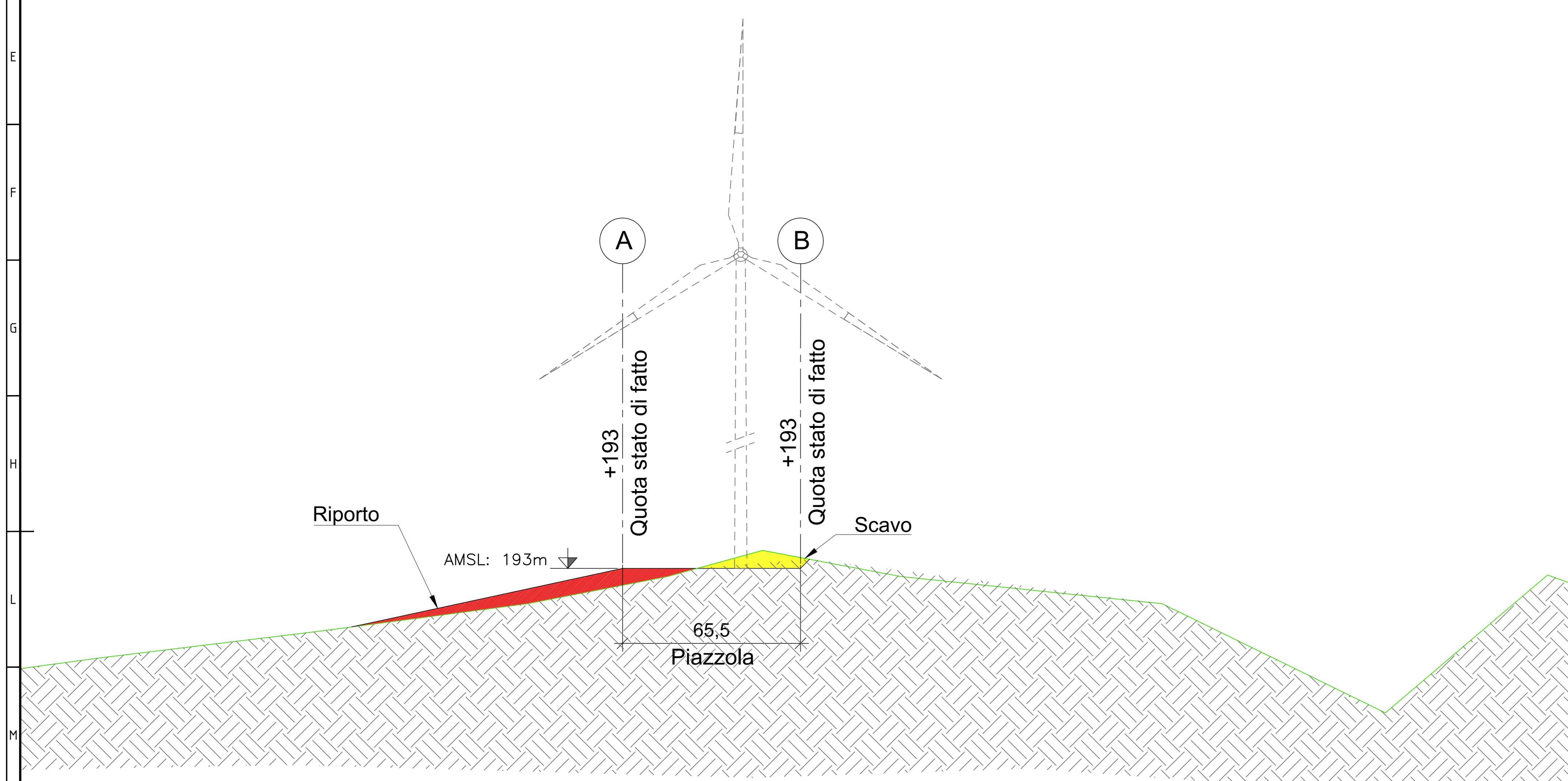
SEZIONE A-A - FASE DI CANTIERE scala 1:100
