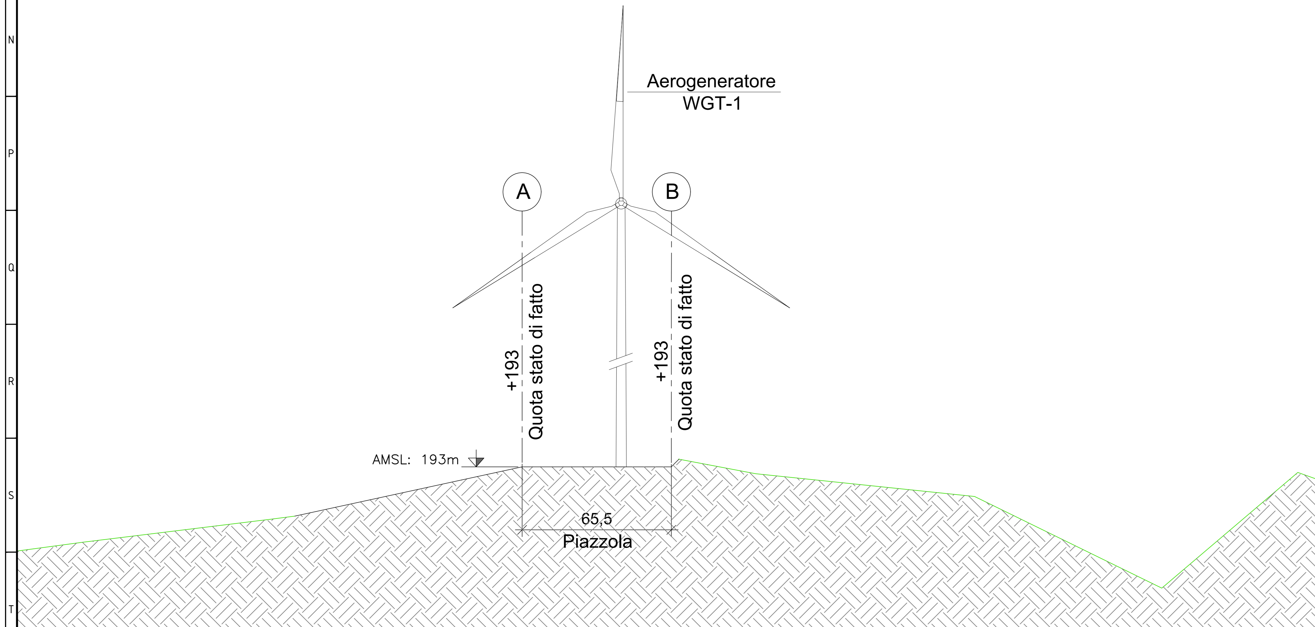
SEZIONE A-A - FASE DI ESERCIZIO scala 1:100
