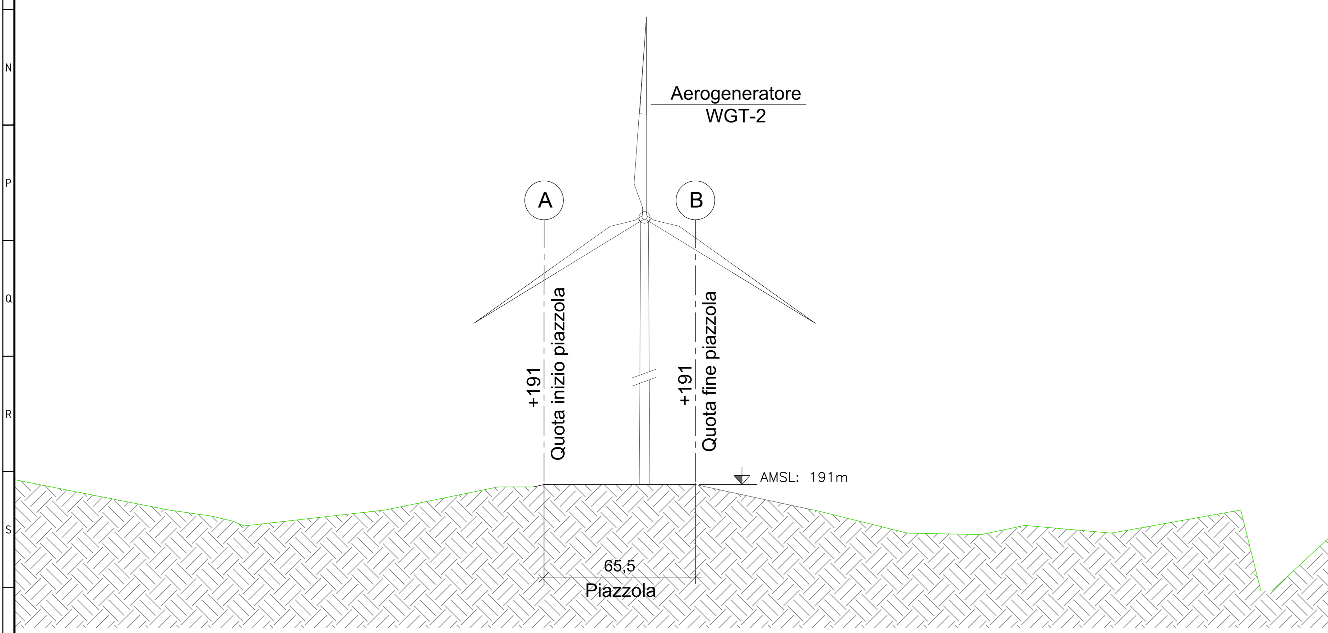
SEZIONE B-B - FASE DI ESERCIZIO scala 1:100
