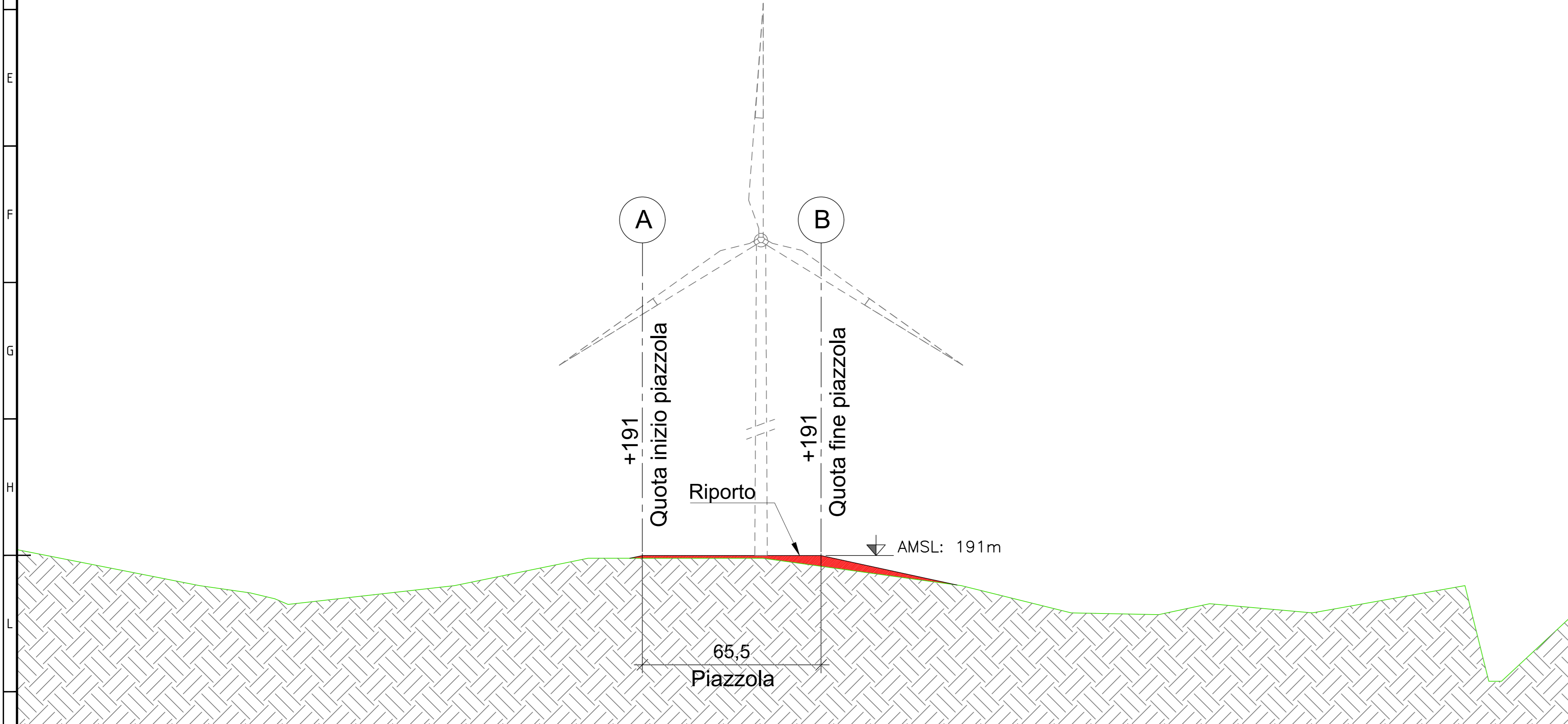
SEZIONE B-B - FASE DI CANTIERE scala 1:100
