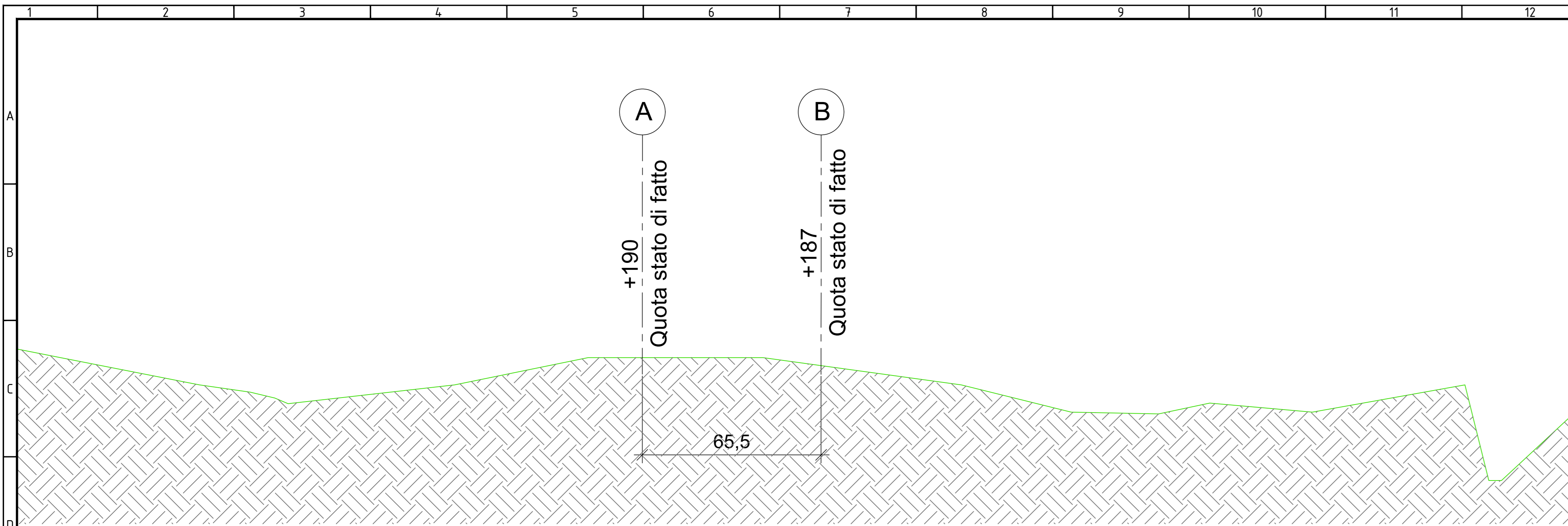
SEZIONE B-B - STATO DI FATTO scala 1:100
