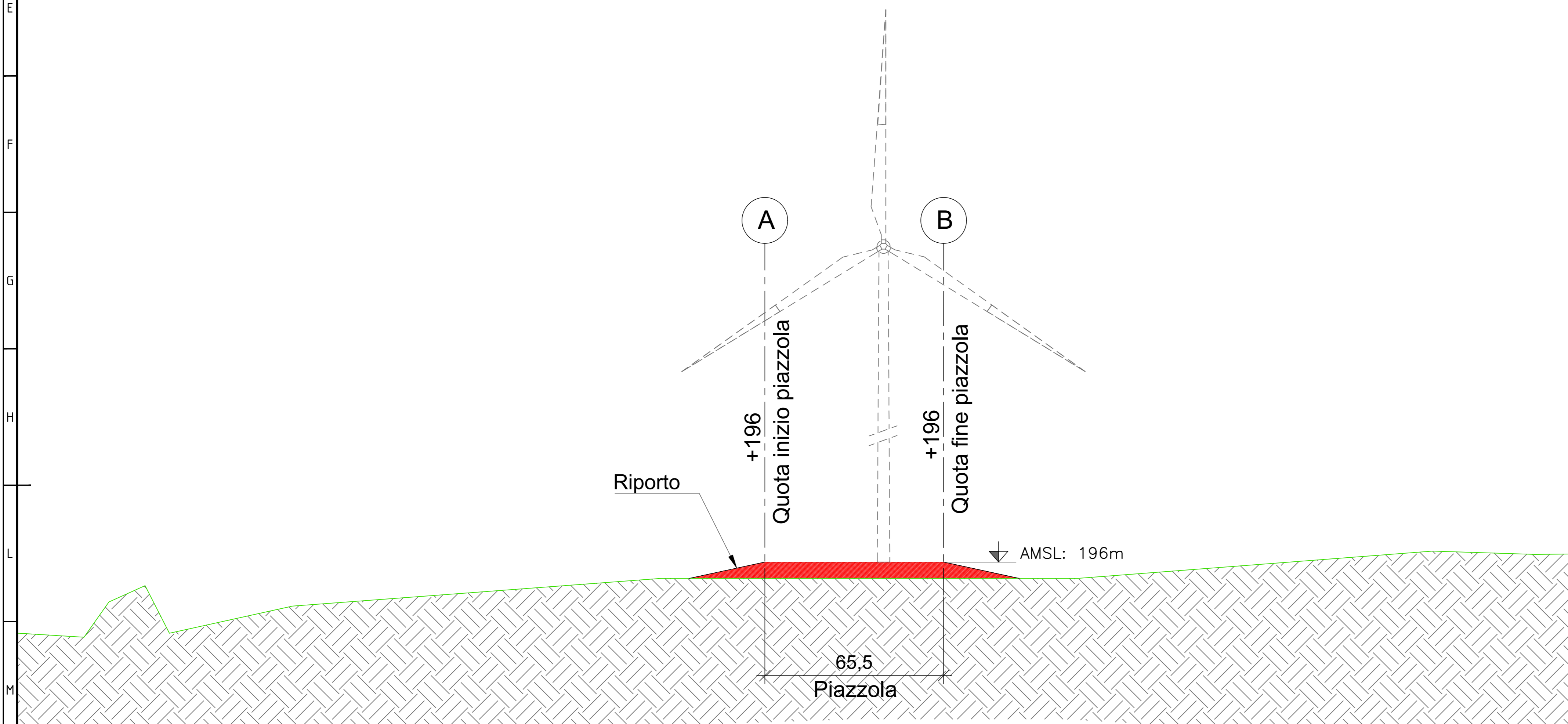
SEZIONE C-C - FASE DI CANTIERE scala 1:100
