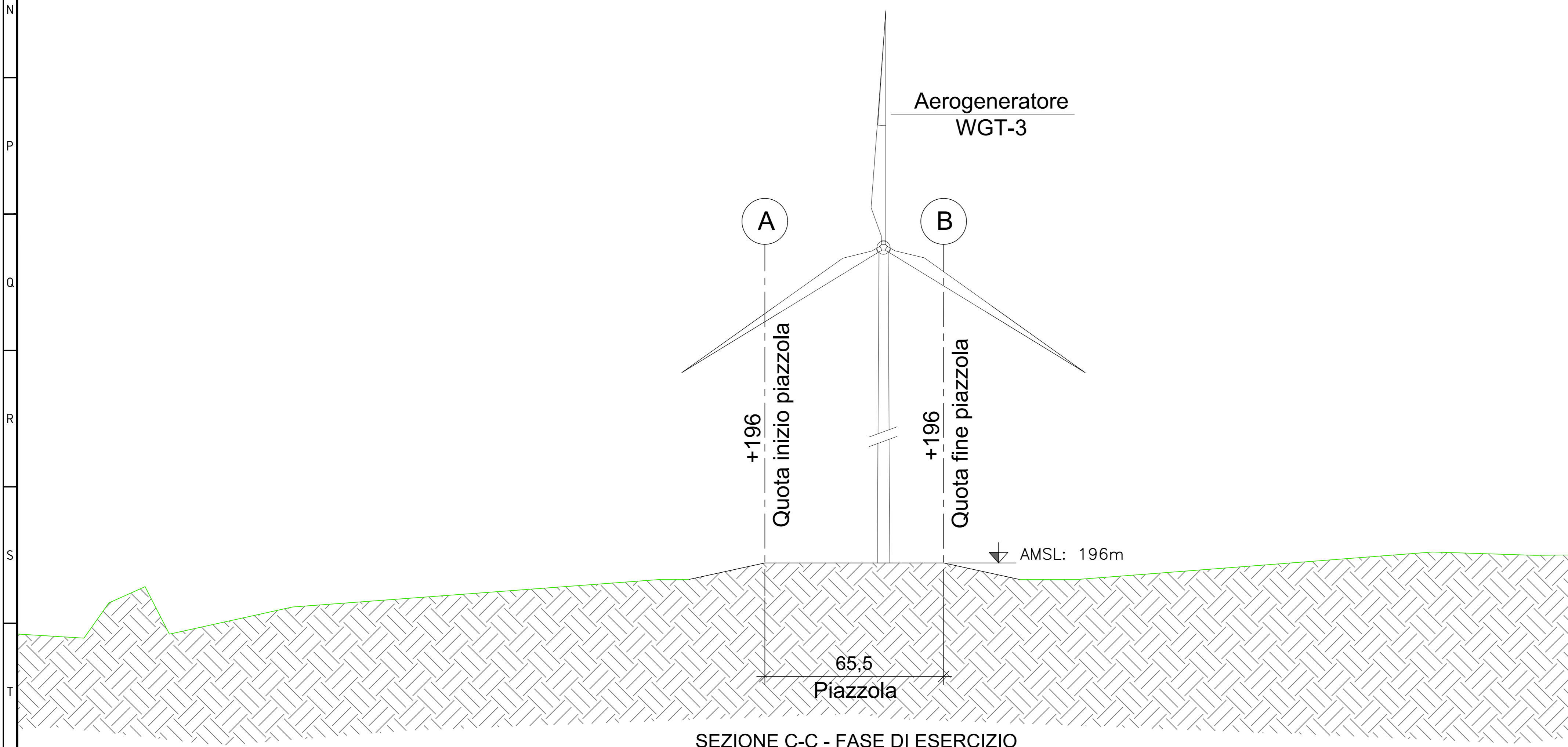
SEZIONE C-C - FASE DI ESERCIZIO scala 1:100
