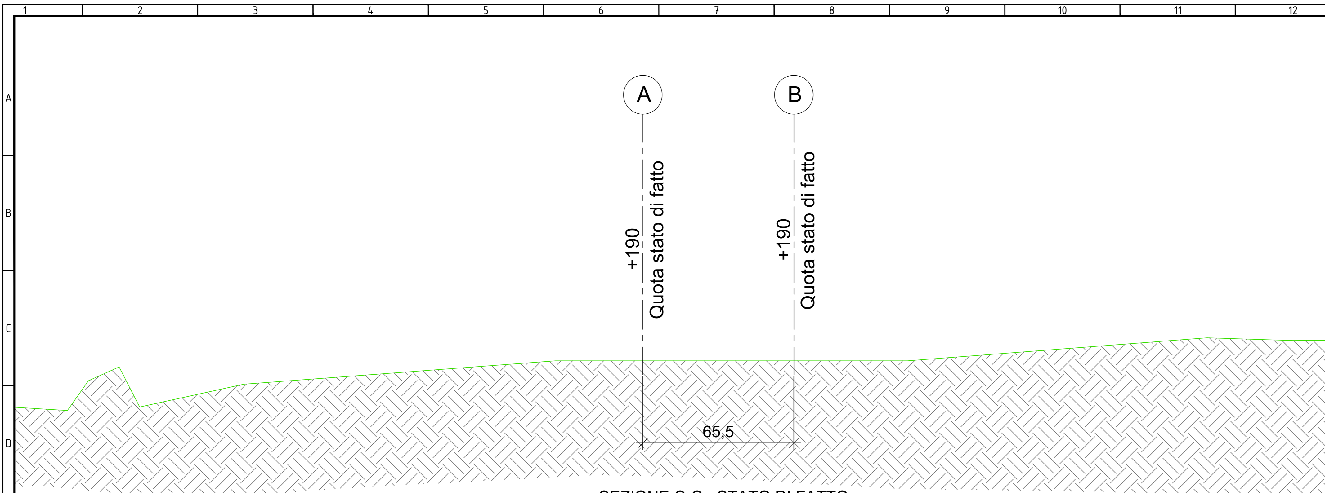
SEZIONE C-C - STATO DI FATTO scala 1:100
