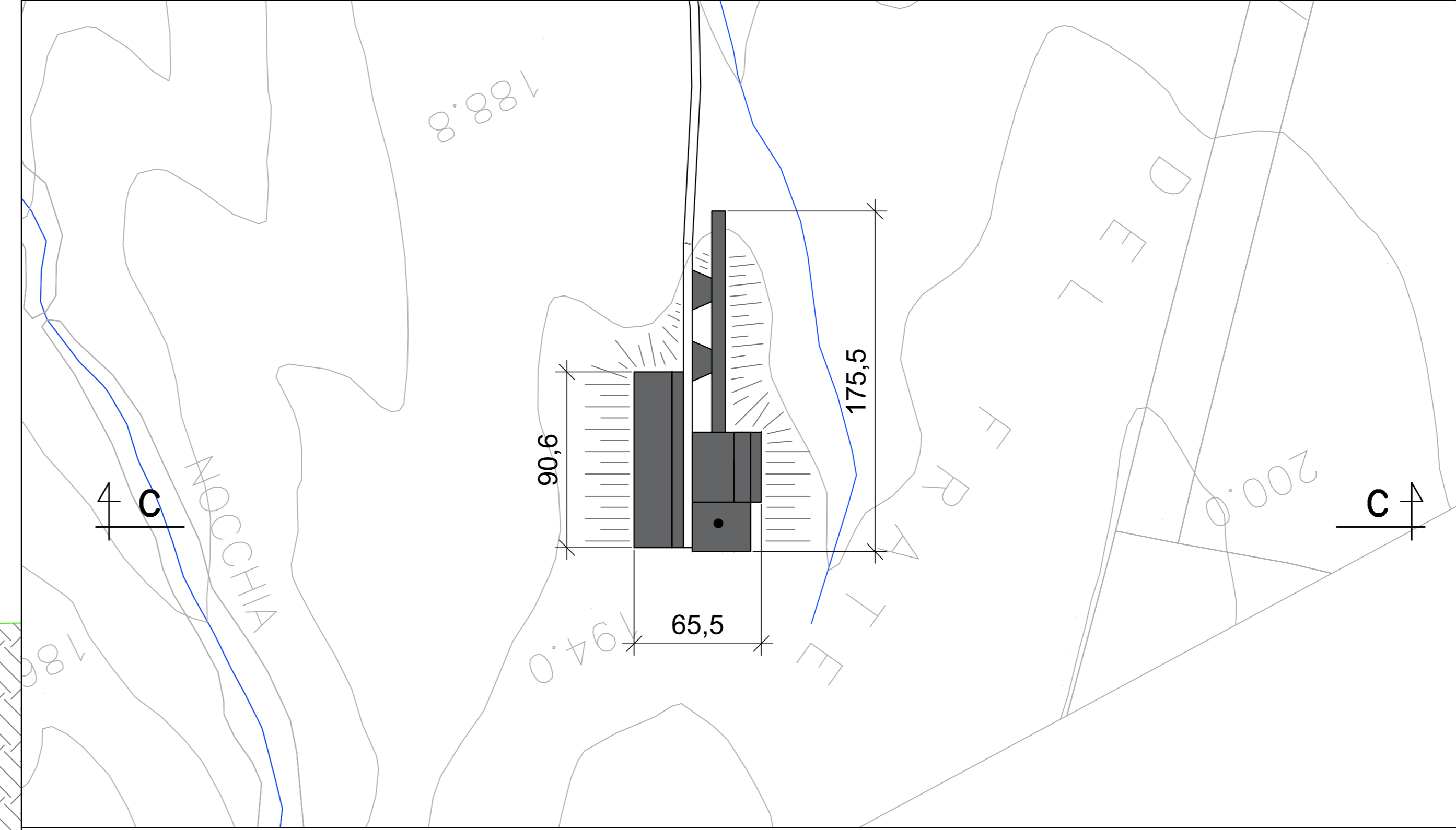
VISTA IN PIANTA PIAZZOLA WGT-3 scala 1:200
