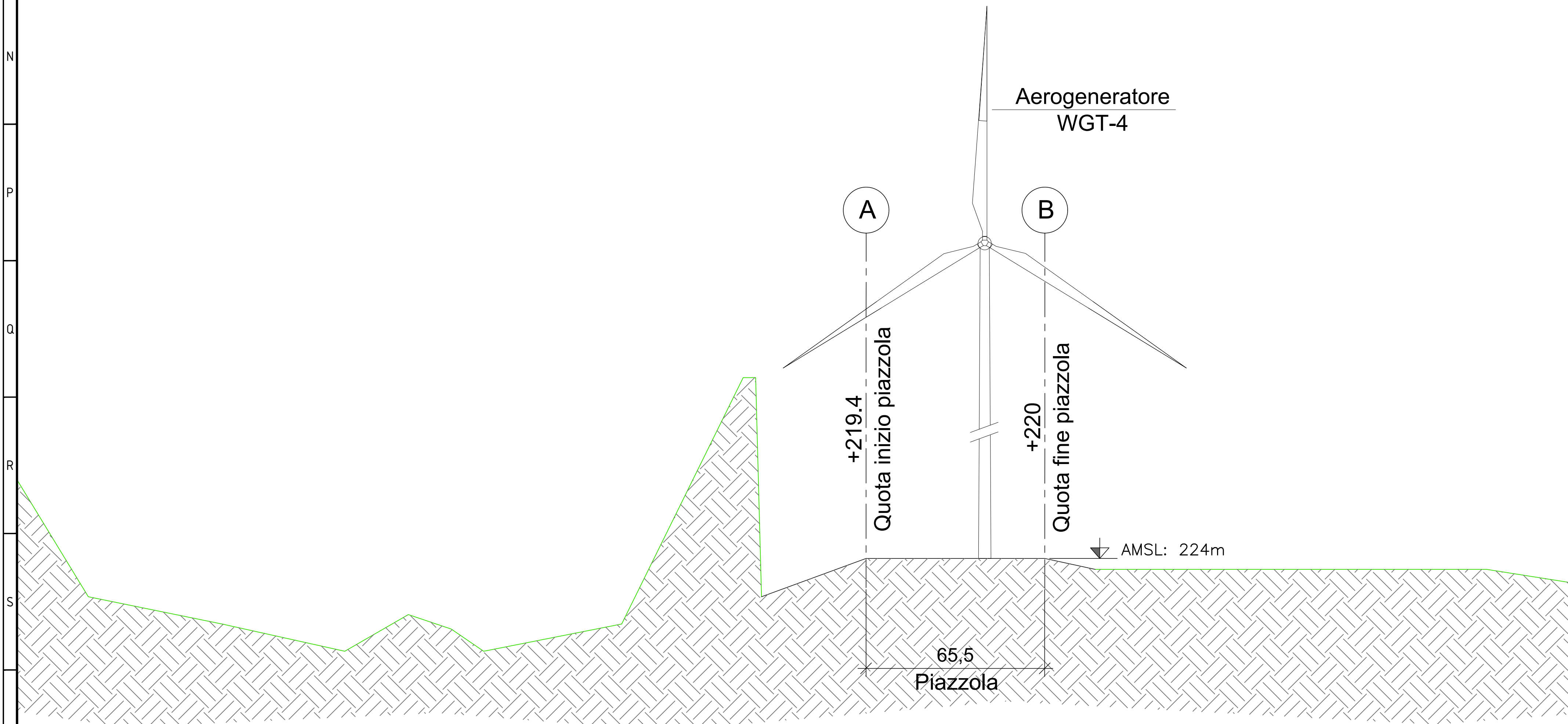
SEZIONE D-D - FASE DI ESERCIZIO scala 1:100
