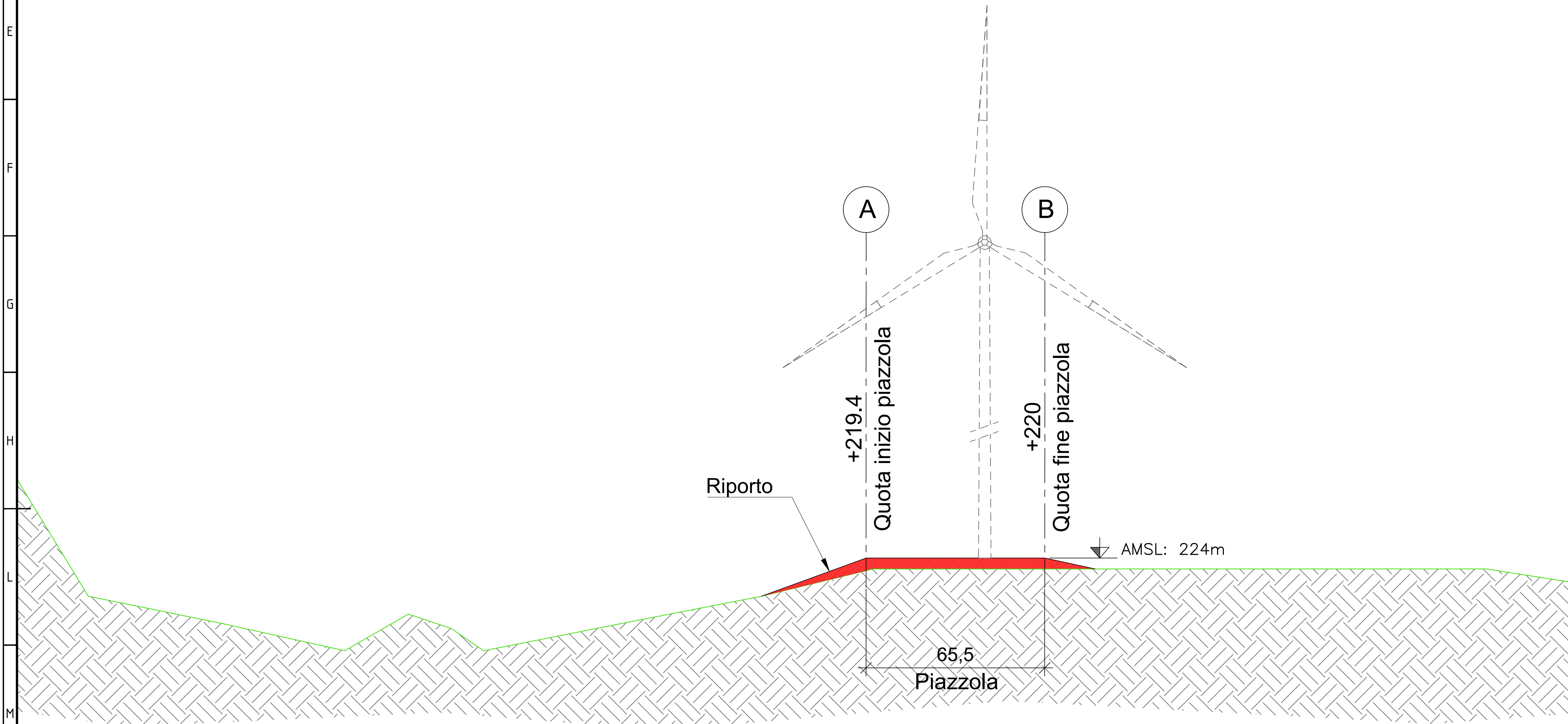
SEZIONE D-D - FASE DI CANTIERE scala 1:100
