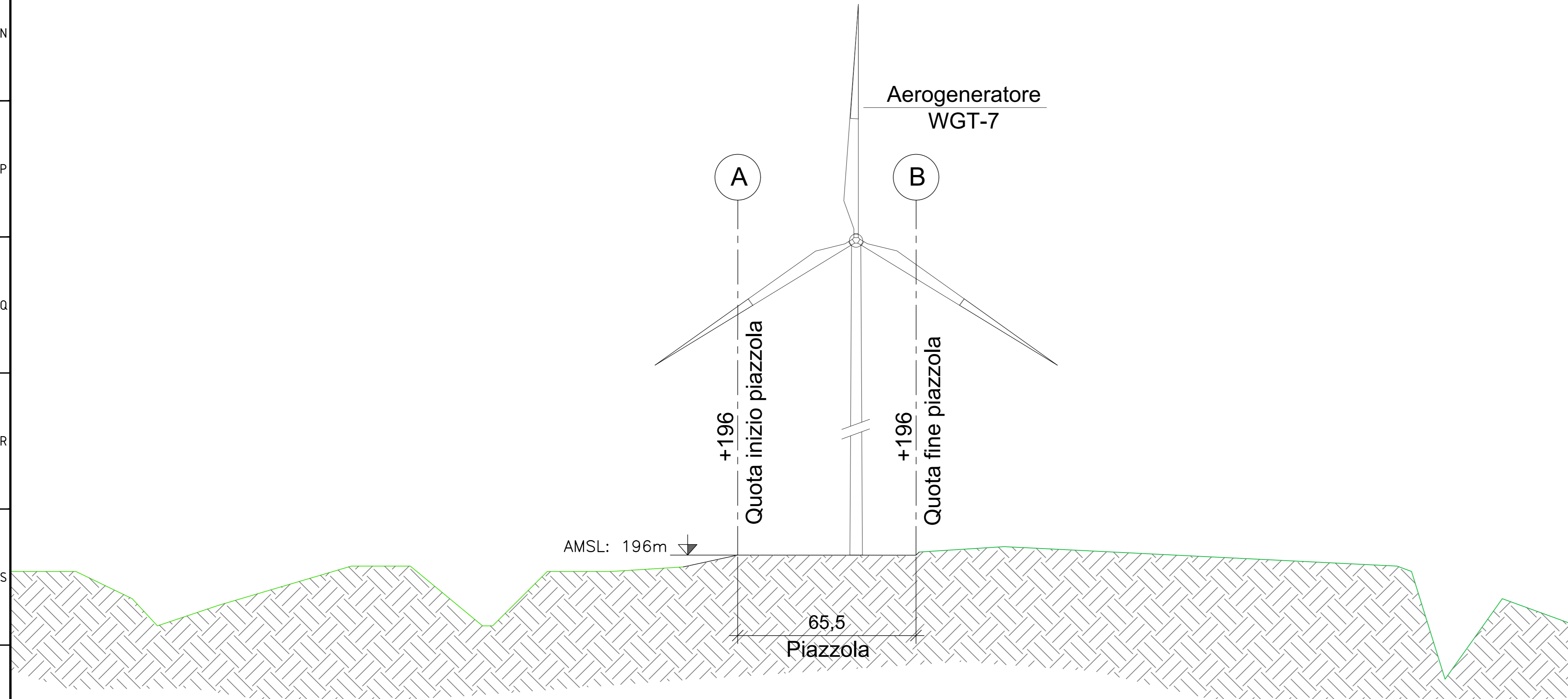
SEZIONE G-G - FASE DI ESERCIZIO scala 1:100
