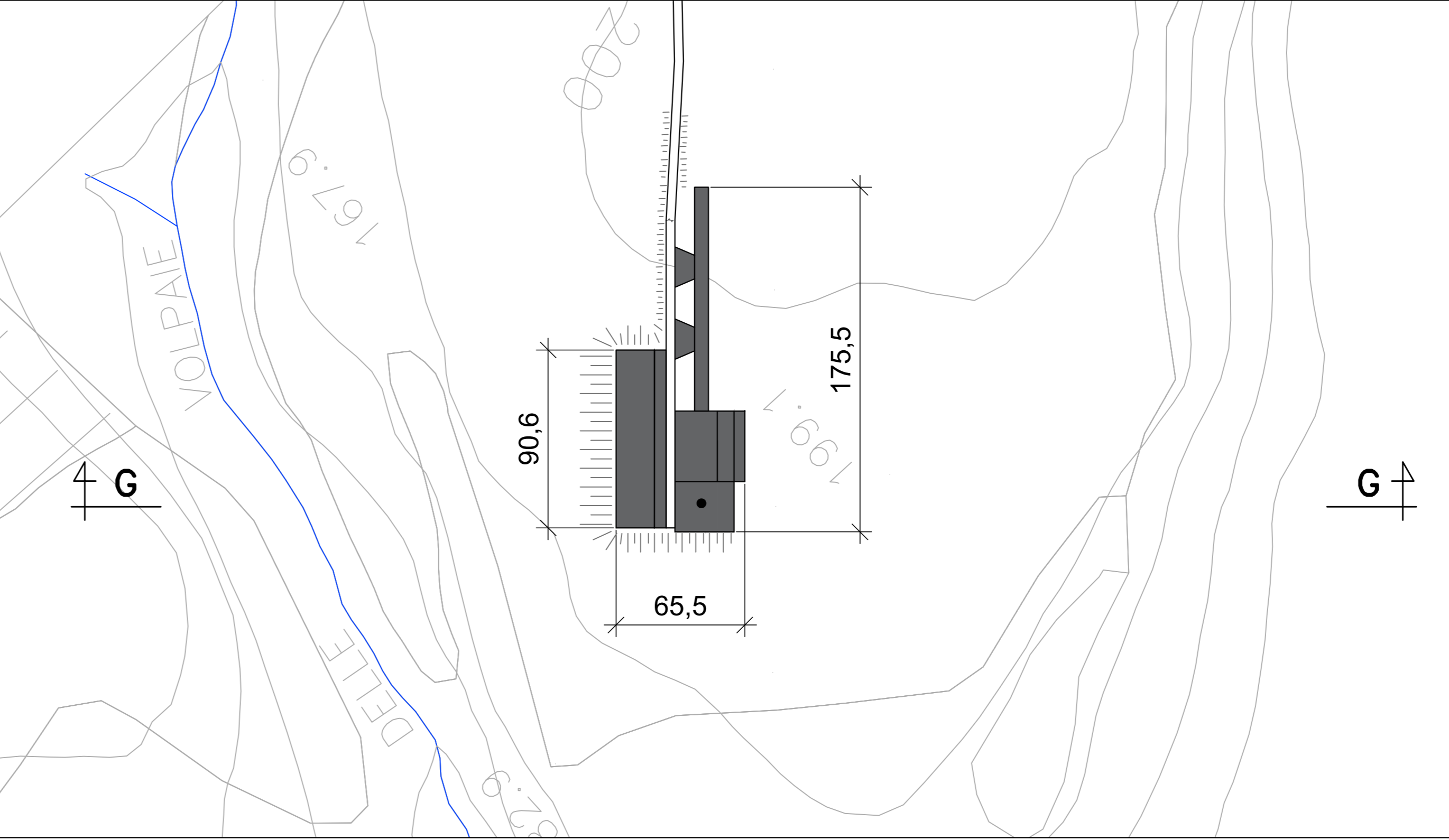
VISTA IN PIANTA PIAZZOLA WGT-7 scala 1:200
