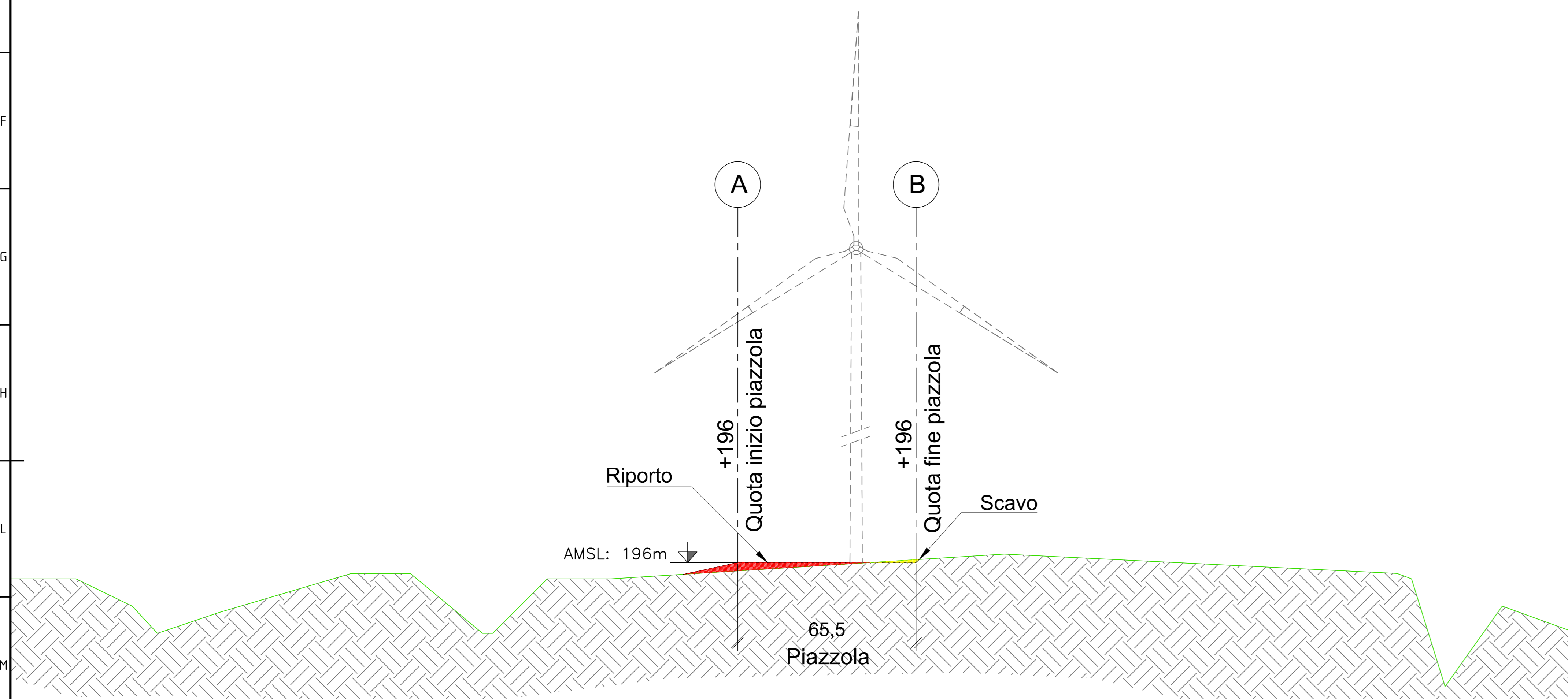
SEZIONE G-G - FASE DI CANTIERE scala 1:100
