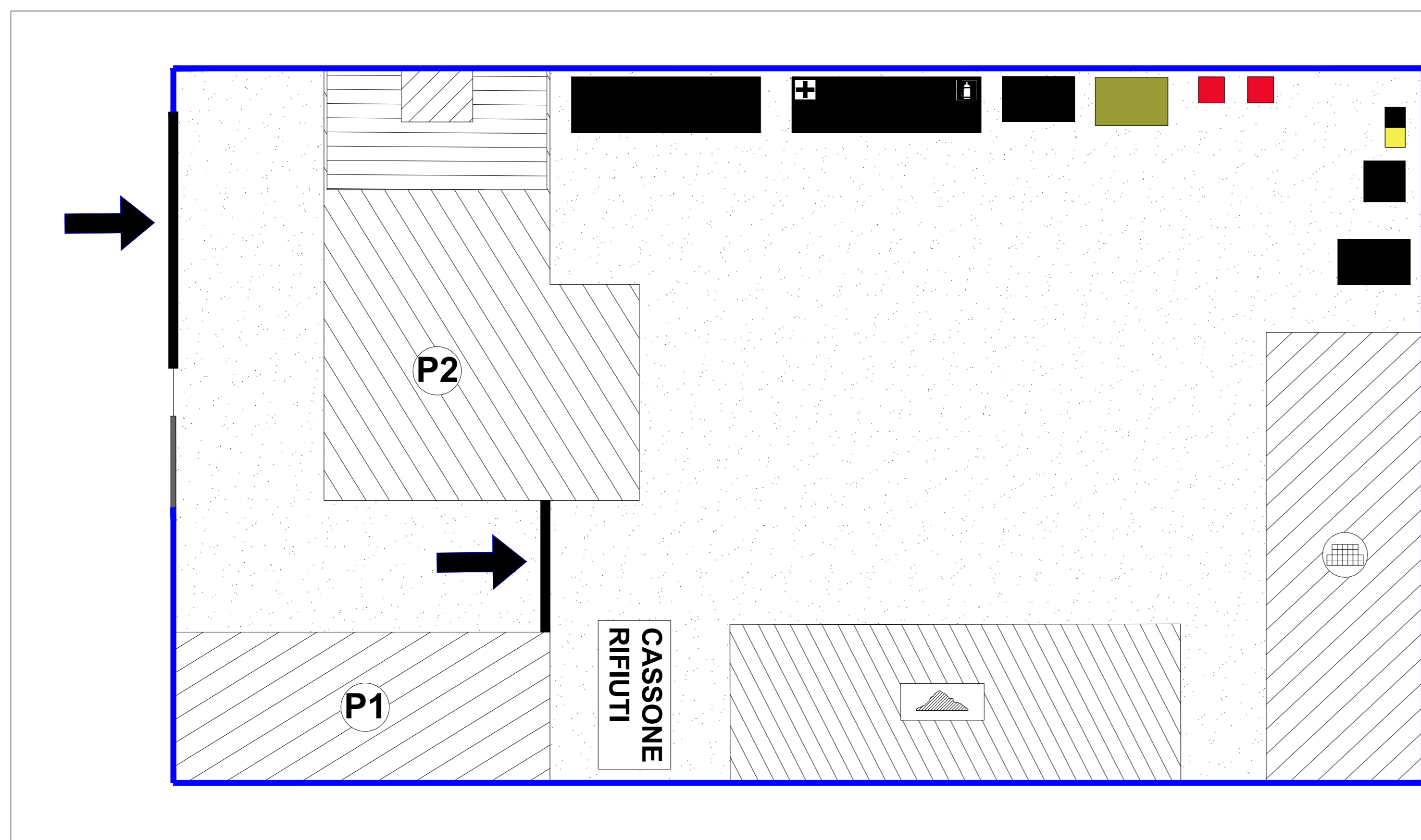
TIPOLOGICO AREA DI CANTIERE 2 Scala 1:200
